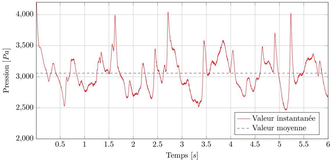
FIGURE IV.1 – Oscillations de la pression dynamique du fluide (air) sur la face d'entrée du réacteur pour U_{in} = 2U_{mf} . Propriétés du système données dans le tableau IV.1
