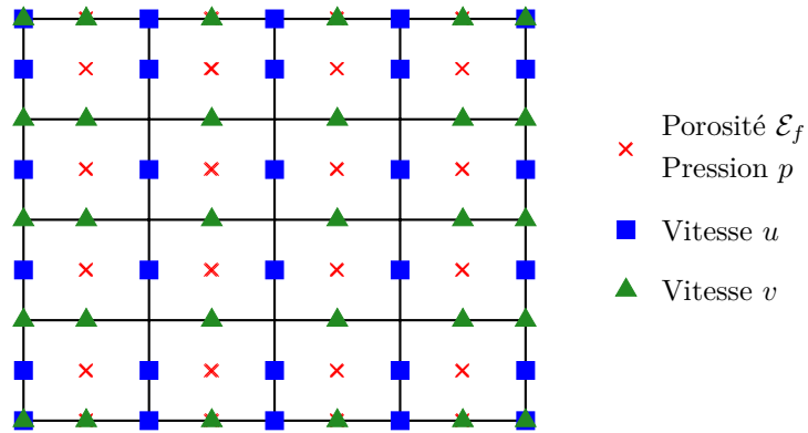
FIGURE III.4 – Positions des variables sur la grille décalée en 2D
