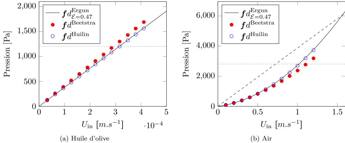
FIGURE IV.3 – Evolution du saut de pression à travers le lit en fonction de la vitesse d'entrée du fluide. Les paramètres de simulation \mathcal{E} sont présentés dans les tableaux IV.1-(a) et (b)
