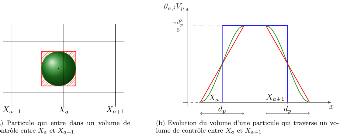
FIGURE II.12 – Variation de la prise en compte du volume d'une particule dans un volume de contrôle. En bleu, méthode du centre de gravité, en vert variation exacte, en rouge la méthode du cube englobant
