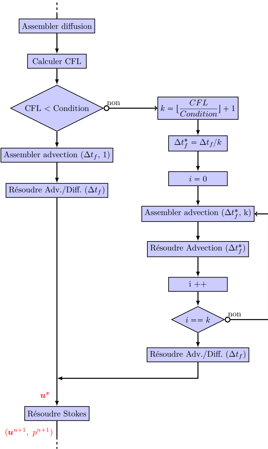
FIGURE 16 – Détail du calcul des champs u_f et p
