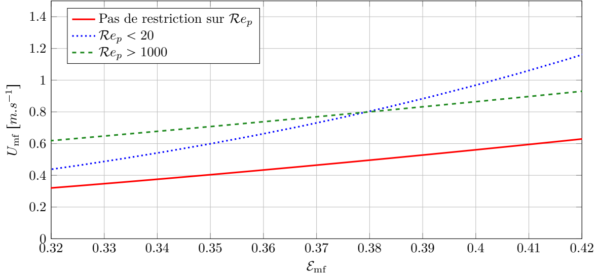
FIGURE I.8 – Vitesse minimale de fluidisation en fonction de la porosité au minimum de fluidisation pour des particules de diamètre d_p = 1\text{mm} de densité \rho_p = 2500\text{ kg.m}^{-3} fluidisées par de l’air \rho_f = 1.2\text{ kg.m}^{-3} . Equation (I.29) en rouge, équation (I.30) en bleu et équation (I.33) en vert
