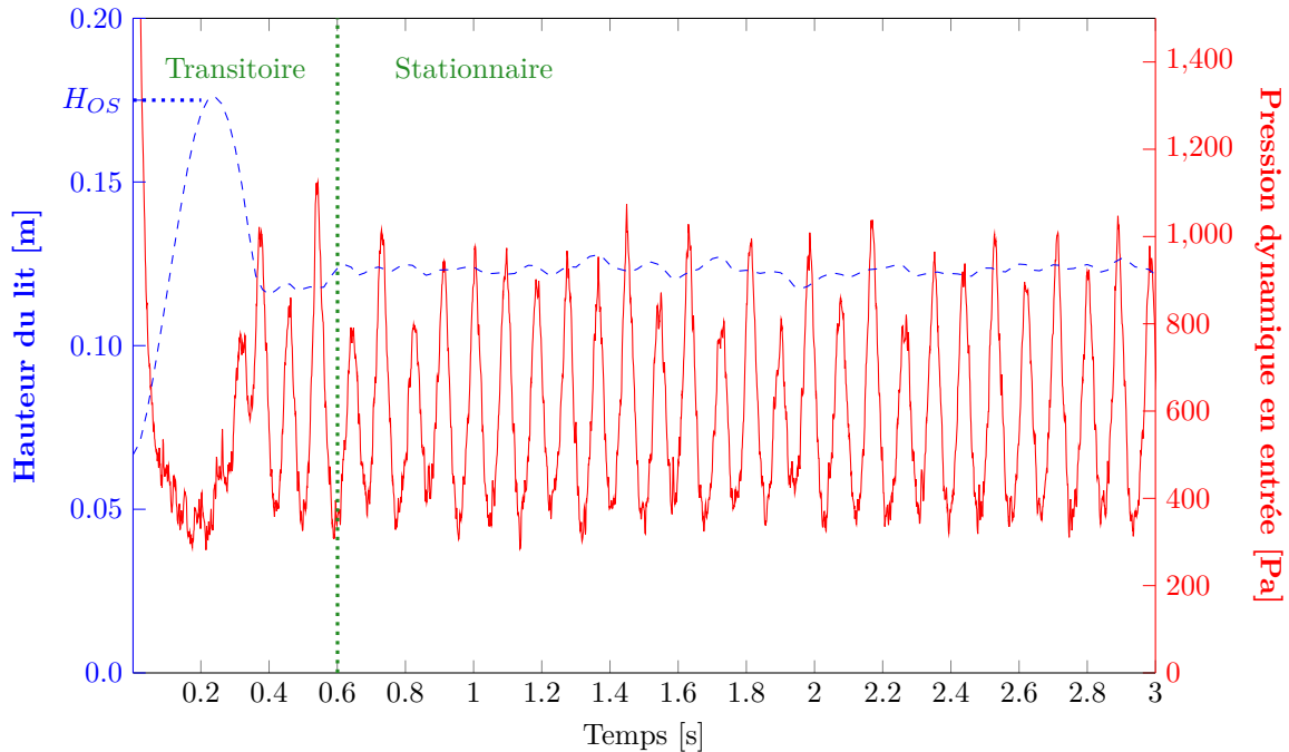
FIGURE IV.11 – Exemple d'évolution temporelle de la hauteur (en bleu) et de la pression en entrée (en rouge) dans un lit pulsé mono-jet pour une vitesse d'injection U_{\text{bulk}} = 3U_{\text{in}}
