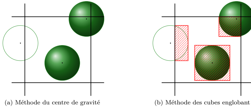
FIGURE II.11 – Illustration de la méthode des cubes englobants
