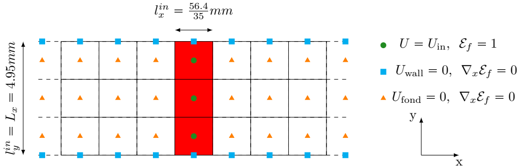
FIGURE IV.10 – Conditions aux limites discrétisées sur la face inférieure d'un lit pulsé
