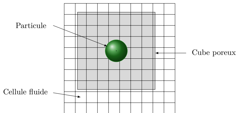
FIGURE II.13 – Méthode du cube poreux proposée par Link [138]
