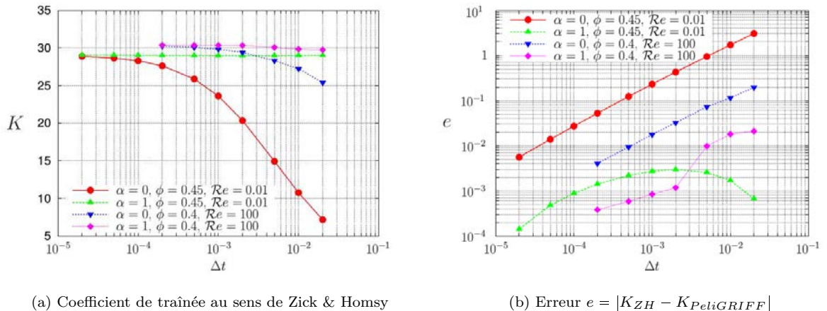
FIGURE VI.1 – Convergence temporelle pour un écoulement à travers un assemblage cubique simple de sphère en fonction du régime d'écoulement et du type de forçage
