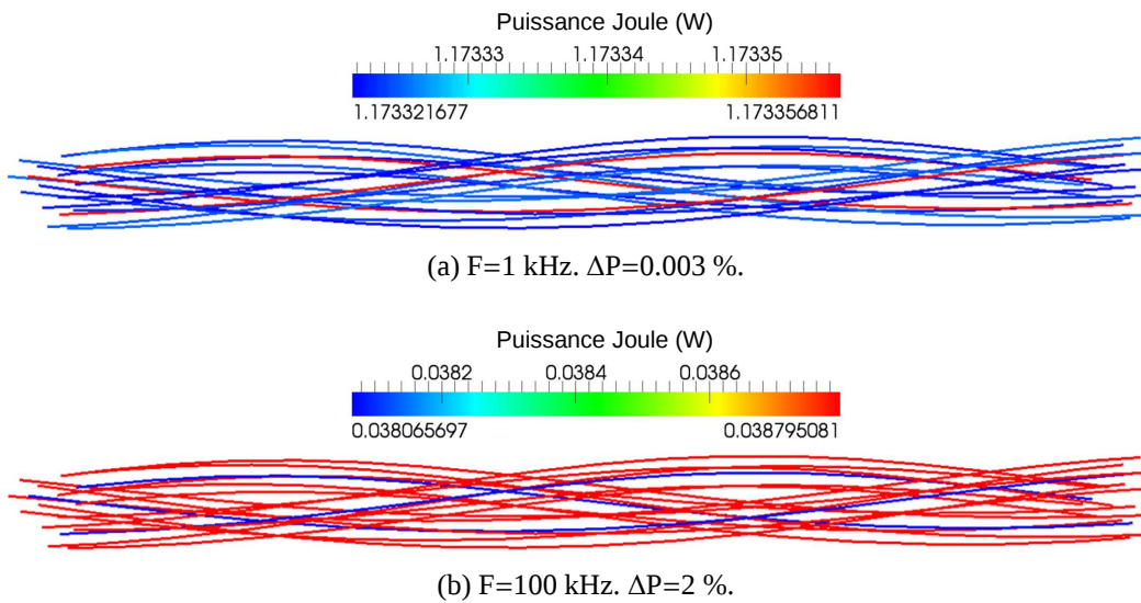
FIGURE 4.4 – Répartition de la puissance Joule entre les brins de l'inducteur 3x6 à 1 kHz et à 100 kHz (modèle filiforme).
