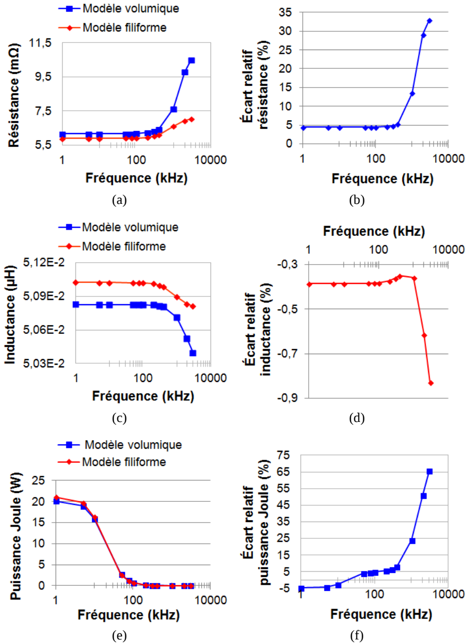
FIGURE 4.2 – Évolution des valeurs et des écarts calculés par le modèle filiforme par rapport au modèle volumique et en fonction de la fréquence, pour la résistance, l'inductance et la puissance Joule de l'inducteur 3×6.
