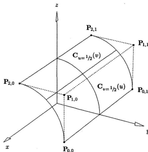
Figure 2.20 – Un exemple de surface de Bézier. Un patch d'une surface cylindrique générée par une surface rationnelle de Bézier [PT97].
