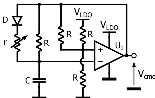
FIGURE 4.46 – Schéma électrique du circuit oscillateur astable
