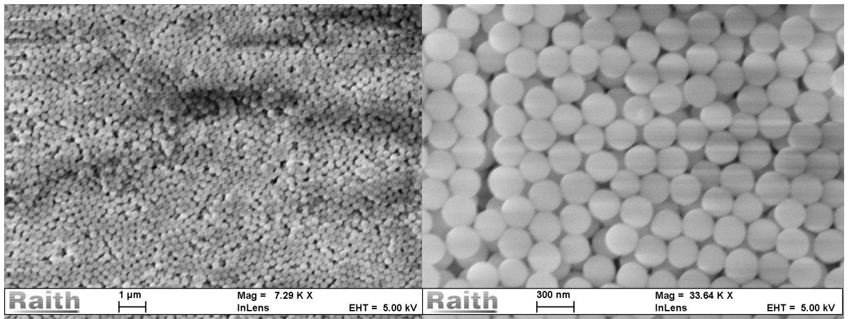
Figure 2-8: Imagerie par microscope électronique à balayage d'une opale de 20 couches de billes en \text{SiO}_2 de diamètre 250 nm. On observe des lacunes et des agrégats de billes. La dernière couche ne présente pas d'organisation hexagonale.
