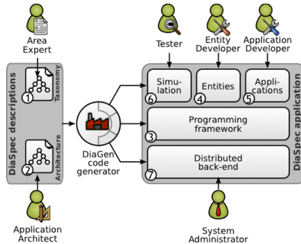
FIGURE 3: DiaSuite : Vue globale
