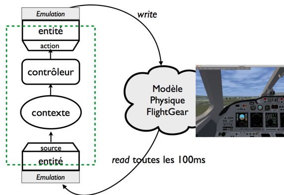
FIGURE 11: Test de l'application : Environnement FlightGear
