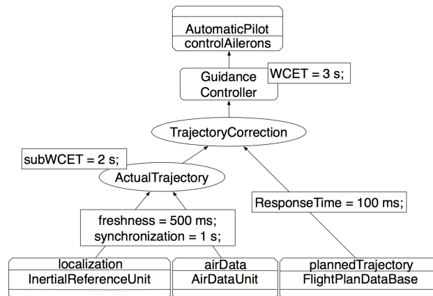
FIGURE 5: Architecture de l'exemple, enrichie de contrats de QoS
