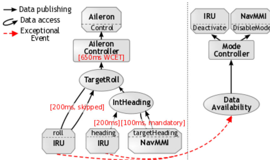
FIGURE 9: Extrait de la conception de l'application de guidage
