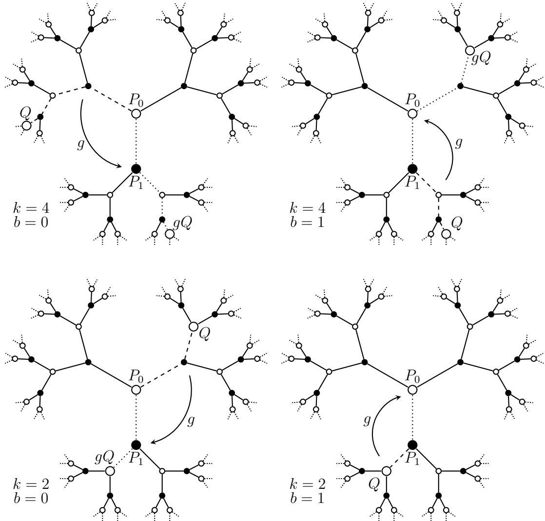
FIGURE 1. PReduce (Subalgorithm 4.2.1.9)
