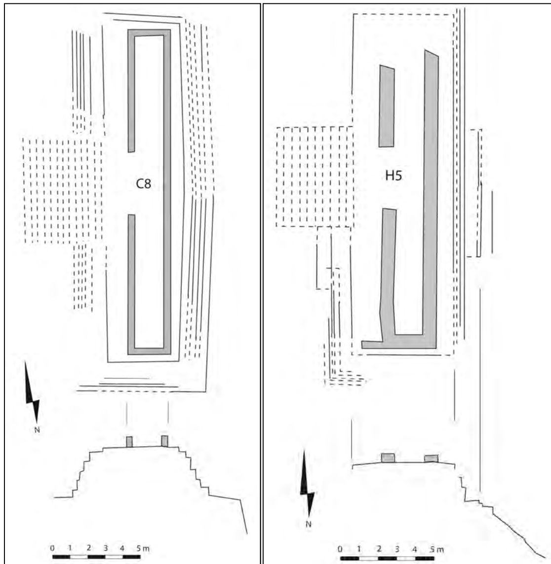
Figure 89 : Relevés en plan des yacatas C8 et H5 de Malpaís Prieto (d'après Michelet 2000).
