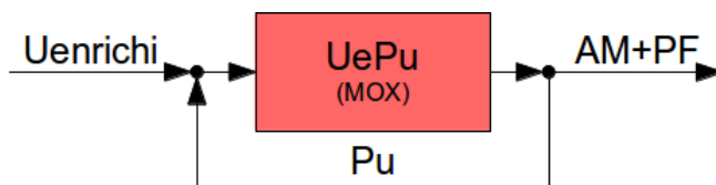
FIGURE 2.2 – Scénario multiUePu. Les flux d'actinides valorisables mais non recyclé (uranium de retraitement) ne sont pas indiqué dans ce schéma
