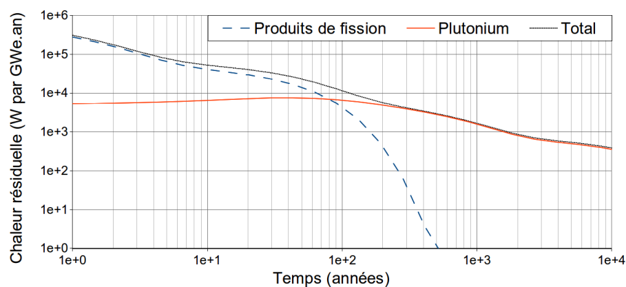
FIGURE 1.4 – Chaleur résiduelle d'un combustible UOX usé
