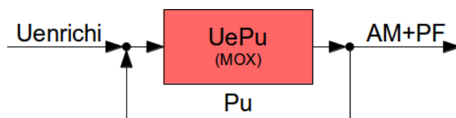
FIGURE 2.2 – Scénario multiUePu. Les flux d'actinides valorisables mais non recyclé (uranium de retraitement) ne sont pas indiqués dans ce schéma
