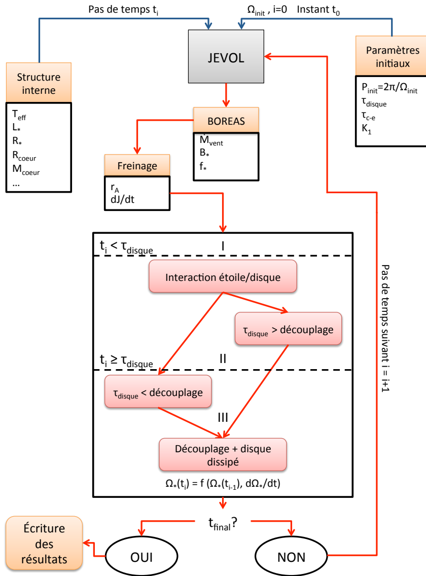
FIGURE 2.1 – Schéma synthétique du code JEVOL.
