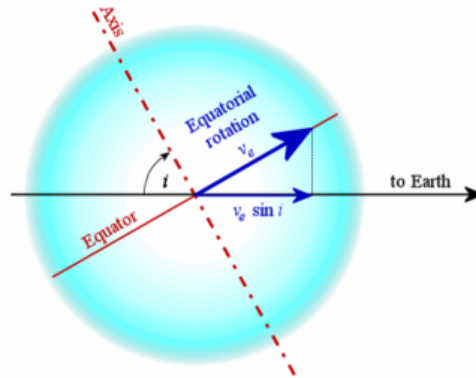
FIGURE 1.5 – Schéma de la mesure de vitesse radiale
