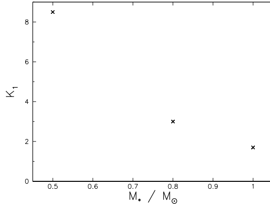
FIGURE 3.12 – Évolution de K_1 en fonction de la masse stellaire.
