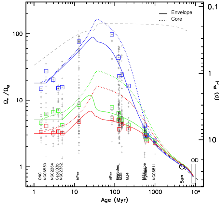
FIGURE 2.15 – Évolution de la vitesse de rotation pour les étoiles de 1 M_{\odot} en fonction du temps. Évolution de la structure interne, freinage par vent stellaire, interaction étoile-disque et découplage coeur-enveloppe. La courbe en pointillé noir représente l'évolution de la vitesse de rupture (équation 1.2).
