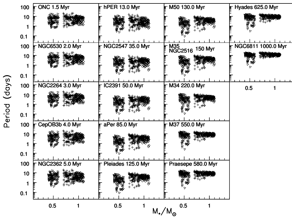
FIGURE 3.17 – Distributions synthétiques obtenues après méthode de Monte-Carlo.
