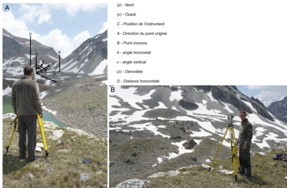
Figure 8-1. Principe et mise en contexte de l'utilisation du tachéomètre électronique pour le suivi des déplacements de surface d'un glacier rocheux. A. Données mesurées et repères mis en contexte sur le terrain. B. Position du tachéomètre à l'aplomb de blocs servant de point de repère
