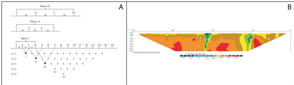
Figure 6-3. Principe de construction d'une pseudo-section (A) (ici pour la configuration de Wenner) et carte de pseudo section (B)
