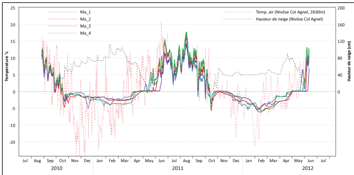
Figure 7-15. Evolution de la température du sol mesurée sur le glacier rocheux du Marinnet, de la température de l'air et de l'enneigement à la station Nivôse des Rochilles, entre Aout 2010 et juin 2012
