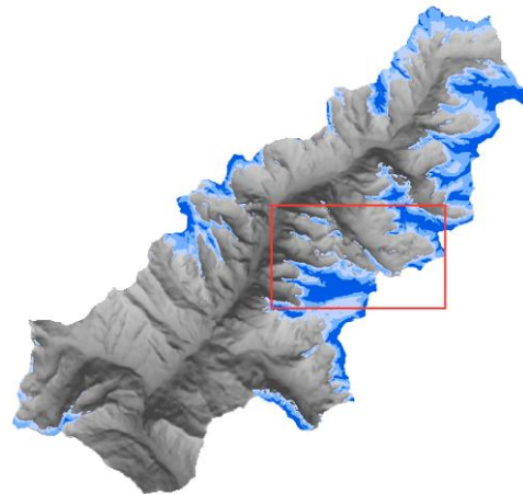
Figure 5-19. Extrait de carte de la distribution du pergélisol et distribution des glaciers rocheux
