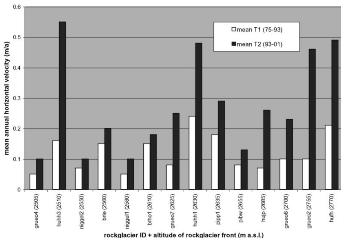
Figure 1-24. Vitesses annuelles moyennes comparées entre la période 1975-1993(T1) et la période 1993-2001(T2) pour 14 glaciers rocheux des Alpes suisses. De gauche à droite, les glaciers rocheux sont classés en fonction de l'altitude du front. D'après Roer et al. , 2005
