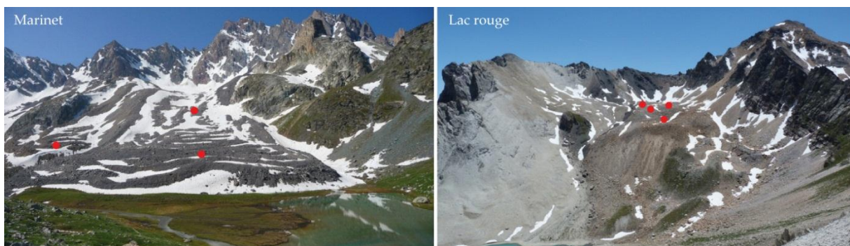
Figure 7-25. Localisation de quelques-uns des emplacements des capteurs ayant présenté un régime thermique théorique de sol à pergélisol au cours des deux années de mesure
