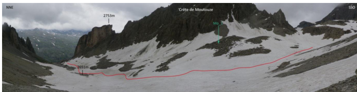
Figure 7-20. Situation de l'enneigement dans le cirque de Moutouze le 12/07/2012. Noter le maintien tardif du couvert neigeux et la variabilité spatiale de ce dernier ; les zones « en relief » sont déneigées de manière plus précoce. Le trait rouge marque le pied du front du glacier rocheux et la flèche turquoise l'emplacement du capteur Mu_1
