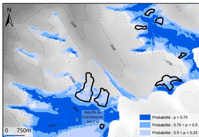
Figure 5-19. Extrait de carte de la distribution du pergélisol et distribution des glaciers rocheux
