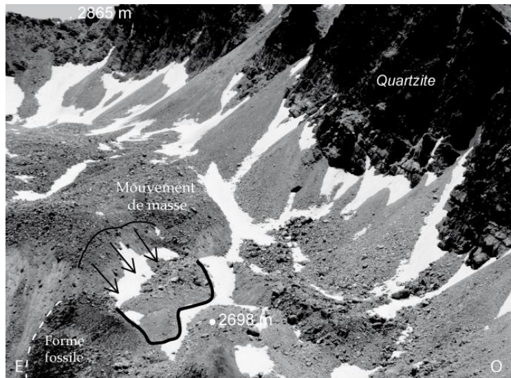
Figure 9-2. Illustration photographique du mouvement de masse présente dans la partie frontale occidentale du glacier rocheux du Lac Rouge
