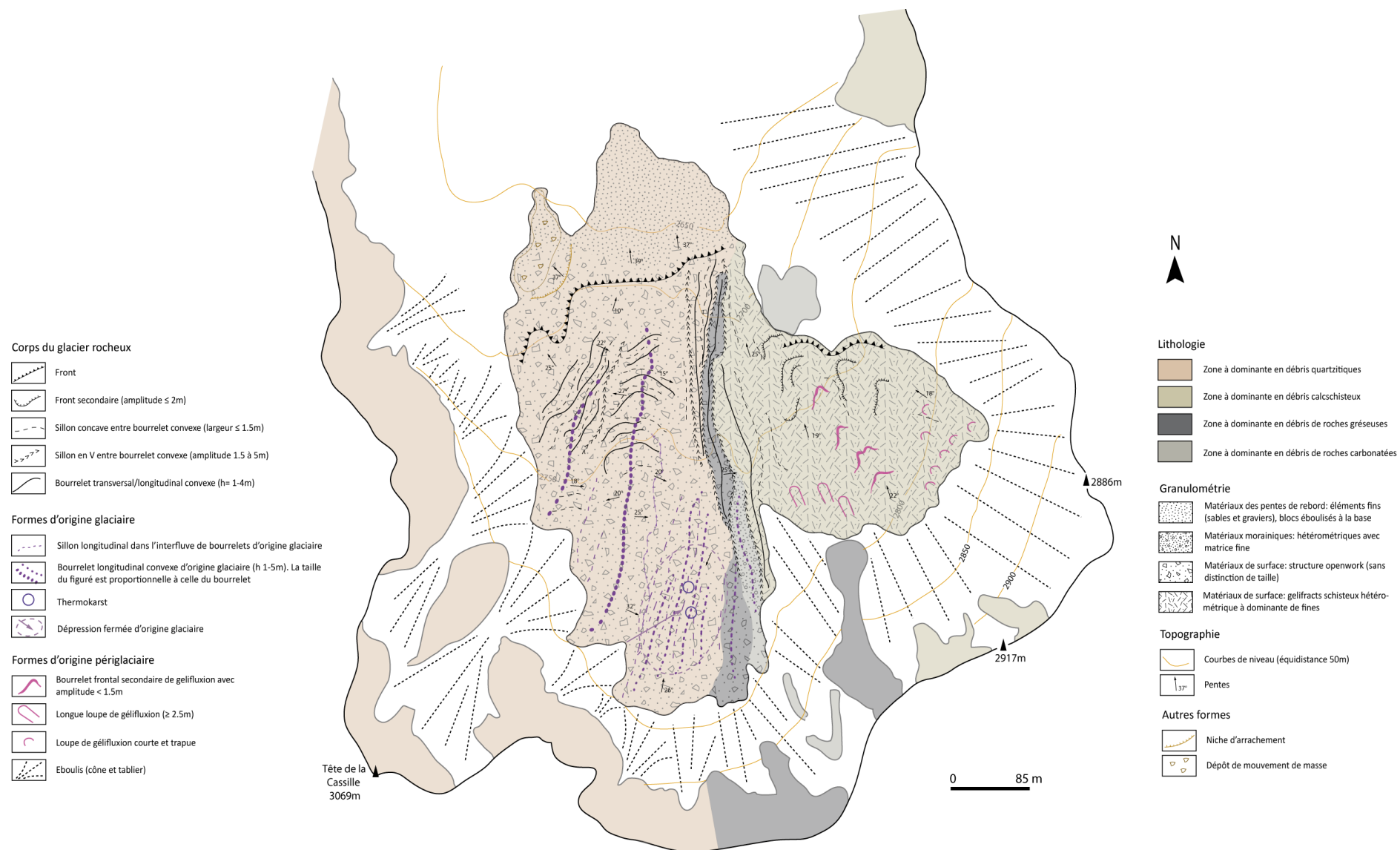
Figure 6-10. Carte géomorphologique du glacier rocheux du Lac Rouge
