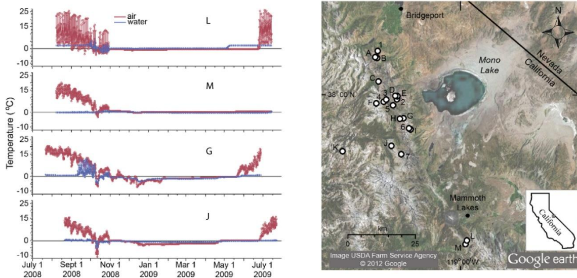
Figure 5-1. Mesures de température d'eau de source et de température de l'air réalisées sur des glaciers rocheux actifs de la Sierra Nevada (Californie, USA). Les lettres situées au-dessus de chaque graphique correspondent à celles présentées sur la carte de localisation. D'après Millar et al. (2012)
