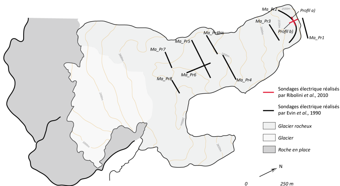
Figure 6-19. Localisation des sondages électriques réalisés à la surface du glacier rocheux du Marinet. D'après Evin et al. (1990) et Ribolini et al. (2010)
