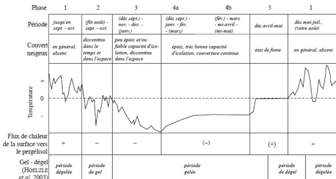
Figure 7-1. Comportement théorique d'un sol à pergélisol en milieu alpin (d'après Delaloye, 2004)
