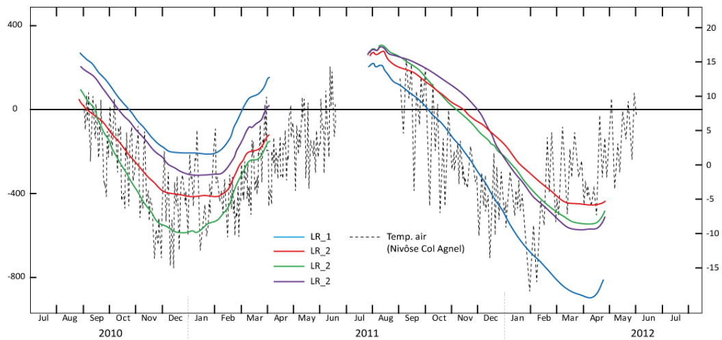
Figure 7-6. Cumul des écarts journaliers entre les températures de l'air (station Nivôse Col Agnel) et les températures du sol, aux sites LR_1, LR_2, LR_3 et LR_4
