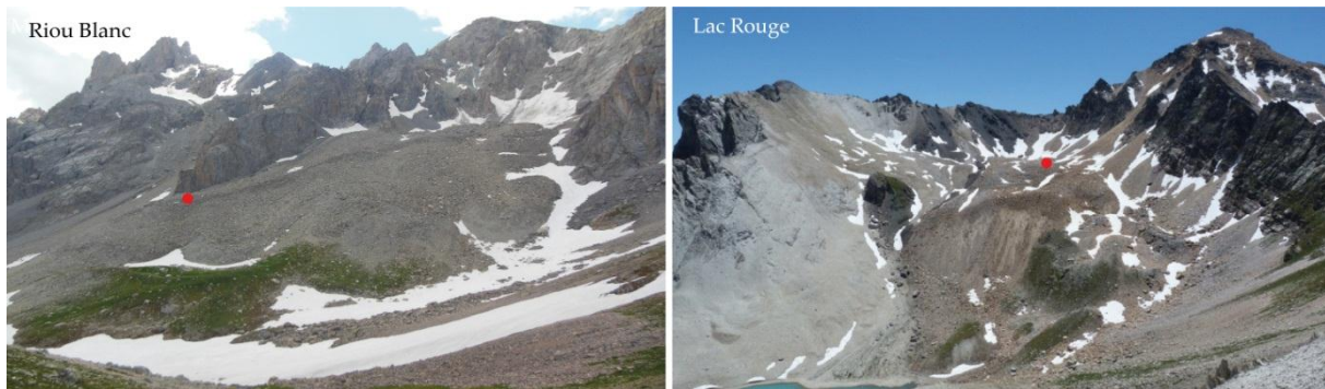
Figure 7-29. Localisation de l'emplacement de capteurs ayant présenté un régime thermique à variabilité annuelle continue durant les deux saisons de mesure
