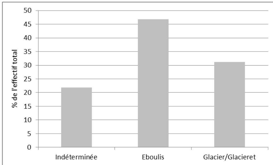
Figure 4-8. Type de transition morphologique entre la racine des glaciers rocheux et leur zone amont (N=55)
