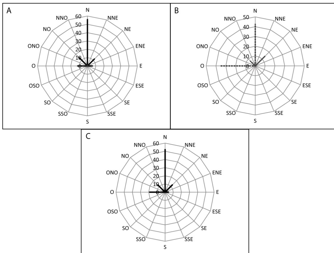
Figure 4-5. Exposition des sites d'occurrence des glaciers rocheux frais. A. Vallée de la Clarée, B. Vallée de l'Ubaye, C. Clarée et Ubaye
