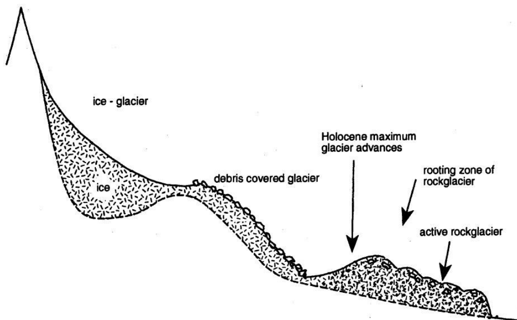
Figure 1-11. Modèle du type « continuum glacier/glacier rocheux » de développement d'un glacier rocheux (modifié de Barsch, 1996)
