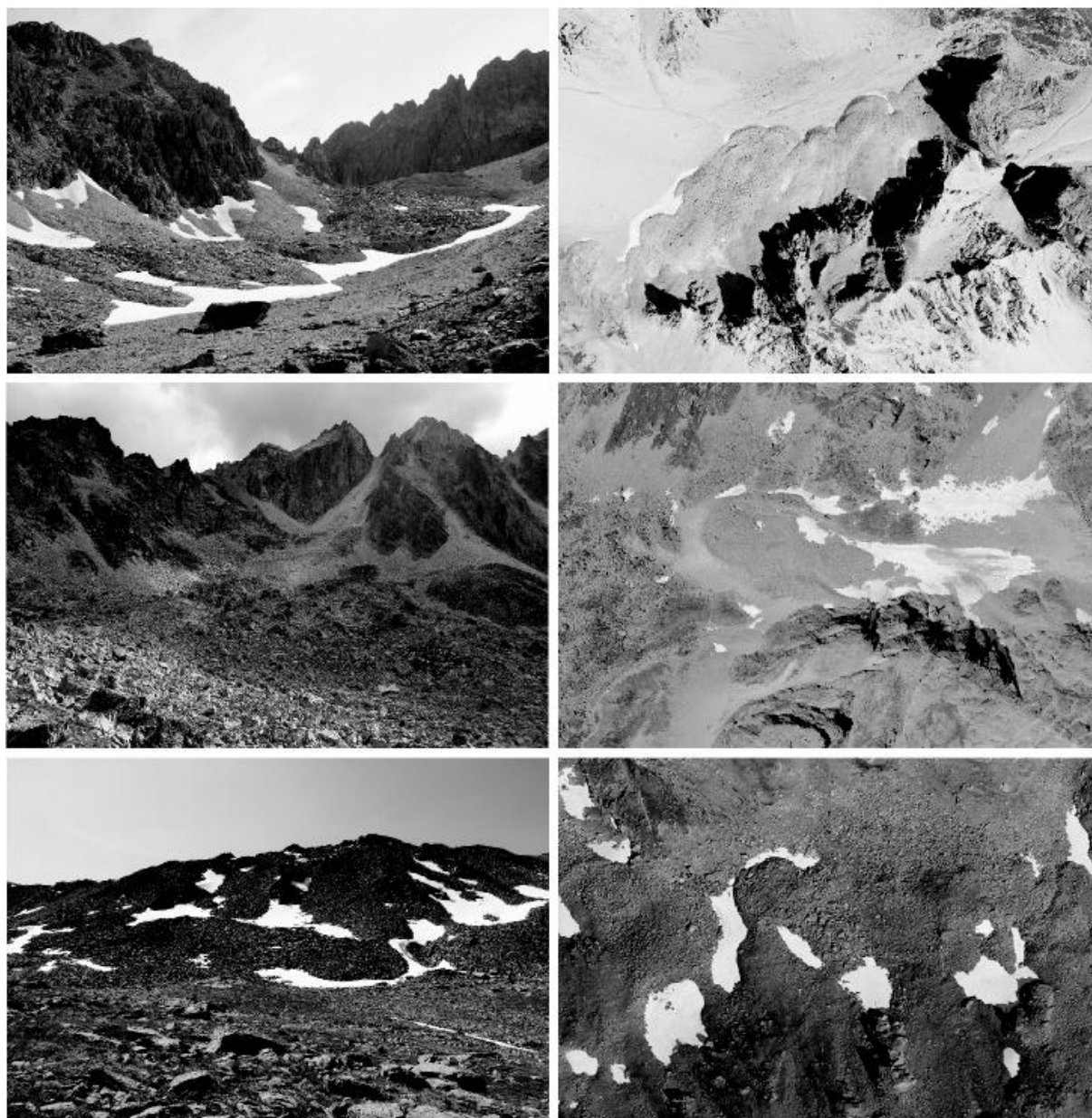
Figure 4-12. En haut, Talus-derived rockglacier lobé (Moutouze, Clarée), au milieu : Talus-derived rockglacier en langue (Tuissier, Ubaye) et en bas : protalus (Muandes, Clarée)
