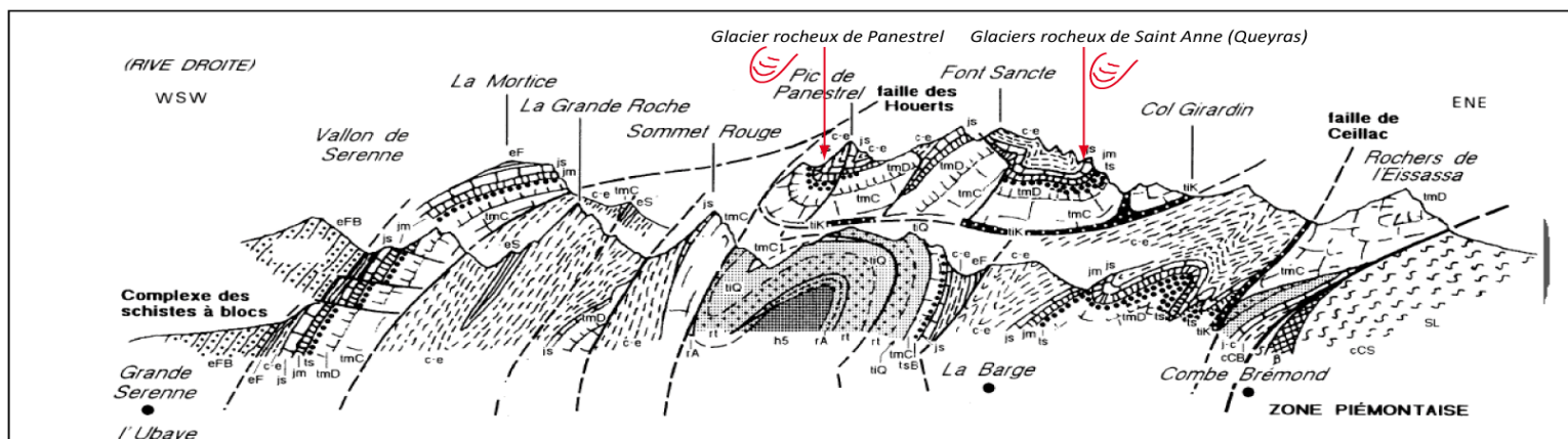
Figure 2-19. Coupes lithologiques dans la haute vallée de l'Ubaye (d'après Gidon et al., 1994). Noter les flèches rouges indiquant la présence de glaciers rocheux le long des profils et les lignes en pointillé qui soulignent les réseaux de faille et de contacts anormaux
