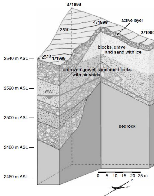
Figure 1-13. Structure interne du glacier rocheux de Muragl (Alpes suisses) déterminée à partir de forages profonds. Tiré d'Arenson et al, 2002
