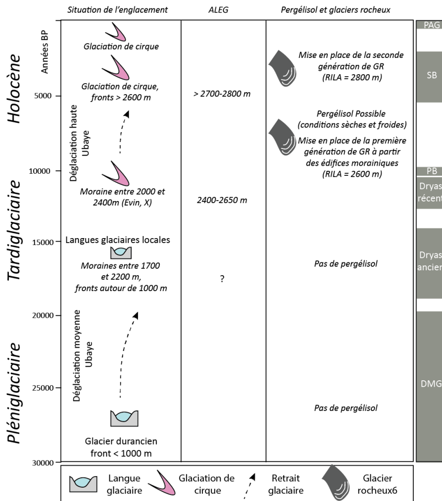
Figure 3-2. Synthèse de l'évolution glaciaire depuis le DMG et mise place des différentes générations de glaciers rocheux dans la haute vallée de l'Ubaye
