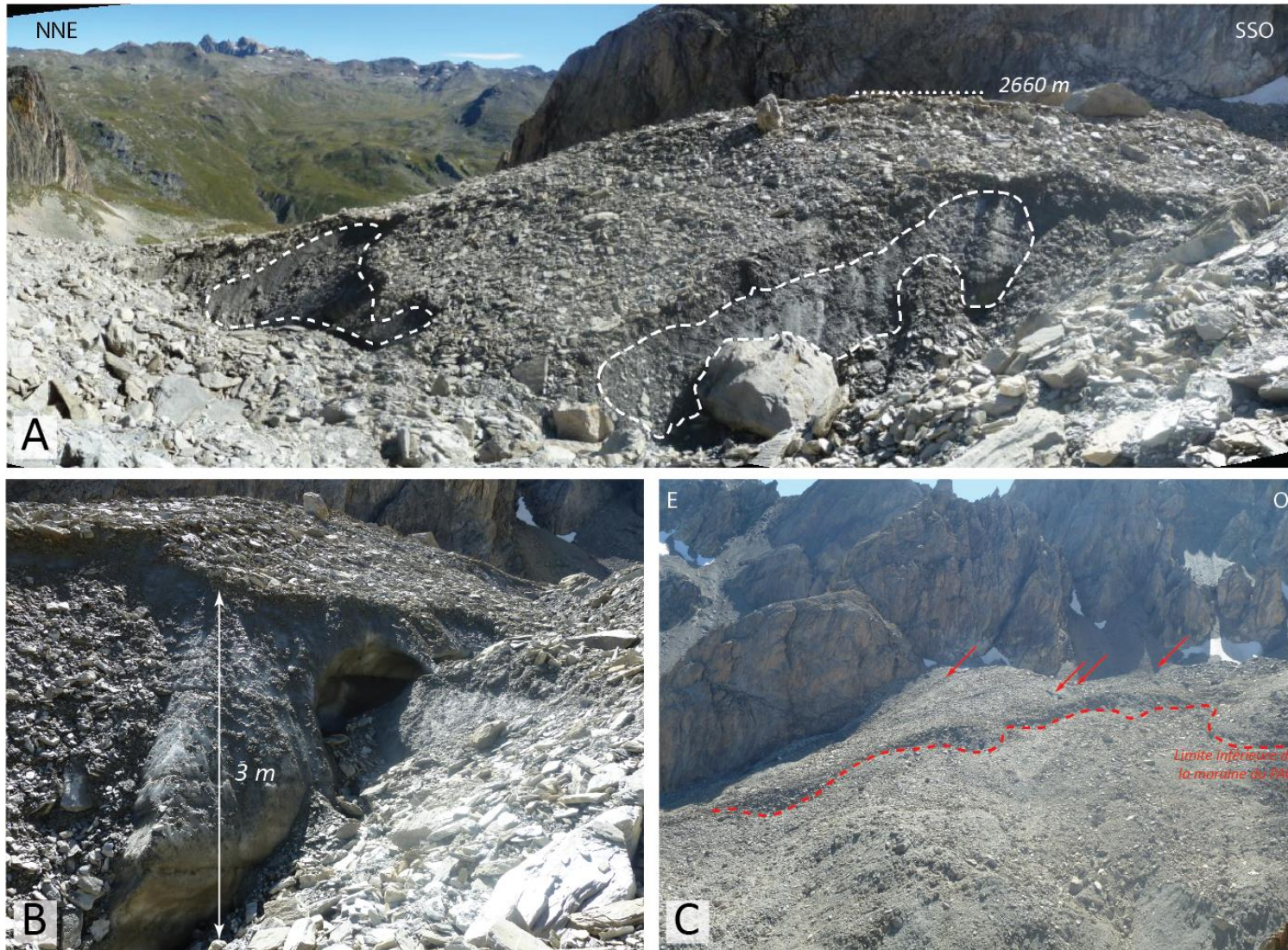
Figure 9-6. Glace massive observée à la surface du glacier rocheux du Riou Blanc. A) Partie amont du glacier rocheux où un corps massif de glace héritée est présent. Celui-ci mesure près de 100 m de diamètre. B) Zoom sur la glace massive observée. Noter l'épaisseur de glace apparente et la couche peu épaisse de débris qui la recouvre. C) Secteurs (flèches rouges) ayant présenté de la glace massive durant l'été 2013
