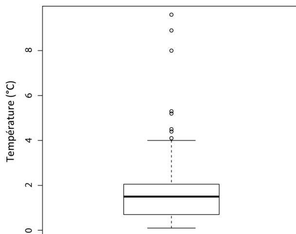
Figure 5-6. Valeurs statistiques (min., max., 1 er et 3 ème quartiles, médiane) des températures d'eau de source mesurées en haute Clarée et en Ubaye (N=108)
