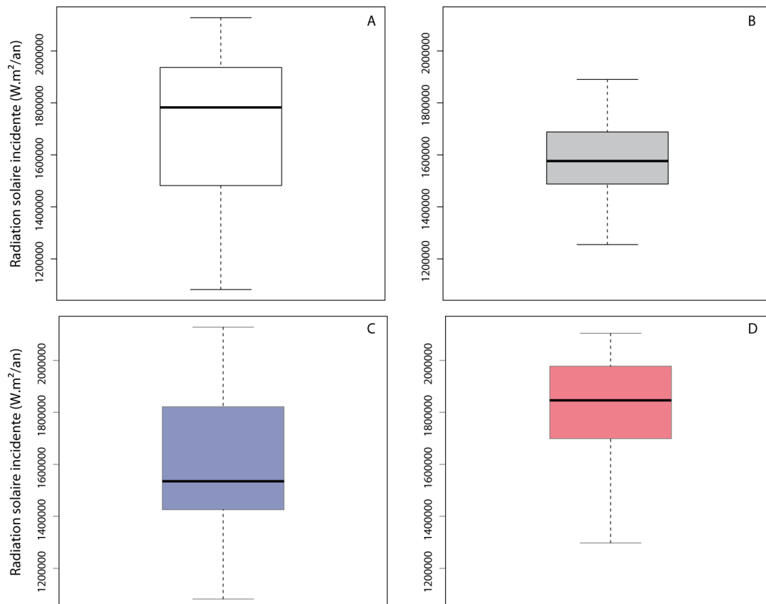
Figure 5-7. Valeurs statistiques (min., max., 1 er et 3 ème quartiles, médiane) de la radiation solaire incidente calculée en chacun des points de mesures de température d'eau de source dans les vallées de la Clarée et de l'Ubaye. A) Clarée B) Ubaye C) Températures inférieures à 1°C (Ubaye/Clarée) D) Températures supérieures à 1°C (Ubaye/Clarée)
