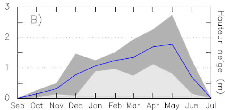
Figure 2-15. Epaisseur moyenne (courbe bleue ; en grisé sombre, l'enveloppe \pm 1\sigma ) du manteau neigeux dans la Combe de Laurichard (2450 m d'altitude, massif du Combeynot sur la période 1979-1986. Données Météo France et Francou, 1988 tiré de Bodin, 2007
