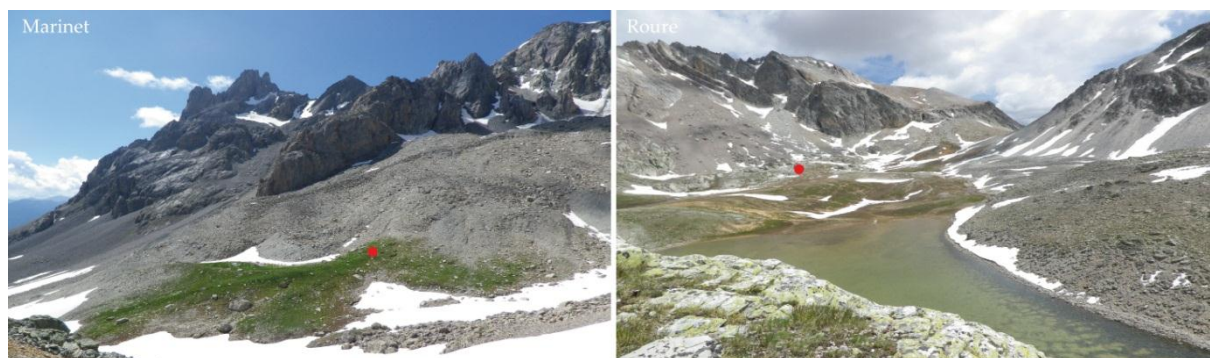
Figure 7-27. Localisation de l'emplacement de capteurs ayant présenté un régime thermique associé à l'absence de pergélisol pendant les deux années de mesure
