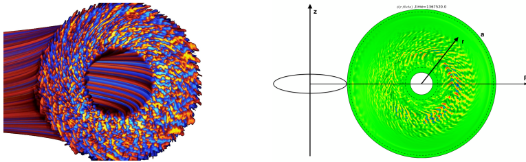
FIGURE 7.1 – Visualisation 3D (à gauche) et coupe poloidale (à droite) de fluctuations du potentiel électrique \phi - \langle \phi \rangle_{FS} . source à gauche : A. Strugarek
