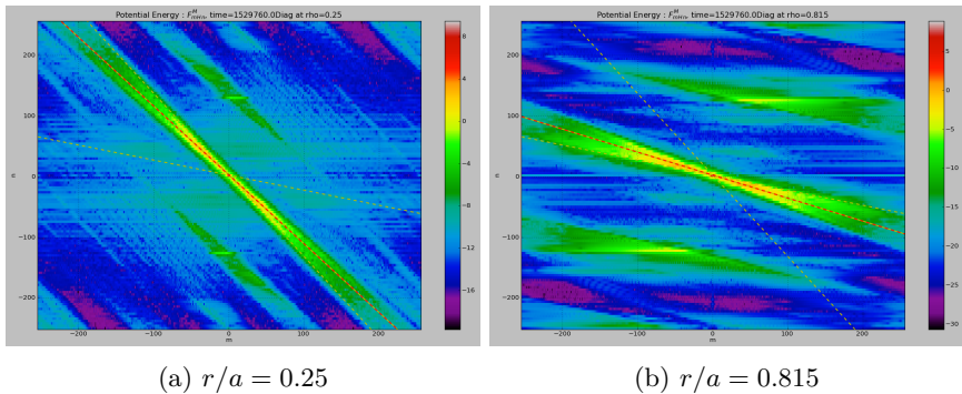
FIGURE 7.2 – Spectres de l'énergie potentielle électrique \phi_{m,n}(r) pour r/a = 0.25 et r/a = 0.81 . On constate que la pente de la droite m + nq = 0 varie puisque q est fonction de r . En conséquence, les modes résonants excités varient.
