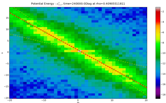
FIGURE 3.3 – Carte de l'énergie potentielle \phi_{m,n}^2(r) dans l'espace (m, n) au centre de la boîte (rayon r/a = 0.5 ). On voit que l'énergie potentielle est concentrée sur l'axe m+nq = 0 (tracé ici en rouge pointillé). On remarquera que cette ligne varie en fonction du rayon car q est fonction de r . Les limites de ces lignes pour les valeurs extrêmes de q sont représentées en orange. Zoom sur les modes proches de (0, 0)
