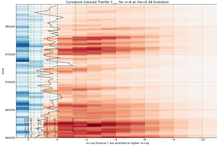
FIGURE 7.6 – Evolution temporelle \Gamma_k^{Curv} en fonction de k_{\parallel}q = m + nq . Les modes résonants équivalents m_{res} à d'autres rayons sont indiqués par les lignes pointillées. En effet, à cause du cisaillement magnétique, q varie, à d'autres rayons, le m_{res} varie d'autant.
