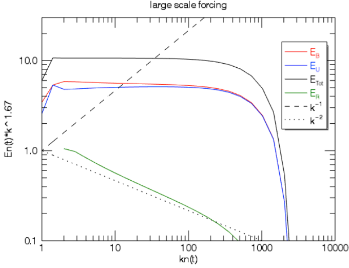
FIGURE 6.6 – Modèle F2 sans expansion : Spectres (compensés par k^{5/3} ) de l'énergie magnétique, cinétique, totale et résiduelle dans un calcul sans expansion, forcé par des grandes échelles à énergie constante. On observe un spectre total en E_T \sim k^{-5/3} et un spectre résiduel en k^{-2} .
