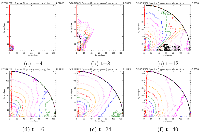
FIGURE 5.1 – Evolution du spectre gyrotropisé de l'énergie magnétique en présence de champ moyen. Simulation homogène avec un champ moyen dans la direction x . On trace des isocontours de l'énergie magnétique, les mêmes niveaux d'énergie sont figurés par les mêmes couleurs. On observe un développement rapide et exclusif de la cascade dans la direction perpendiculaire dans un premier temps 0 < t \leq 12 puis le développement dans la direction parallèle au fur et à mesure jusqu'à atteindre un état quasi stationnaire au temps t = 24 (e). Remarquons que la simulation a été poursuivie jusqu'au temps 80 et qu'il n'y a que très peu de variation du spectre par rapport au temps 40 (f). La courbe rouge proche de l'axe des ordonnées montre l'isocontour \tau_{NL} = \tau_A d'équilibre entre le temps non-linéaire \tau_{NL} = 1/ku et le temps d'Alfvén \tau_A = 1/k_{\parallel}B . Les spectres sont apodisés à partir de k > 128 pour éviter les effets d'aliasing. C'est pourquoi l'énergie chute à 0 à partir de k = 128 .
