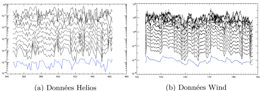
FIGURE 4.7 – Evolution de l’amplitude du spectre de l’énergie magnétique dans les bandes de fréquences de la journée à 1m40 (a) pour Helios et à 6 secondes pour Wind (b), ainsi que de la température des protons (bleu). Les basses fréquences sont classées par leur amplitude. L’amplitude diminue avec la fréquence, les basses fréquences sont donc en haut et les hautes fréquences en bas.
