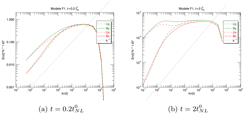
FIGURE 6.5 – Modèle F1 : Evolution temporelle des spectres par composantes, terme dynamo non diagonal à la (6.39). (a) t = 0.01, R = 0.1AU , (b) t = 0.1, R = 1AU . (conditions initiales en k^{-1} isotropes en R= Paramètres du modèle. N_{shell} = 20, d = 2, t_{NL}^0 = 0.05, \nu = 10^{-6}, B_0 = 0, U_0 = 100, u_0 = 1, \alpha = 0, \beta = 1, \gamma = 1 . où t_{NL}^0 est le temps non-linéaire des plus grandes échelles au temps initial.
