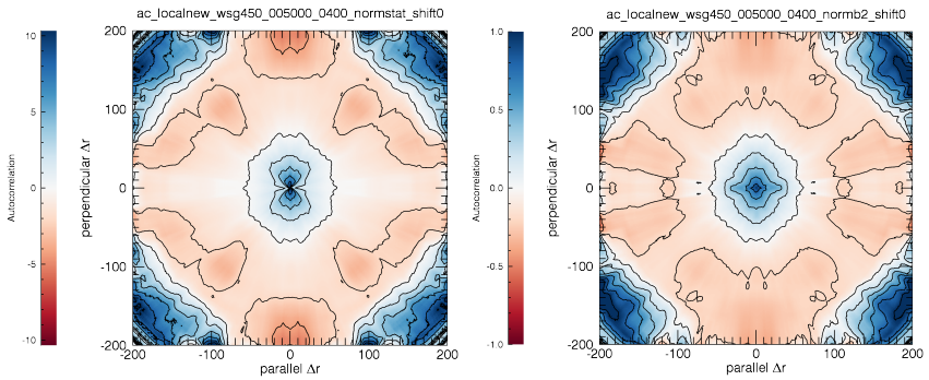
(c) Vents rapides (>450km/s) sans normalisation. (d) Vents rapides (>450km/s) normalisé par B^2 .
