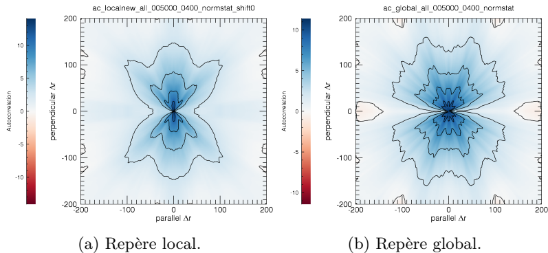
FIGURE 5.6 – Fonctions d’autocorrélations calculées sur toute la période mesurée par Wind, dans le repère local (a) (eq. 5.19) ou le repère global (b) (eq. 5.20). En abscisse, la direction parallèle au champ moyen, en ordonnée, la direction perpendiculaire.
