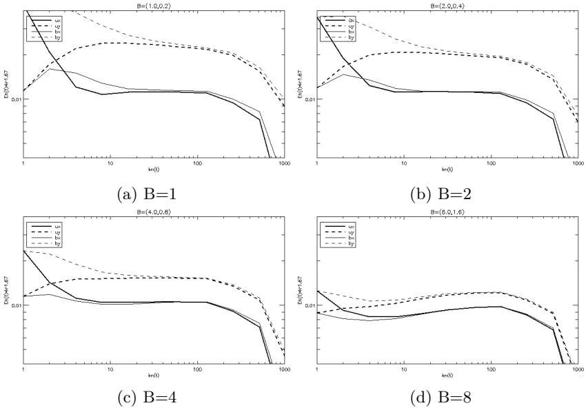
FIGURE 6.12 – Inégalité de polarisation de l'énergie totale et importance du champ moyen.
