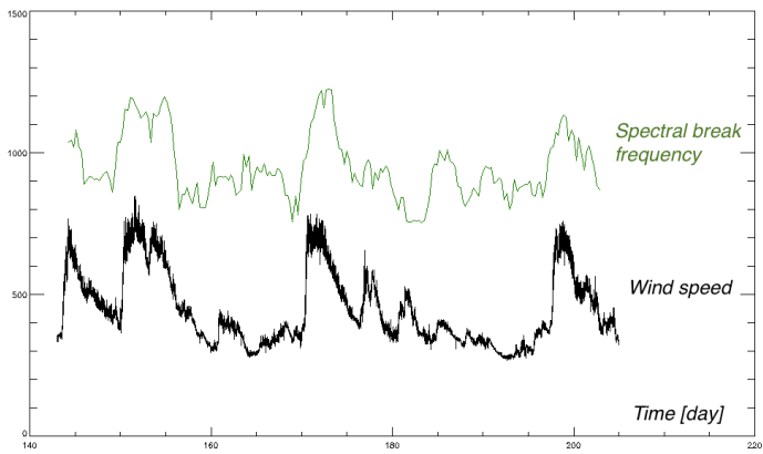
FIGURE 4.15 – Corrélation entre la vitesse du vent (noir) et la fréquence de cassure de pente (vert). Données Wind.
