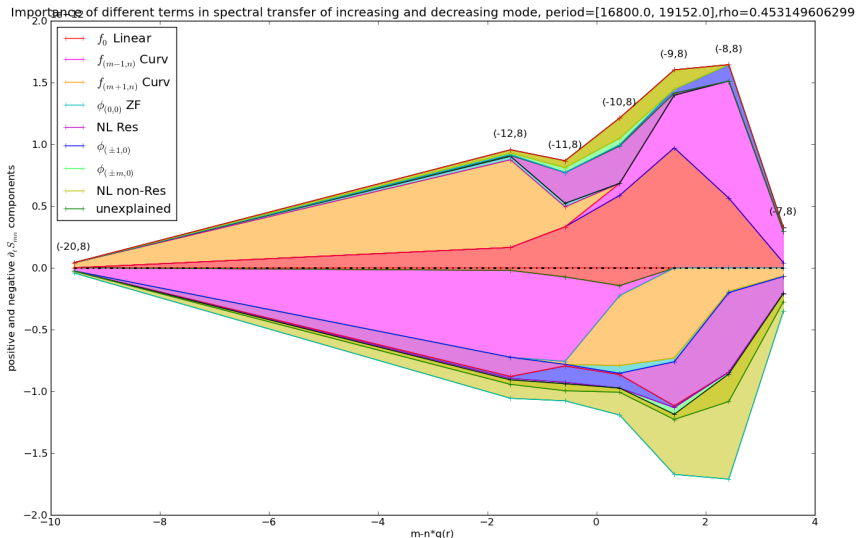
FIGURE 7.4 – Moyenne temporelle des transferts spectraux pour le mode (m, n = 8) au rayon r/a = 0.49 , en fonction du sens du transfert et de la résonance du mode m + nq . Les surface au dessus de y = 0 représentent les transferts positifs (ou les sources d'entropie) et les surfaces au dessous des y = 0 les transferts négatifs (ou les puits d'énergie) (voir texte). On peut voir une source d'énergie issue d'une excitation linéaire (sans doute des ITG) autour des modes les plus résonants, qui est répartie sur les modes environnants via le terme de courbure (ou couplage toroidal).
