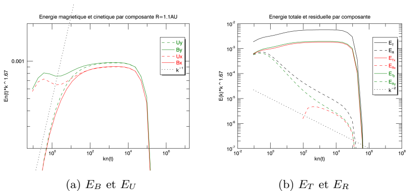
FIGURE 6.8 – Modèle F2 : Spectres par composante (compensés par k^{5/3} ) dans un calcul avec expansion au rayon R = 1.1A.U. (avec conditions initiales isotropes à R=0.1 ). (a) E_B et E_U à gauche, E_T et E_R (b) à droite. On peut voir à gauche les orderings obtenus dans EBM ( B_y > U_x > B_x \approx U_y aux grandes échelles et B_y > U_y > B_x > U_x aux petites échelles). On peut également observer à droite les énergies totales en k^{-5/3} et les énergies résiduelles en k^{-2} pour chaque composante. On peut d'ailleurs vérifier que B_x > U_x aux petites échelles.
