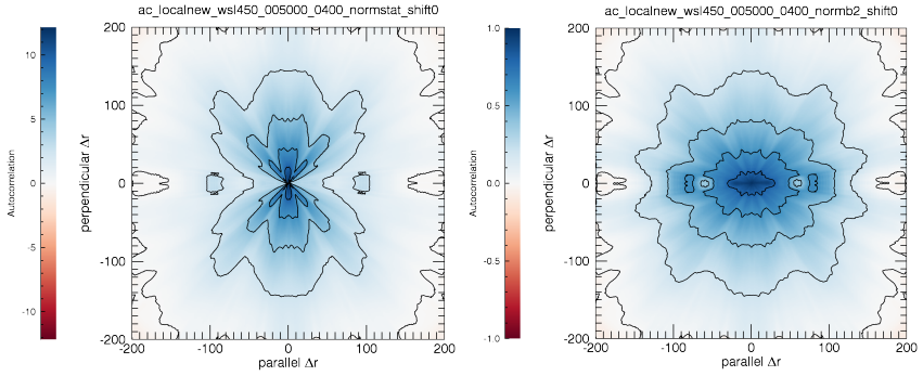
(a) Vents lents (<450km/s) sans normalisation. (b) Vents lents (<450km/s) normalisé par B^2 .
