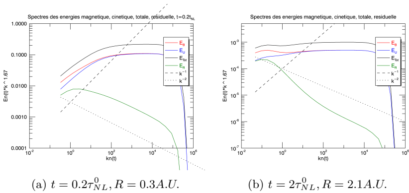
FIGURE 6.7 – Modèle F2 avec expansion : Spectres (compensés par k^{5/3} ) de l'énergie magnétique, cinétique, totale et résiduelle dans un calcul avec expansion, équivalent au calcul E, avec une expansion R(t_f) = 10R(t_0) . A gauche, (a) t = 0.2\tau_{NL}^0, R = 0.2A.U. , on observe une bonne conservation du spectre en k^{-1} jusqu'à k = 10 \sim 10^2 , à droite (b), à 2 U.A., on voit que le spectre en k^{-1} a presque entièrement disparu au profit du spectre en k^{-5/3} . Le spectre résiduel en proche du k^{-2} uniquement dans les plus grandes échelles.
