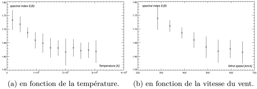
FIGURE 4.10 – Dépendance de l’indice spectral de la zone inertielle en fonction de paramètres du plasma. On fait figurer les barres d’erreurs qui représentent un \sigma de répartition statistique des pentes mesurées. Données Wind.
