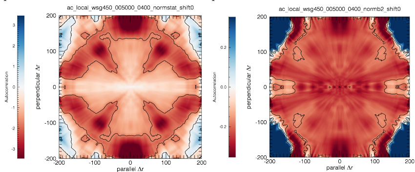
(d) Vents rapides ( >450\text{km/s} ) sans normalisation. (e) Vents rapides ( >450\text{km/s} ) normalisé par B^2 .
