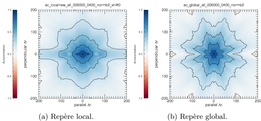
FIGURE 5.7 – Fonction d’autocorrélation calculée sur toute la période mesurée par Wind, normalisée par B^2 , voir texte (5.27), dans le repère local (a) (eq. 5.19) ou global (b) (eq.5.20). En abscisse, la direction parallèle au champ moyen, en ordonnée, la direction perpendiculaire. En raison d’échantillonnage insuffisant, les régions sur l’axe des abscisse sont très bruitées.
