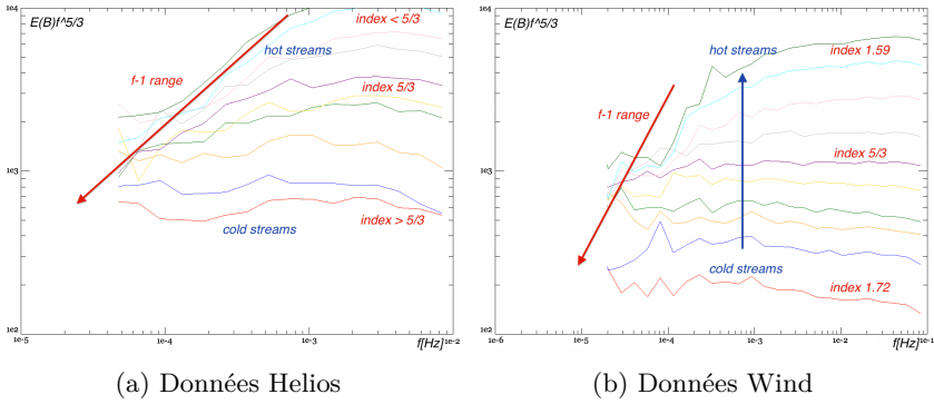
FIGURE 4.8 – Spectres de l’énergie magnétique en moyenne par tranche de température. On constate une amplitude croissante et des pentes décroissantes en fonction de la température. Les spectres sont compensés de telle sorte que E(f)f^{5/3} est représenté. Les mêmes intervalles de température sont représentés par les mêmes couleurs dans les deux figures.
