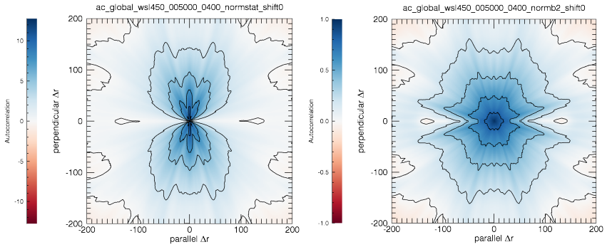
(a) Vents lents ( <450\text{km/s} ) non normalisé. (b) Vents lents ( <450\text{km/s} ) normalisé par B^2 .
