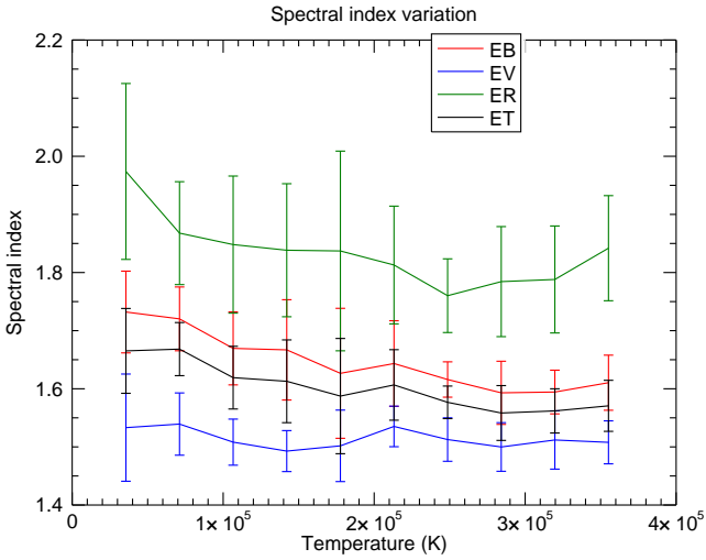
FIGURE 4.12 – Dépendance de l'indice spectral de la zone inertielle des énergies magnétique, cinétique, totale et résiduelle en fonction de la température. Données Wind.
