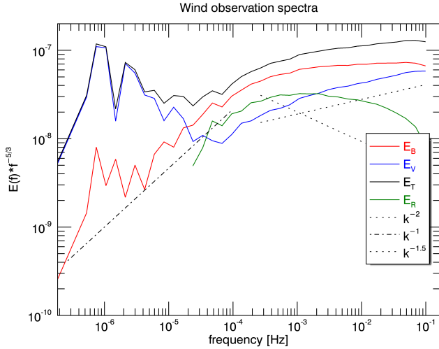
FIGURE 4.6 – Spectres des champs magnétique (rouge), cinétique (bleu), total (noir) et résiduel (vert) mesurés par la sonde Wind, compensé par f^{-5/3} pour mettre en évidence les pentes des spectres et leur dépendance avec l'échelle. On a indiqué les pentes f^{-1} (point-tiret), f^{-3/2} (pointillé croissant) et f^{-2} (pointillé décroissant).
