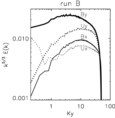
FIGURE 6.3 – Spectres réduits E(K_y) compensés par K_y^{-5/3} en fonction du nombre d'onde perpendiculaire à la radiale K_y , pour les composantes x et y des champs magnétique et cinétique pour la simulation B au temps t = 2 . On remarque les différentes inégalités entre les amplitudes de l'énergie des différentes composantes. Aux grandes échelles, nous observons B_y > U_x > U_y > B_x et B_y > U_y > B_x > U_x aux petites échelles. (figure tirée de l'article, fig. 12c)
