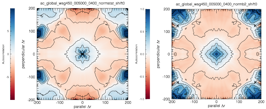
(c) Vents rapides ( >450\text{km/s} ) non normalisé. (d) Vents rapides ( >450\text{km/s} ) normalisé par B^2 .
