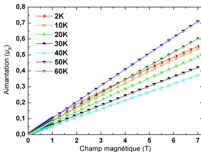
Figure 9-12 – Courbes d'aimantation obtenues entre 2K et 60K dans la gamme [0 – 7T].
