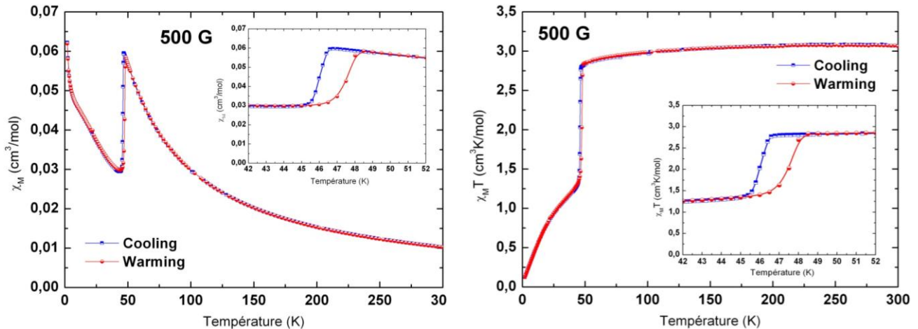
Figure 9-10 – Evolution de la susceptibilité magnétique, mesurée à 500G en descente et remontée en température, représentée sous la forme (a) \chi = f(T) et (b) \chi T = f(T) .
