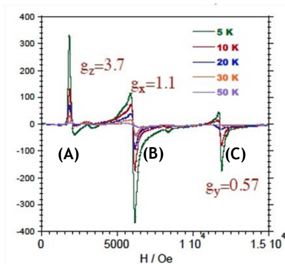
Figure 7-20 – Spectres RPE obtenus sur un échantillon de poudre dans la gamme de température 5K–50K (bande X).
