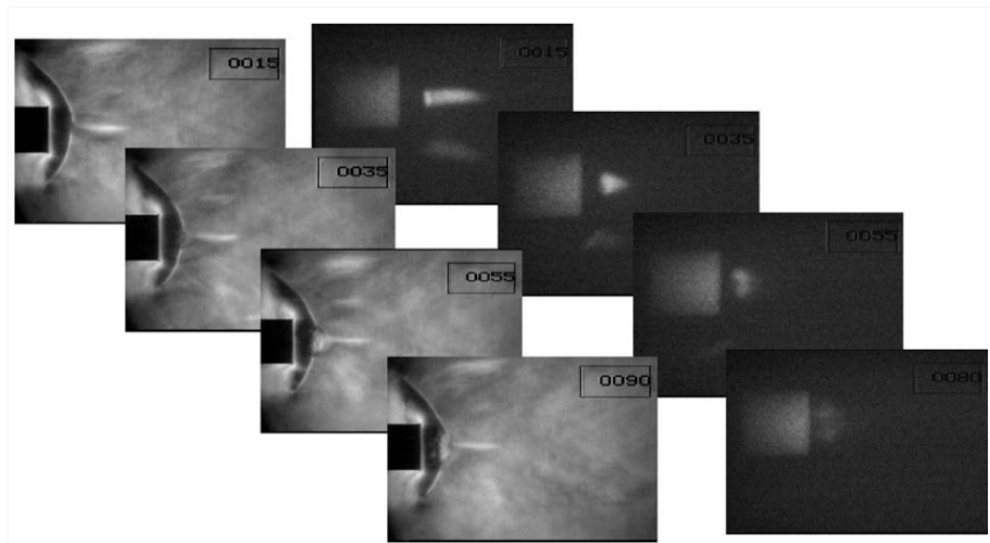
Figure 10: L'interaction du plasmoïde avec le corps de cylindre ( M = 2,1 , temps en ms) [20]. .
