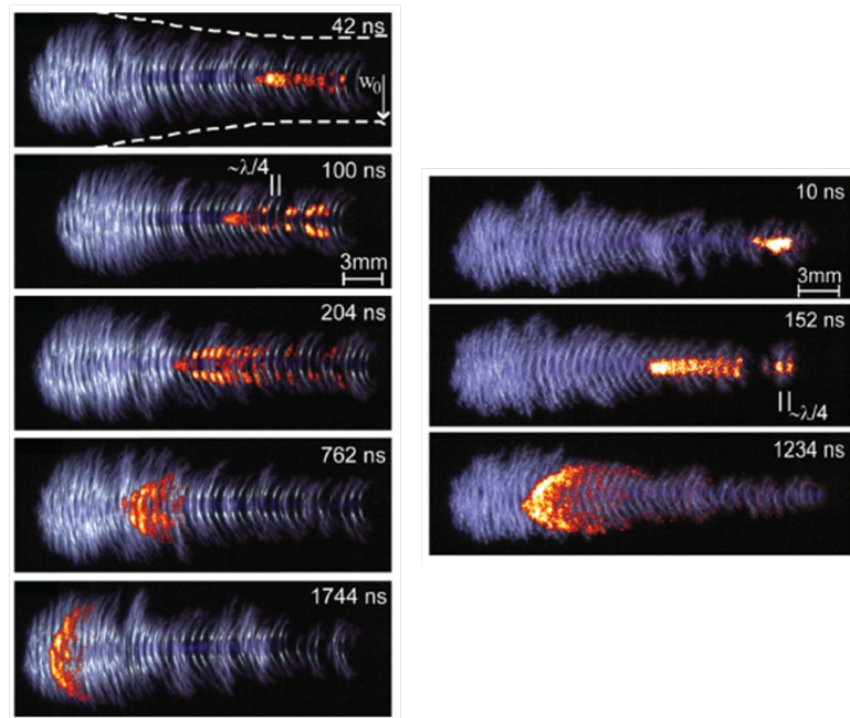
Figure A.3: Decharge microondes avec une polarisation linéaire (gauche) et circulaire (droite) [8].
