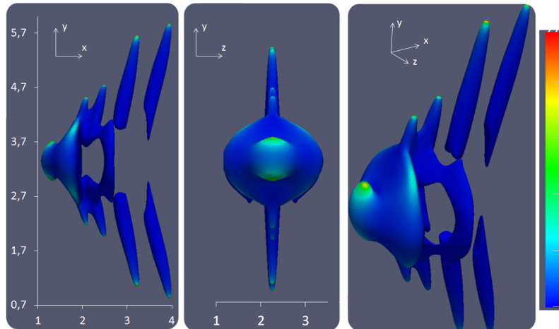
Figure A.7: Iso-surfaces ( 1 \times 10^{21} \text{ m}^{-3} ) contours de la densité électronique colorés par la fréquence d'ionisation, t = 70 \text{ ns} , XY (gauche), YZ (milieu) et 3D (droite). Valeurs max. 9.7 \times 10^9 \text{ s}^{-1} .
