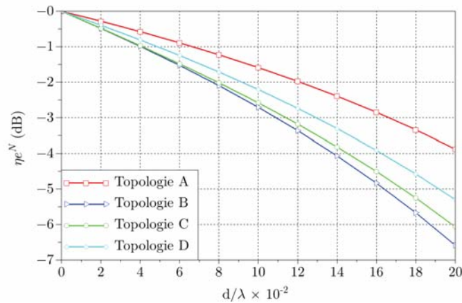
FIGURE II.12 – Critère d'efficacité d'estimation relative à l'antenne composée de six éléments colocalisés en fonction de d/\lambda pour quatre topologies A,B,C et D.
