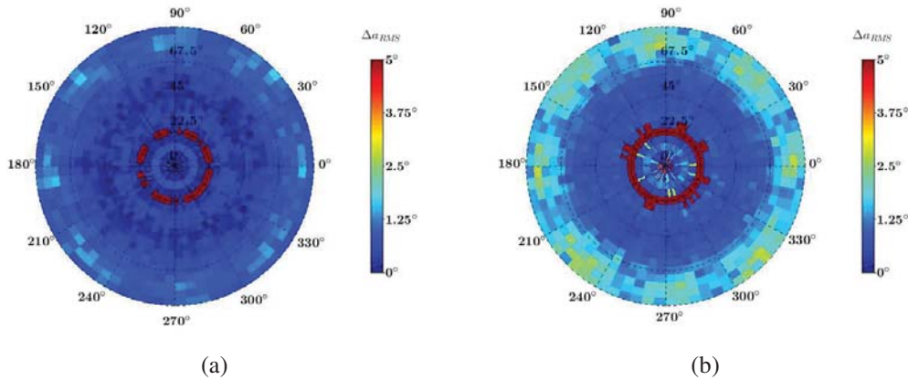
FIGURE III.9 – Erreur RMS \Delta_{a\text{RMS}}(\phi, \theta) simulée de l'antenne Cloc obtenue à l'aide de MUSIC avec (a) P_r = -95\text{dBW.m}^{-2} et (b) P_r = -100\text{dBW.m}^{-2} .
