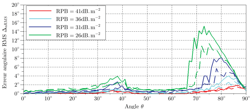
FIGURE V.26 – Erreur RMS \Delta_{aRMS} avec l'antenne bibrande (ligne en pointillé) et l'antenne tribande (ligne solide), simulée pour RPB = 41dB.m -2 , 36dB.m -2 , 31dB.m -2 et 26dB.m -2 , N=100 and L=20, à 1795MHz dans le plan E à \phi = 0^\circ .
