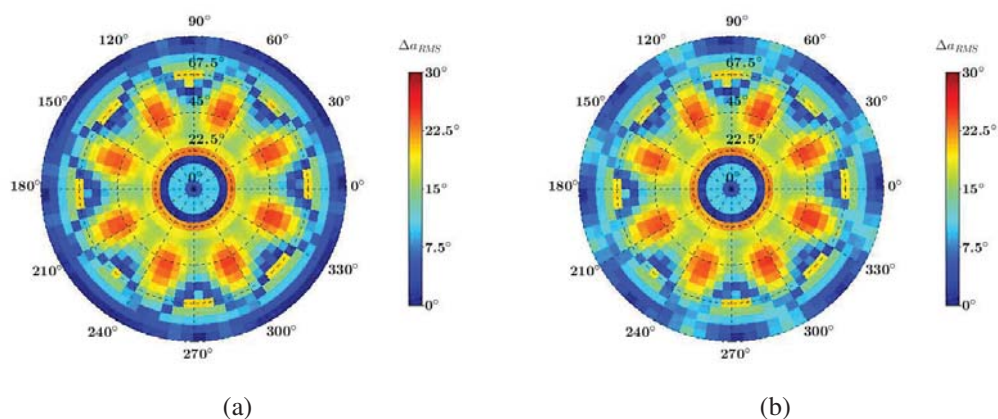
FIGURE III.11 – Erreur RMS \Delta\alpha_{RMS}(\phi, \theta) simulée de l'antenne Cloc obtenue à l'aide de l'algorithme DHS avec (a) P_r = -95\text{dBW.m}^{-2} et (b) P_r = -100\text{dBW.m}^{-2} .
