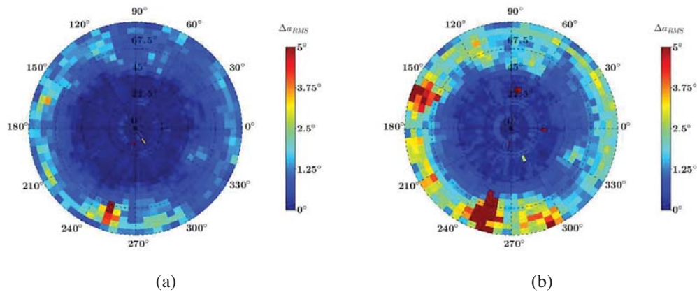
FIGURE III.25 – Erreur RMS \Delta\alpha_{RMS}(\phi, \theta) simulée de l'antenne Dloc obtenue à l'aide de MUSIC avec (a) P_r = -95\text{dBW.m}^{-2} et (b) P_r = -100\text{dBW.m}^{-2} .
