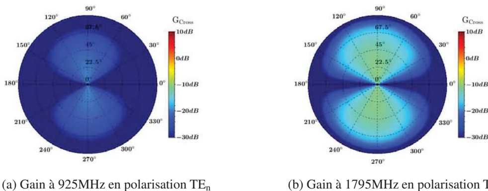
FIGURE IV.18 – Gain simulé du capteur électrique bibande en polarisation croisée à (a) 925MHz et (b) 1795MHz.
