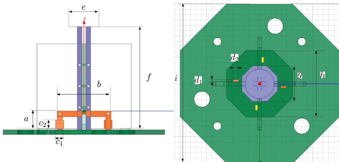
FIGURE III.2 – Antenne Cloc à trois éléments rayonnants colocalisés.
