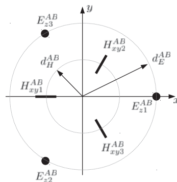
FIGURE IV.3 – Topologie de l'antenne vectorielle bibande à six capteurs spatialement répartis.
