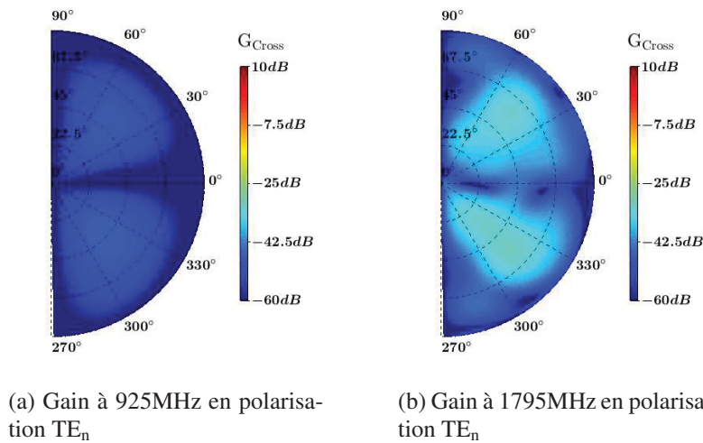
FIGURE IV.30 – Gain simulé du capteur magnétique bibande en polarisation croisée à (a) 925MHz et (b) 1795MHz.
