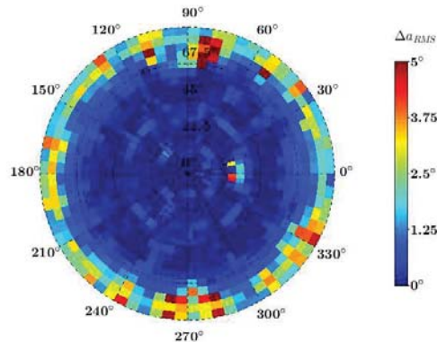
FIGURE III.26 – Erreur RMS \Delta\alpha_{RMS}(\phi, \theta) simulée de l'antenne Dloc sur un support métallique 800x800mm pour P_r = -95\text{dBW.m}^{-2} obtenue à l'aide de MUSIC.
