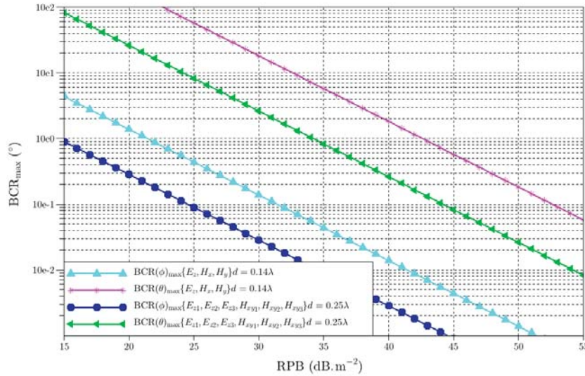
FIGURE IV.32 – \text{BCR}(\phi) et \text{BCR}(\theta) maximales obtenues dans l'ensemble du demi-espace 3D, à partir de l'antenne Dloc ( d = 0.14\lambda ) et de l'antenne vectorielle bibande ( d = 0.25\lambda ), en polarisation \text{TM}_z .
