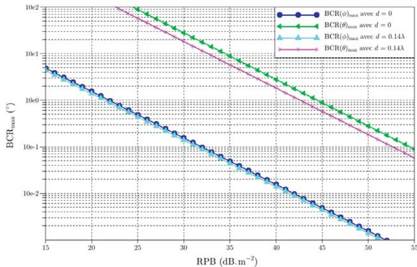
FIGURE III.21 – BCR( \phi ) et BCR( \theta ) maximales obtenues dans l'ensemble du demi-espace 3D, à partir de l'antenne Cloc ( d = 0 ) et de l'antenne Dloc ( d = 0.14\lambda ), en polarisation \text{TM}_z .
