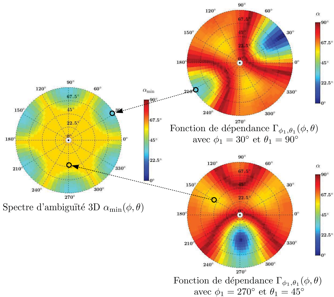
FIGURE II.16 – Illustration de l'extraction des \alpha minimaux des fonctions d'ambiguïtés pour établir le spectre d'ambiguïtés 3D, exemple à (\phi = 30^\circ, \theta = 90^\circ) et (\phi = 270^\circ, \theta = 45^\circ) .
