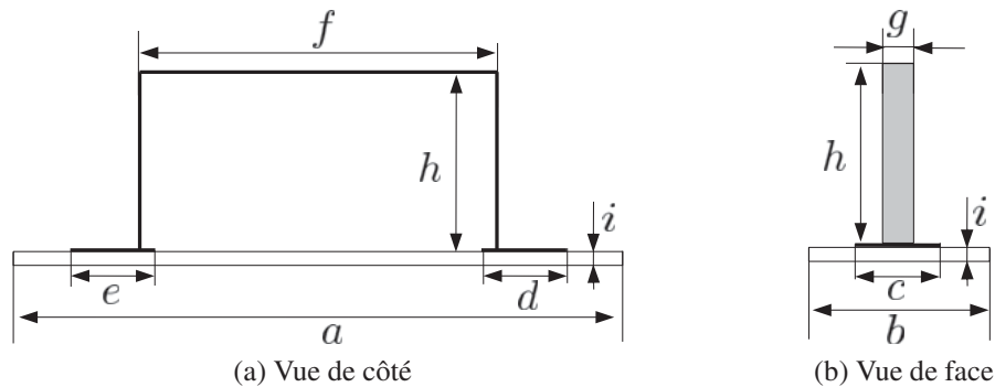
FIGURE V.10 – Demi-boucle chargée couvrant la bande [400MHz-430MHz]
