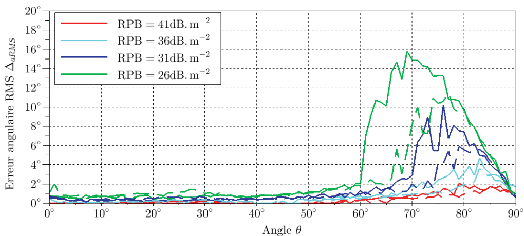
FIGURE V.25 – Erreur RMS \Delta_{aRMS} avec l'antenne bibrande (ligne en pointillé) et l'antenne tribande (ligne solide), simulée pour RPB = 41dB.m -2 , 36dB.m -2 , 31dB.m -2 et 26dB.m -2 , N=100 and L=20, à 925MHz dans le plan E à \phi = 0^\circ .
