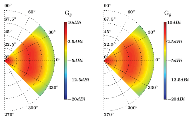
FIGURE III.16 – Gain simulé et mesuré du capteur électrique E_z et des capteur magnétiques H_x et H_y de l'antenne Cloc en polarisation TM_z à 2800MHz.
