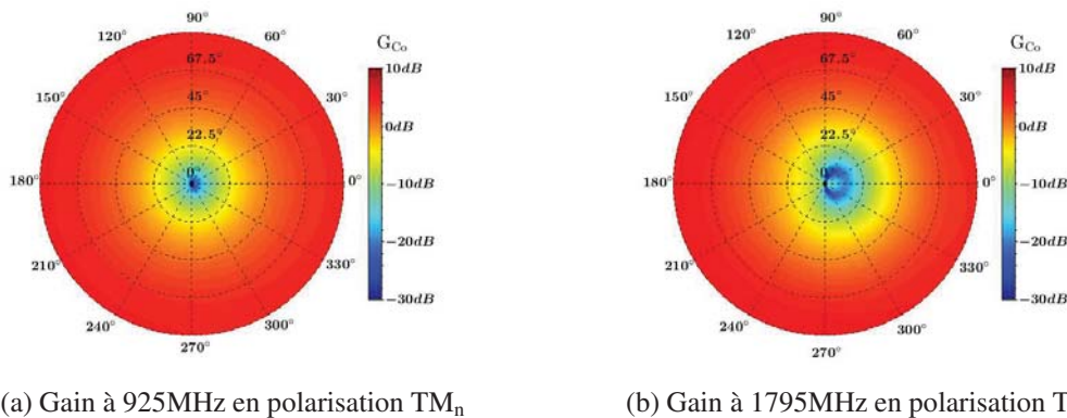
FIGURE IV.17 – Gain simulé du capteur électrique bibande en co-polarisation à (a) 925MHz et (b) 1795MHz.
