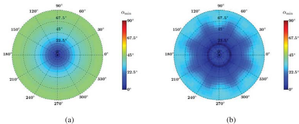
FIGURE III.8 – Spectres d'ambiguïtés 3D de l'antenne Cloc pour d = 0 obtenus par (a) calcul analytique et par (b) simulation numérique.
