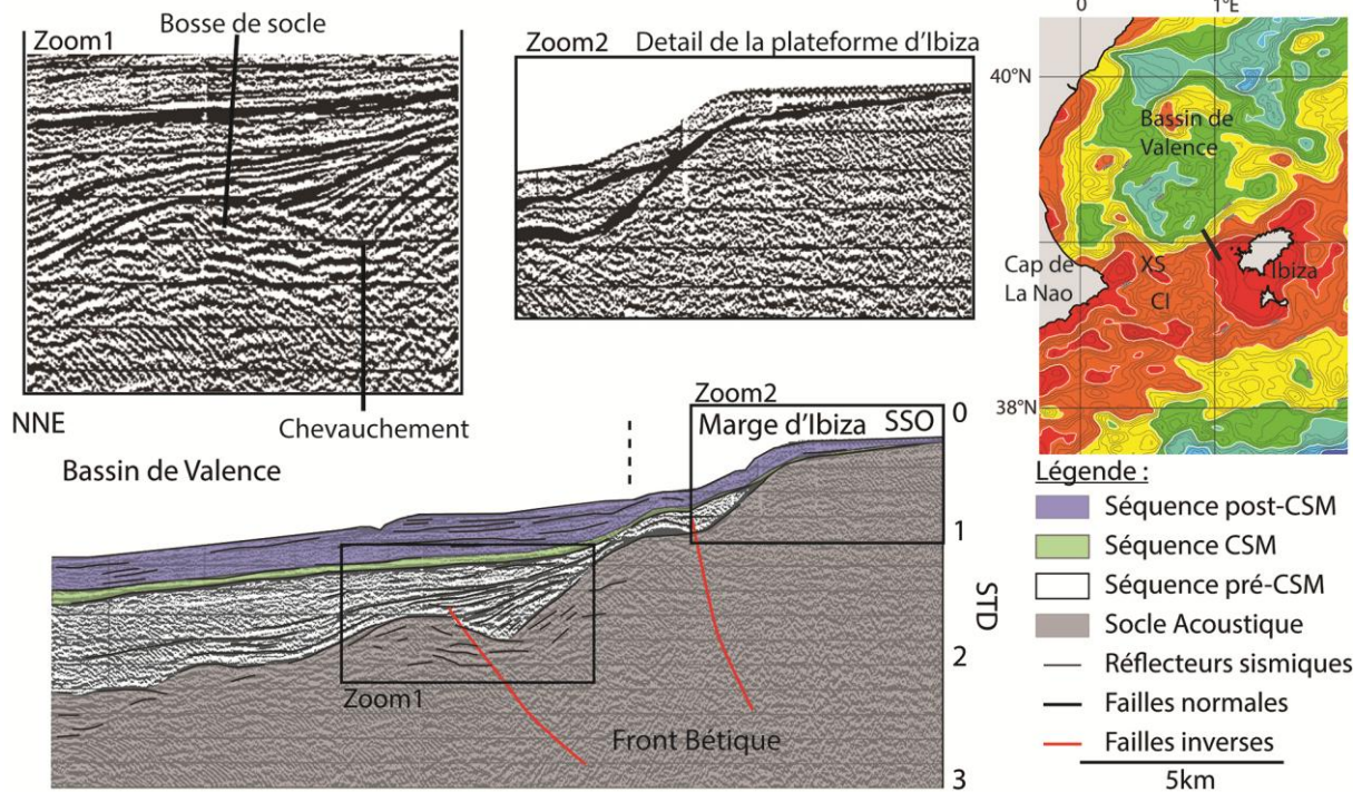
Figure III. 22: Profil de sismique-réflexion Meds77-28 montrant l'influence des chevauchements bétiques sur la structure et la morphologie de la marge nord d'Ibiza. Exagération verticale = 3.5. XS : Mont Xabia ; CI : Chenal d'Ibiza
