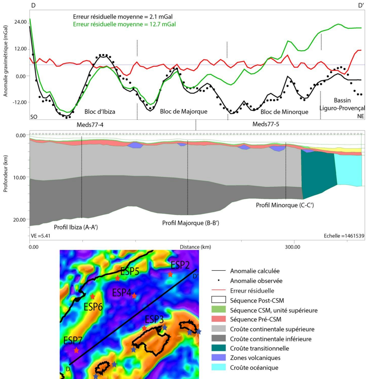
Figure III. 19: section gravimétrique DD' longitudinale au bassin de Valence le long des profils Meds77-4 et Meds77-5 localisés sur la carte de l'anomalie à l'air libre. La courbe verte correspond à un modèle où la croûte transitionnelle est remplacée par de la croûte continentale
