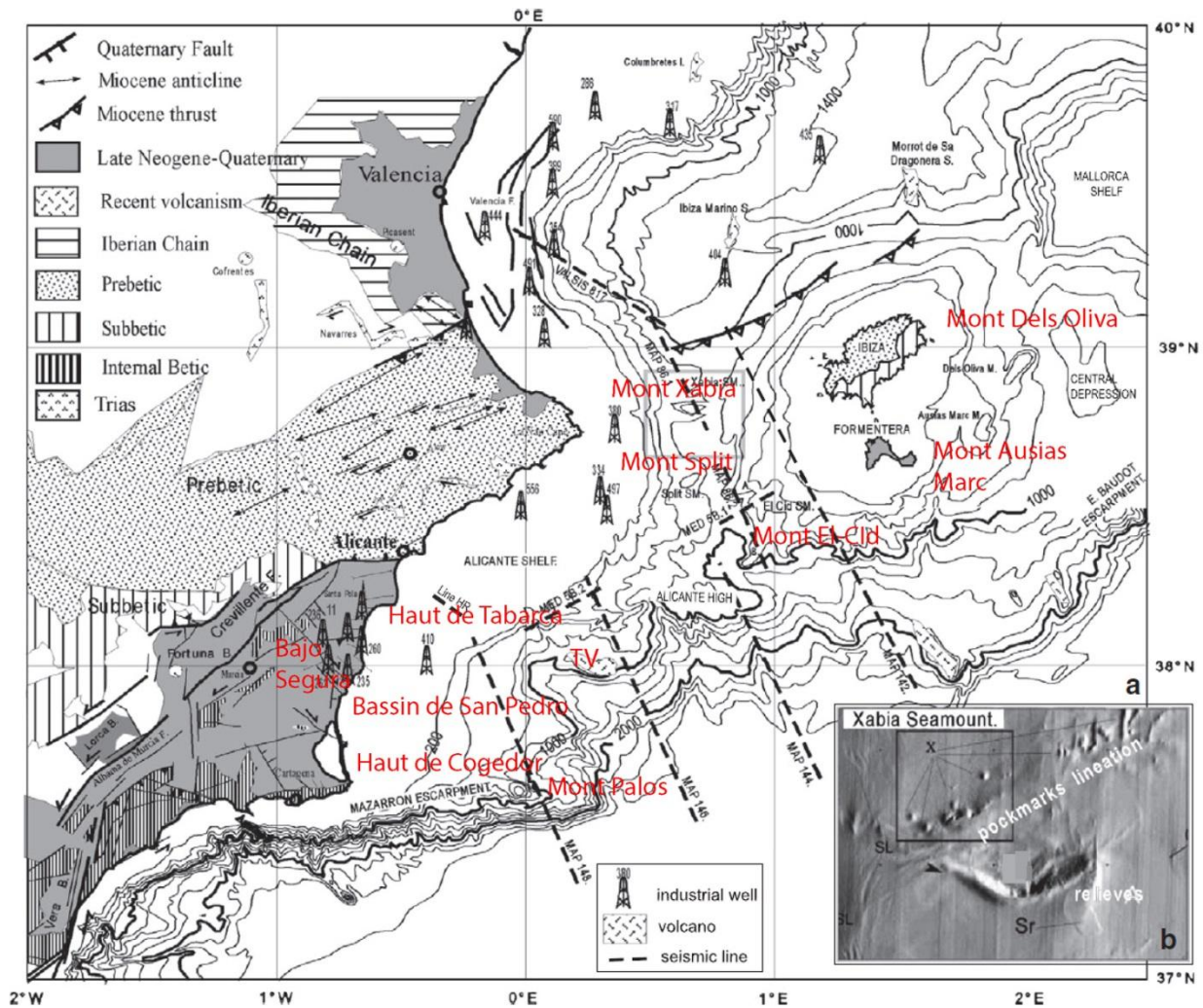
Figure I. 20: Carte bathymétrique du chenal d'Ibiza (Maillard et Mauffret, 2013). Le détail du mont Xabria en haute résolution est d'après Acosta et al. (2002)
