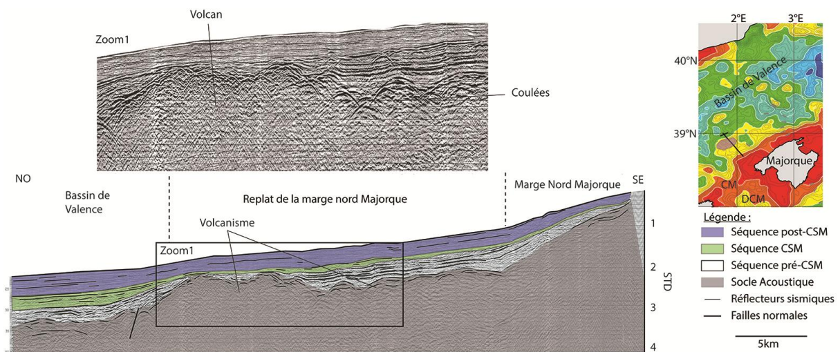
Figure III. 12: Profil de sismique-réflexion Map77-62 situé sur le replat de la marge nord Majorque. Exagération verticale = 2. CM = chenal de Majorque; DCM = dépression centrale de Majorque. CM : Chenal de Majorque ; DCM : Dépression Centrale de Majorque.
