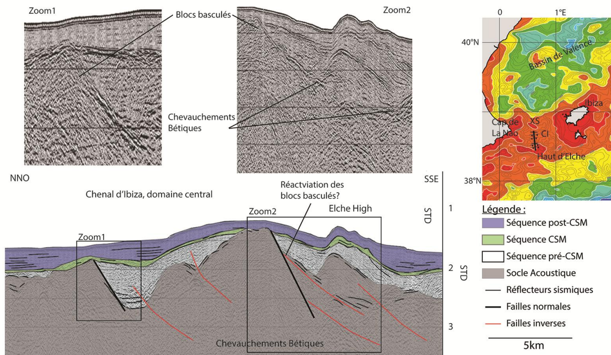
Figure III. 3: Profil de sismique-réflexion Map86 situé dans le chenal d'Ibiza central au niveau de l'extrémité est du haut d'Elche. Exagération verticale = 4. XS : Mont Xabia ; CI : Chenal d'Ibiza
