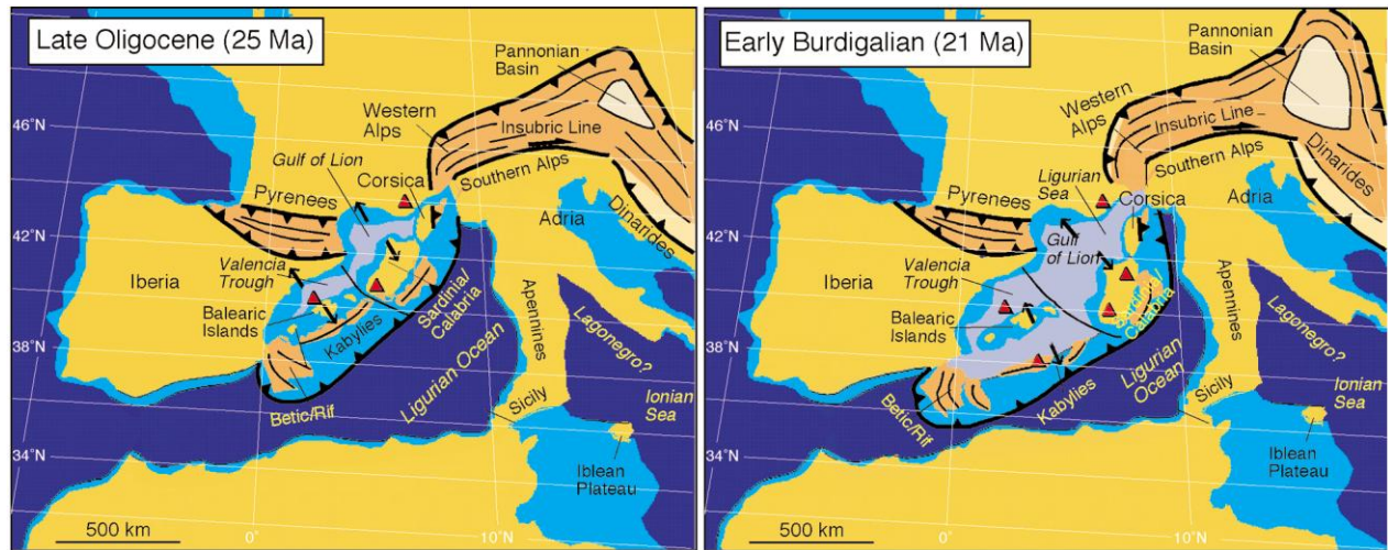
Figure I. 10: La Méditerranée occidentale au Miocène inférieur. (Rosenbaum et al., 2002)
