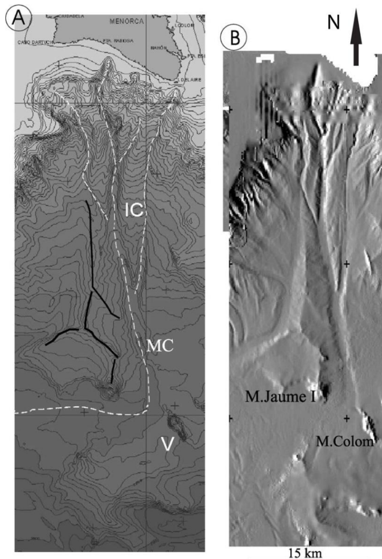
Figure I. 25: Bathymétrie haute résolution de la partie centrale du bloc sud Minorque d'après Acosta et al. (2002). Les trait blanc pointillés marquent le trajet du canyon de Minorque. Les
