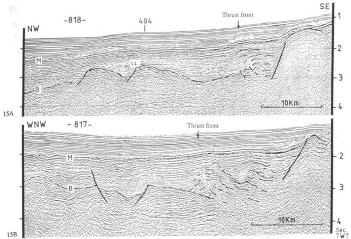
Figure I. 23: Profils de sismique-réflexion montrant les chevauchements Bétiques au pied de la marge nord-Baléares (Maillard et al., 1992). La localisation des profils est indiquée sur la figure I.19.
