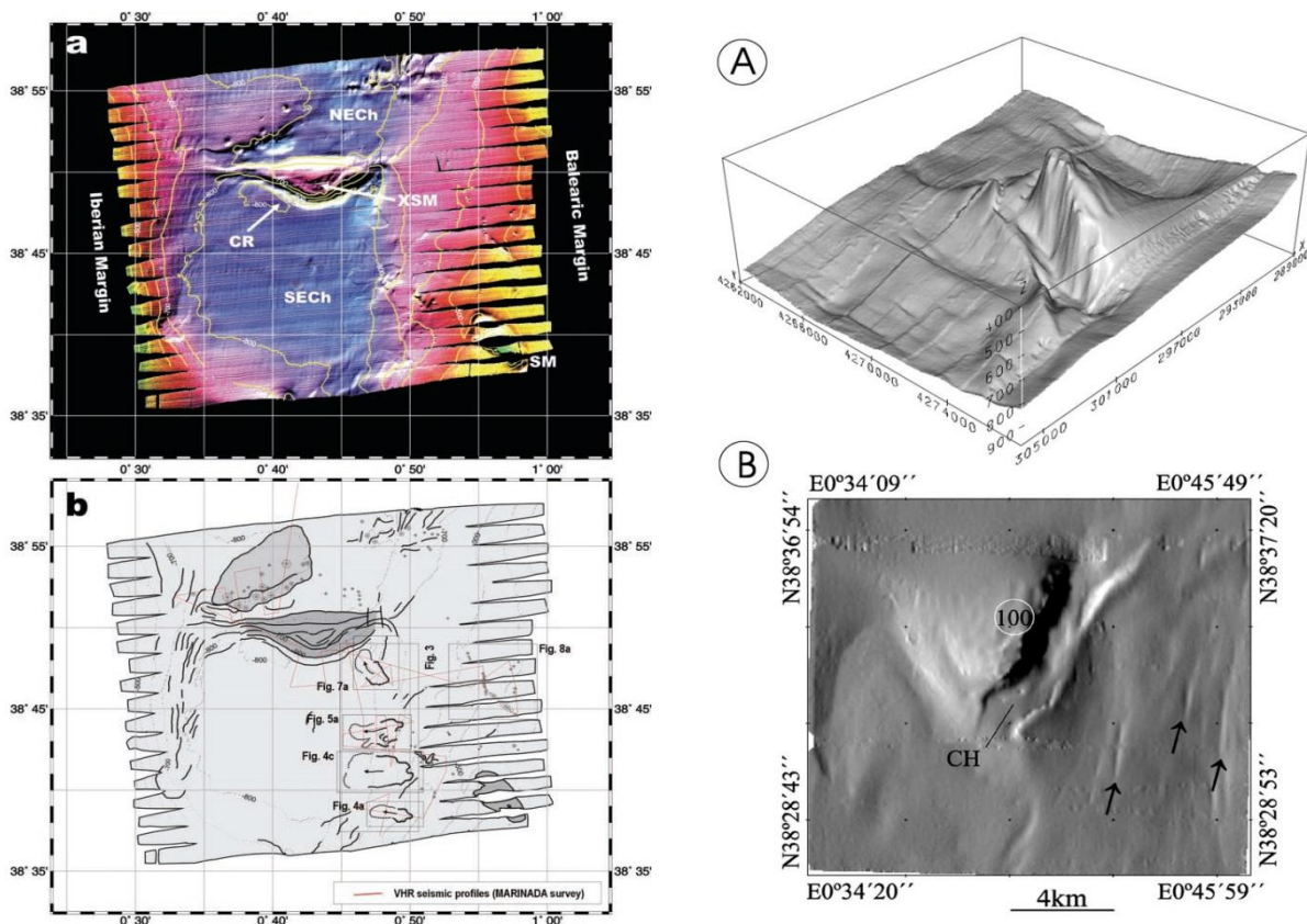
Figure I. 39: Détail des deux monts majeurs du chenal d'Ibiza. A gauche, le Xabia Seamount situé au centre du chenal et formant une structure lenticulaire d'axe E-O et différents glissement de terrain affectant la pente continentale d'Ibiza (Lastras et al., 2004). A droite, le Split Seamount situé au sud du chenal, à la limite du bassin de San Pedro (Acosta et al., 2002).
