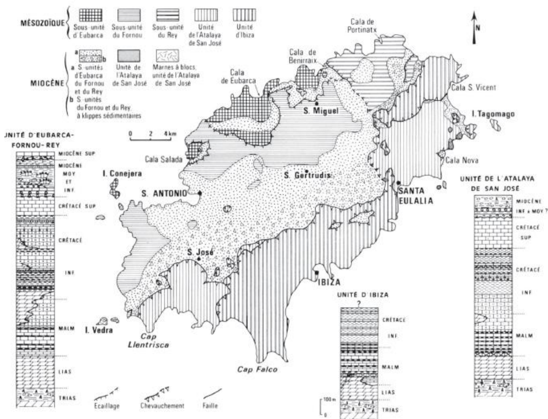
Figure I. 31: Carte géologique de l'île d'Ibiza et les différents log stratigraphiques correspondant aux unités de l'île, d'après Fourcade et al. (1982).
