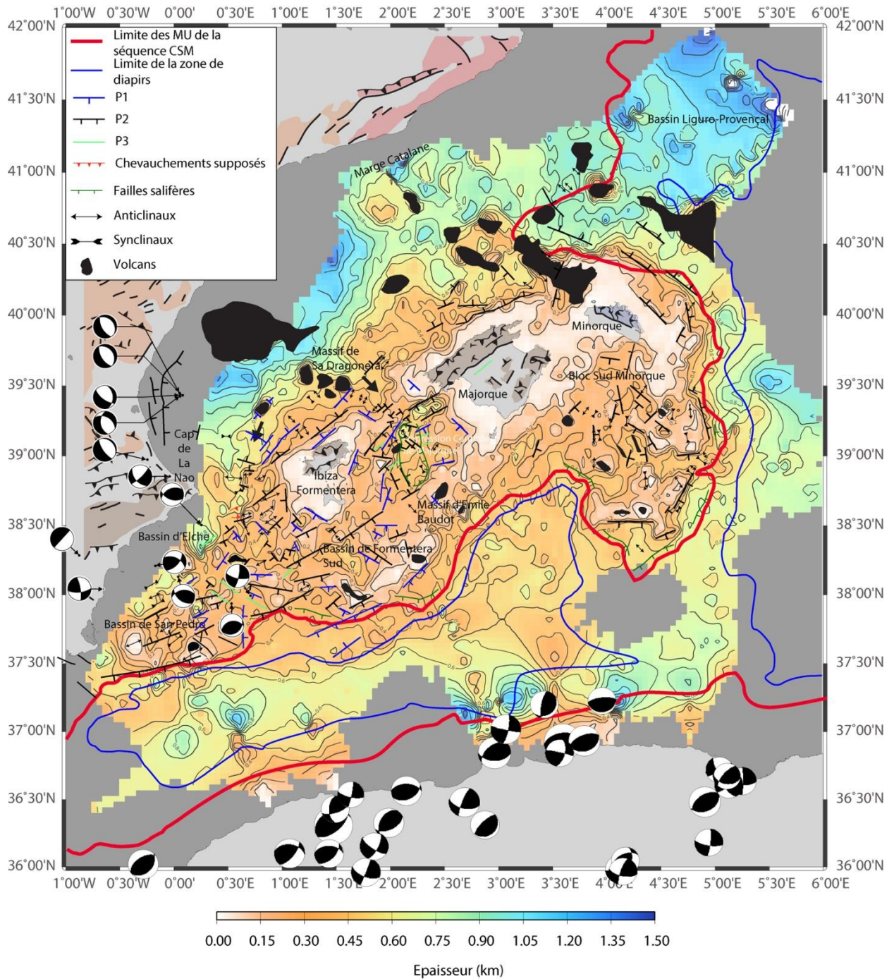
Figure V. 21 : Carte structurale synthétisant l'ensemble des observations réalisées en sismique réflexion. Le fond de carte représente les isopaques de la séquence post-CSM. Les mécanismes au foyer sont modifiés d'après Serpelonni et al. (2007).
