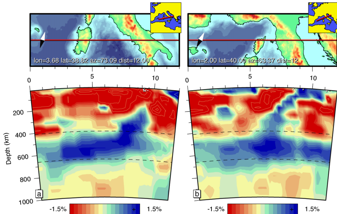
Figure I. 17: Données de tomographie montrant la présence d'un corps froid sous l'Italie, interprété comme les vestiges du slab téthysien. En A, les données montrent une déchirure du slab dans sa partie supérieure. Dans les deux cas, on remarque que le slab a atteint la limite des 670km et à tendance à s'horizontaliser (Spakman et Wortel, 2004).
