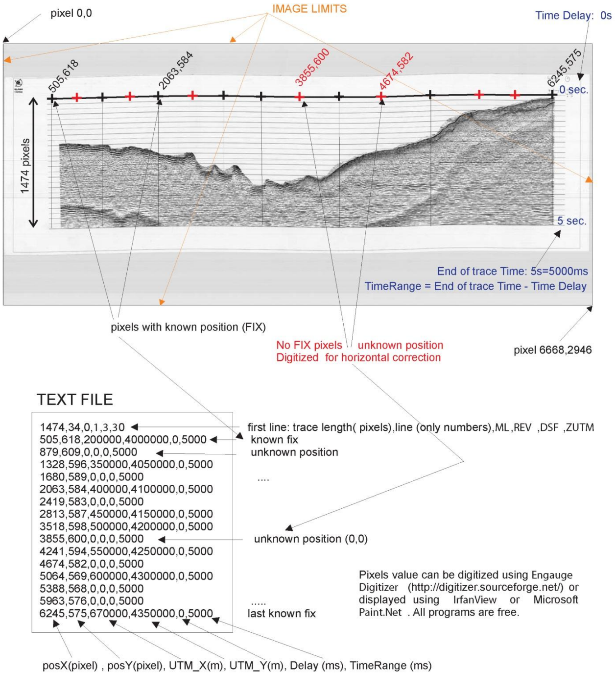
Figure II. 3: Synthèse du processus de segysation d'après Farràn (2008).
