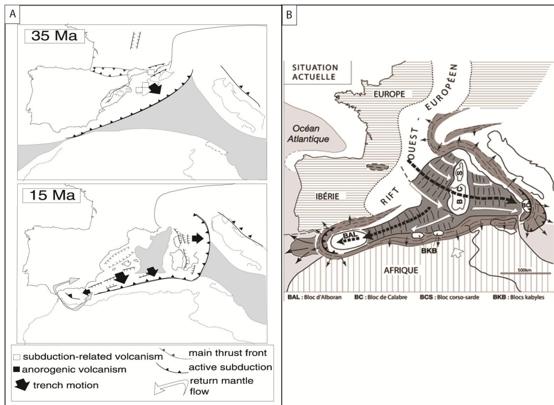
Figure 0. 2 : Exemples de modèles géodynamiques expliquant l'ouverture des bassins de la Méditerranée occidentale. A. Modèle d'ouverture en NO-SE, Faccenna et al. (2004) ; Modèle d'ouverture E-O, Mattauer, 2007.
