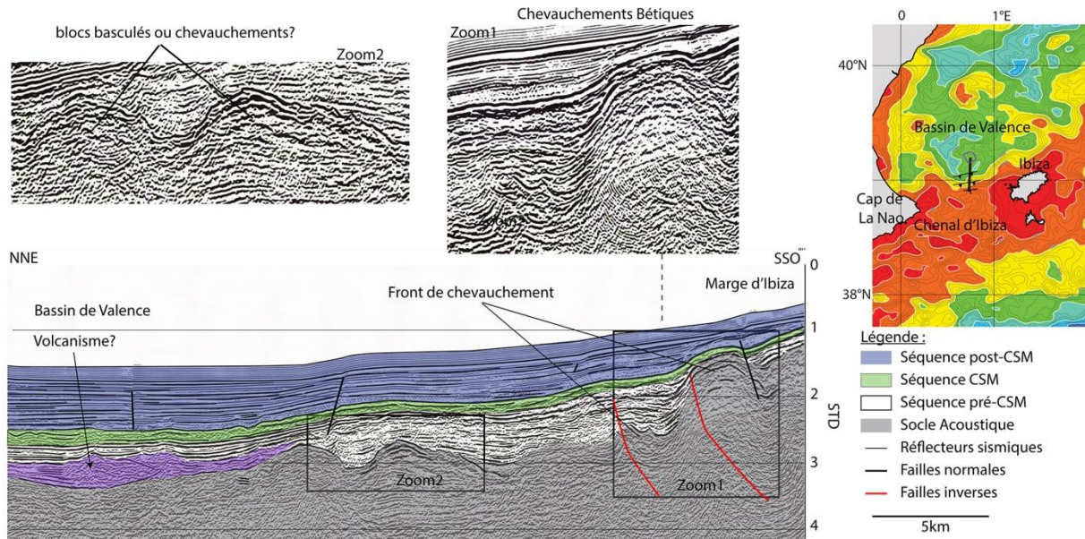
Figure III. 4: Profil de sismique-réflexion Valsis2-818 localisé sur la marge nord Ibiza. Exagération verticale = 2
