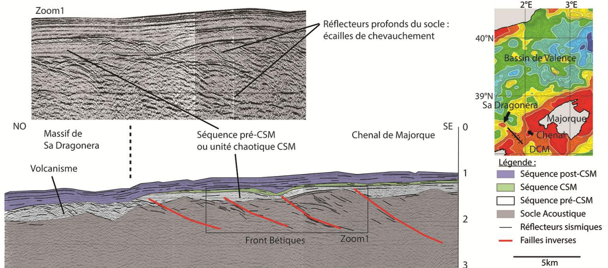
Figure III. 10: Profil de sismique-réflexion Map77-72 situé sur la bordure ouest du chenal de Majorque. Exagération verticale = 2. CM : Chenal de Majorque ; DCM : Dépression Centrale de Majorque
