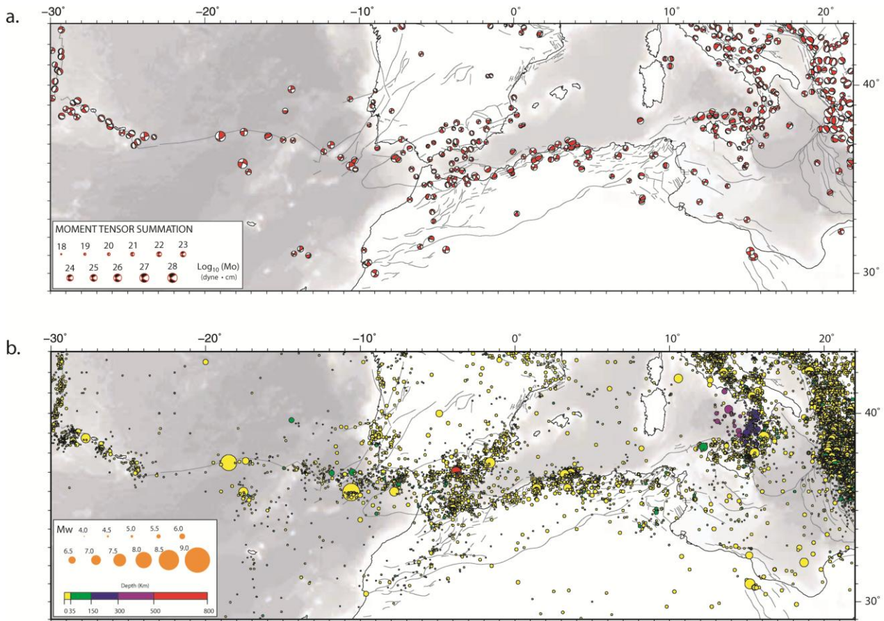
Figure I. 5: Mécanismes au foyer et carte de sismicité de la région ouest méditerranéenne (Serpeloni et al., 2007)
