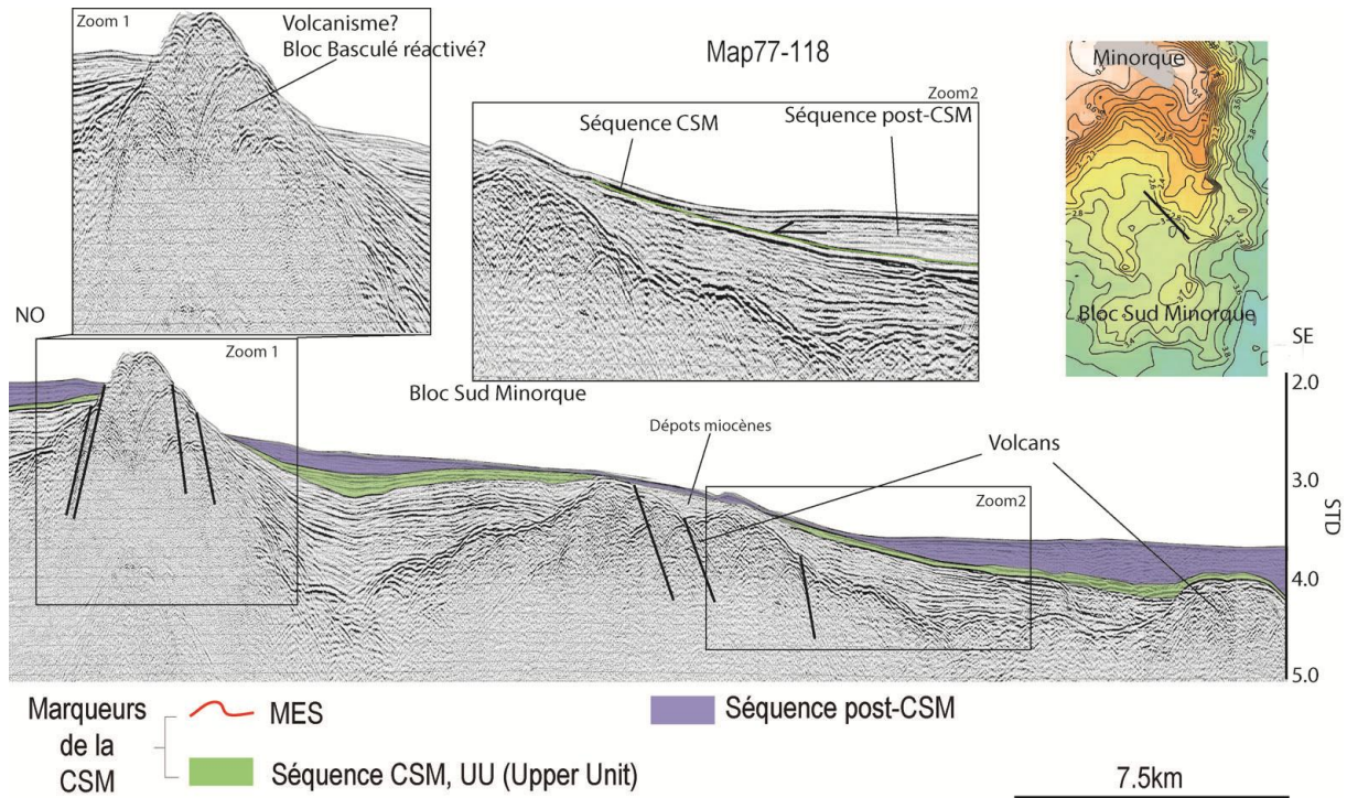
Figure V. 5 : Profil sismique Map77-118 situé sur le bloc sud-Minorque. La position du profil est indiquée dans le coin haut gauche sur la carte des isobathes de la base du Pliocène.
