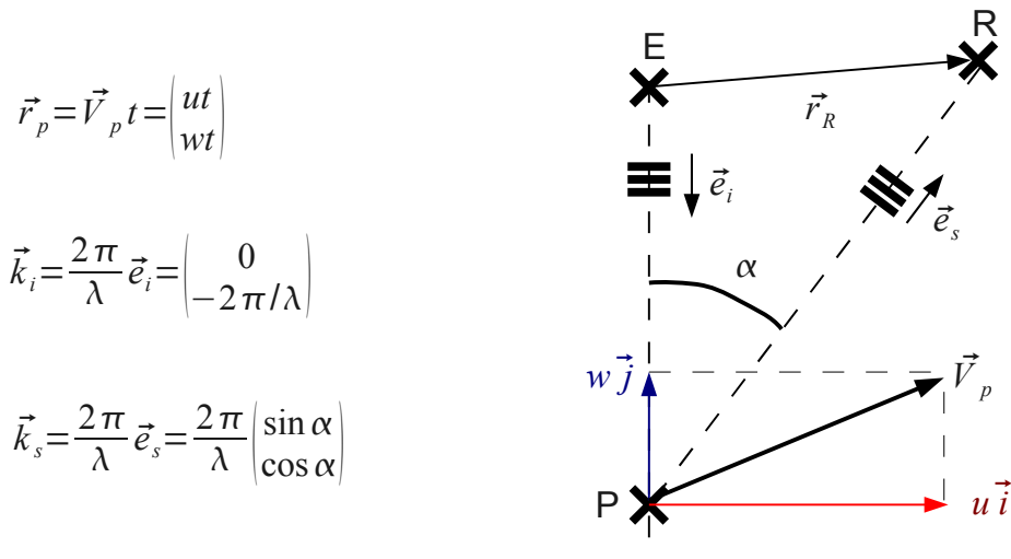
FIGURE 3.9 – Schéma de fonctionnement de la mesure de vitesse par les profilers acoustiques (photocopie du cours Flow Measurement Science , D. Hurther). E représente la céramique émettrice, P une particule (ou rétro-diffuseur) voyageant à la vitesse \vec{V}_p et R un des récepteurs. \lambda = cf_0 représente la longueur d’onde du train d’onde pulsé.
