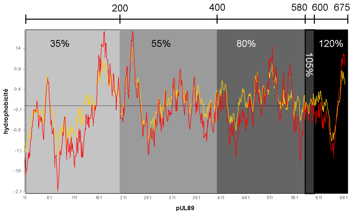
Figure 43: Résultats des affinités relatives pour pUL56 de fragments de pUL89 fusionnés à la GST. Adapté de Thoma et al. 2006. La séquence de pUL89 est représentée en fonction du profil d'hydrophobicité selon les échelles de Kyte & Doolittle et Eisenberg, en rouge et jaune respectivement. L'affinité exprimée en % de chaque portion est normalisée par rapport à pUL89 entier et symbolisée en dégradé de gris. L'affinité de la GST pour pUL56 est de l'ordre de 20%.
