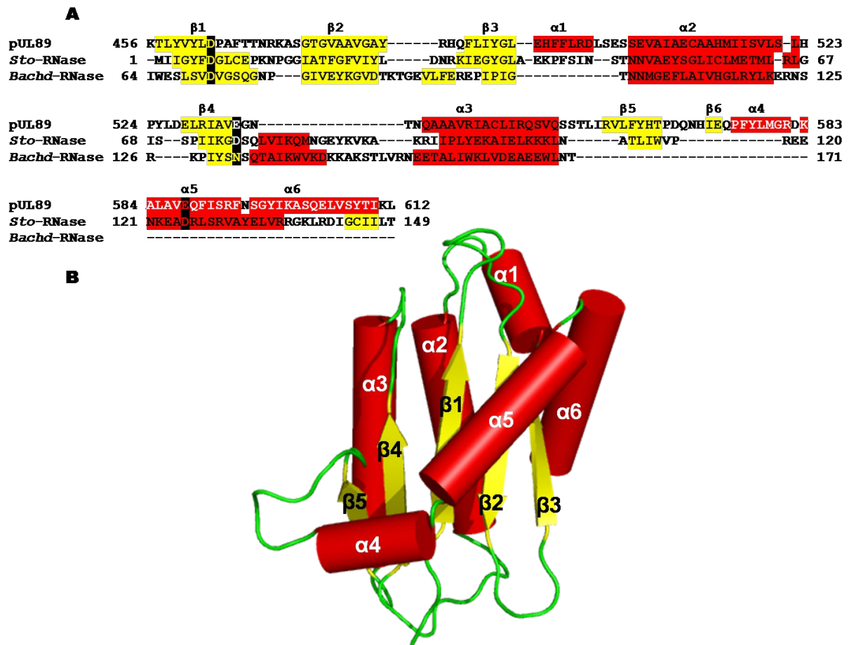
Figure 54: Construction du modèle pUL89-endo par MODELLER. A. Alignement de séquences entre pUL89-endo avec Sto -RNase (2EHG, chaîne A, fragment 1-149) et Bachd -RNase (1ZBI, chaîne A, fragment 64-171). Les brins \beta et hélices \alpha prédits pour pUL89-endo et observés expérimentalement pour les structure-supports sont colorés en jaune et rouge, respectivement. Les hélices observées en RMN sont représentées avec des lettres blanches et imposées comme contraintes. Les résidus catalytiques alignés sont encadrés en noir. B. Modèle de pUL89-endo sans le duplexe ARN/ADN issu de l'alignement de A. L'annotation des éléments de structures secondaires se réfère à celle utilisée en A.
