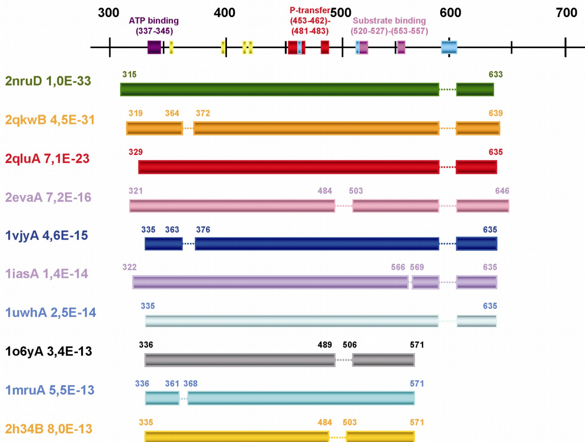
Figure 71: Modèles générés par PHYRE sur le mutant de délétion pUL97 \Delta (590-607). Même légende que précédemment. Les pointillés dans la zone 590-607 traduisent la délétion souhaitée qui n'est donc pas un artefact de reconstruction.
