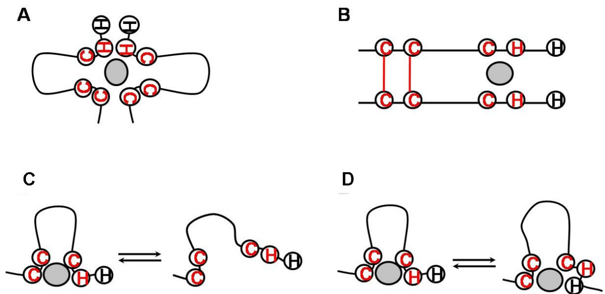
Figure 61: Cas expliquant une déstabilisation du signal observé en UV/visible au-delà de 0,5 équivalents. Le disque gris schématise l'atome de zinc, les résidus conservés (Cys 191 , Cys 194 , Cys 217 , His 219 ) sont annotés en rouge et l'histidine non conservée (His 223 ) en noir. A et B montrent la possibilité de dimérisation à travers la chélation du zinc. C et D illustrent des échanges conformationnels entre deux formes.
