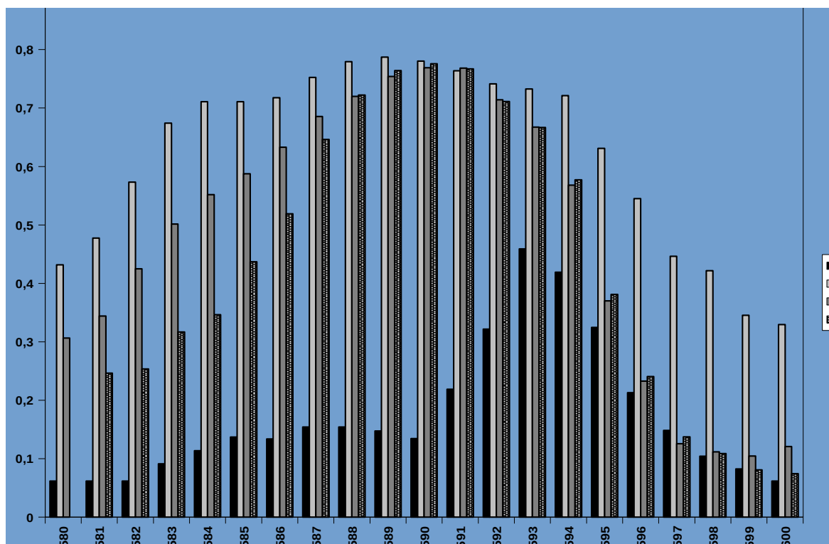
Figure 46: Calcul du paramètre d'ordre ( S^2 ) pour chaque acide aminé le long de la séquence de pUL89(580-600). L'estimation a été faite sur le serveur http://wishart.biology.ualberta.ca/rci . en prenant en compte les déplacements chimiques H\alpha , H\beta et NH . La structure dans l'eau est peu stable alors que dans le TFE et le DPC elle est très ordonnée entre Ala 584 et Phe 595 , principalement.
