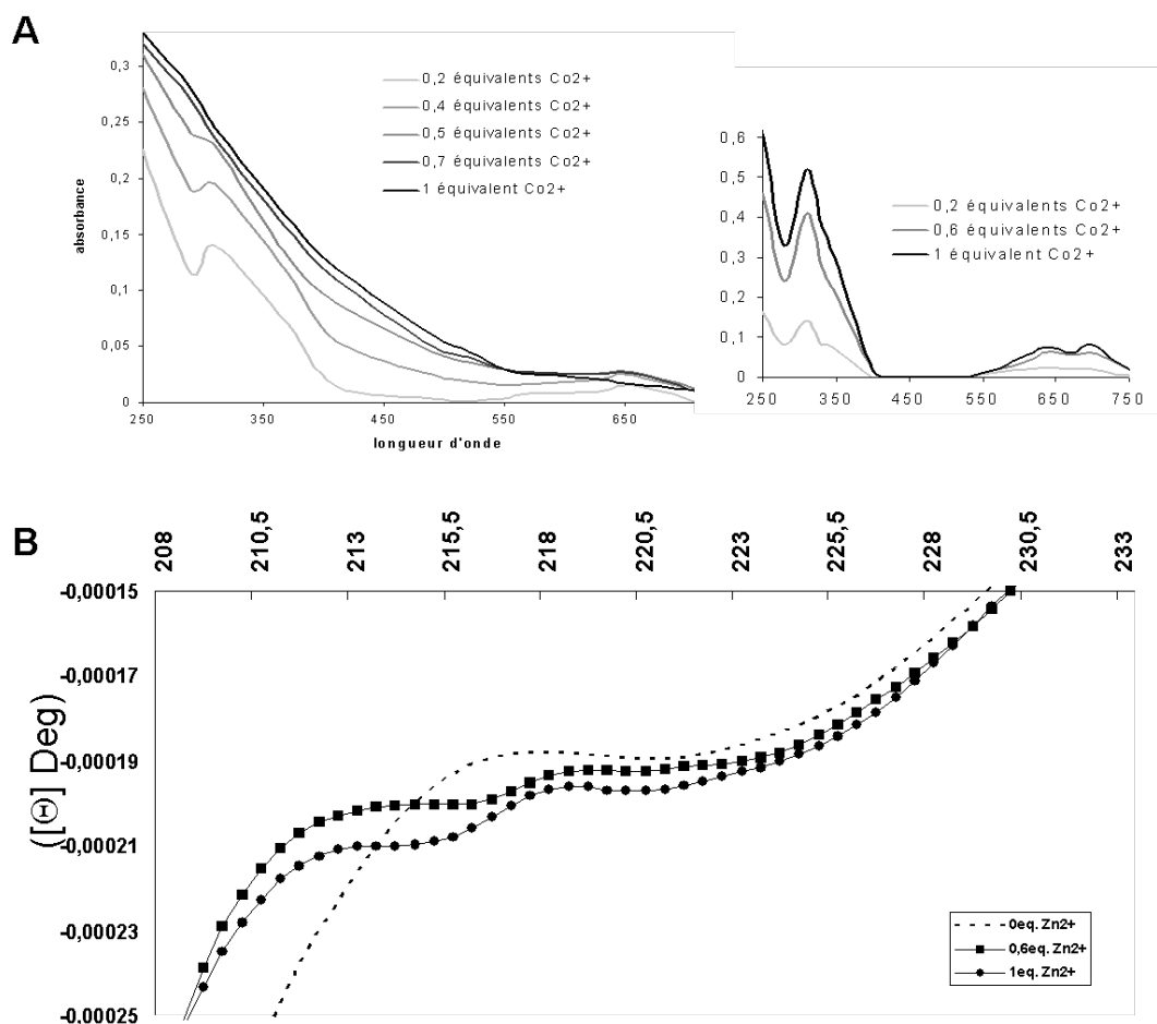
Figure 60: Analyse de pUL56-ZF par spectroscopie UV/visible et dichroïsme circulaire. A. Une solution de 150 \mu M de pUL56-ZF en tampon phosphate 7,5 et en présence de DTT a été incrémenté en CoCl_2 (gauche). La même expérience avec Ncp7(1-30) du VIH a été effectuée (droite) pour valider notre protocole expérimentale. B. Zoom des courbes de dichroïsme circulaire dans la région 208-235nm obtenu pour puL56-ZF incrémenté en ZnCl_2 . Les courbes obtenues pour 0, 0,6 et 1 équivalent sont représentées en pointillés, carrés et disques noirs, respectivement.
