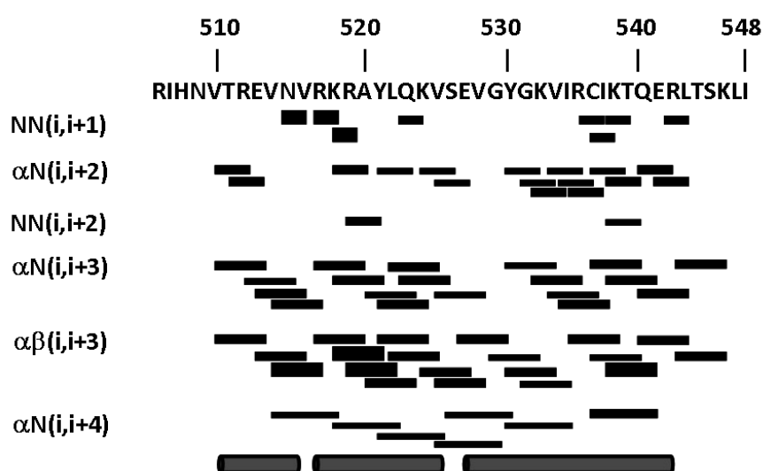
Figure 67: Table de connectivités des NOEs recueillies pour la modélisation du dimère de pUL56(506-548).
