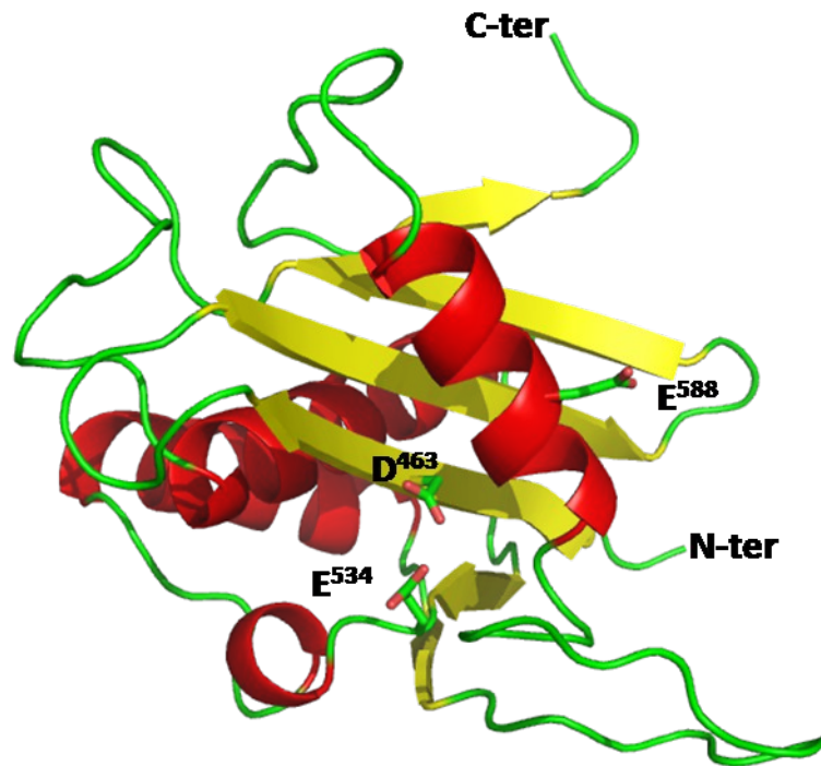
Figure 53: Modèle de pUL89-endo calculé par MUSTER à partir de la structure PDB de la ribonucléase H de type 1 de Solfobus Tokodaii (2EHG). Le squelette est coloré en fonction des éléments de structure secondaires (brins \beta jaunes et hélices \alpha rouges). Les chaînes latérales d'Asp 463 , Glu 534 et Glu 588 sont représentées en sticks et font apparaître un positionnement entre elles favorables à la formation d'une poche de liaison à un ou plusieurs métaux.
