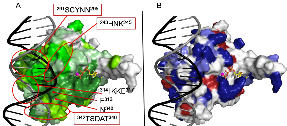
Figure 41: Répartition du taux de conservation et des caractères physicochimiques à l'interface avec le duplexe d'ADN. A. Le taux de conservation est codifié par nuance de vert. Les résidus dont les atomes lourds sont situés à moins de 5Å du duplexe y sont précisés. Ils sont principalement inclus dans les boucles Ia, Ic, IIa et III. B. Même vue qu'en A. Les positivement (H, K et R), négativement chargés (D et E), glutamines et asparagines, et tous les autres résidus sont colorés en bleu, rouge, bleu clair et blanc respectivement ce qui montre non seulement une bonne conservation des résidus à l'interface avec l'ADN mais aussi un grand nombre d'asparagines et résidus basiques.
