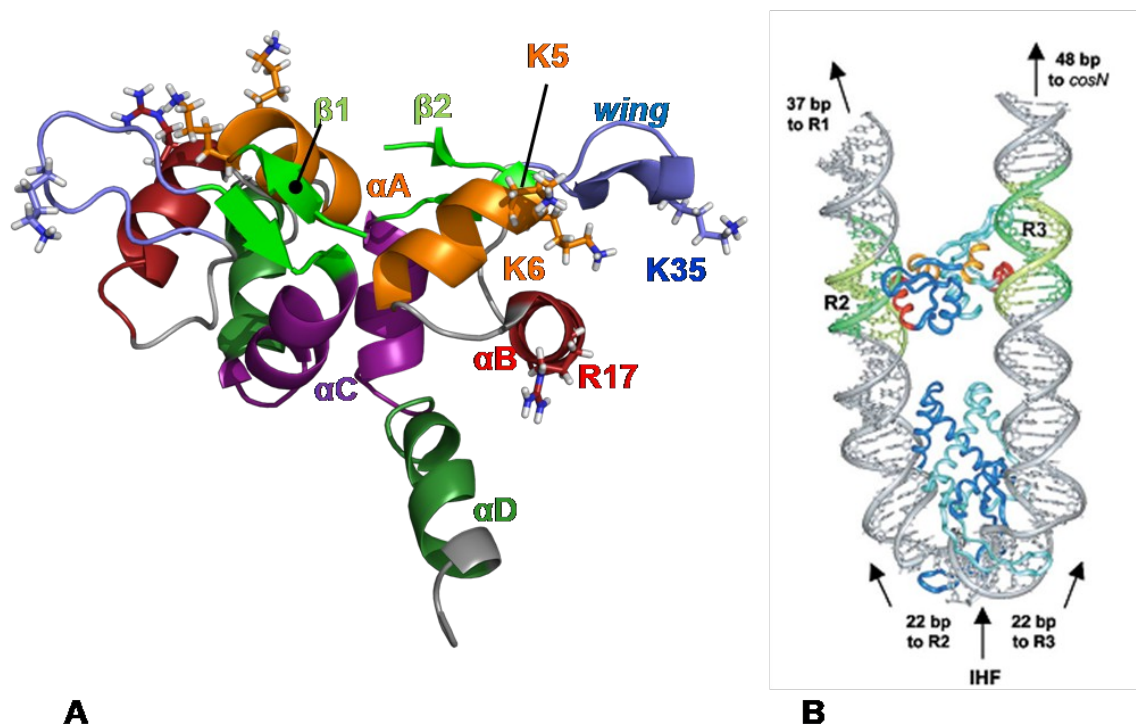
Figure 12: A. Dimère de gpNu1. Représentation des différents éléments de structures secondaires constituant le monomère de gpNu1: hélice \alpha A (AA 5-12) en orange, hélice \alpha B (AA 16-25) en rouge, hélice \alpha C (AA 43-53) en violet, hélice \alpha D (AA 53-60) en vert foncé, brins \beta 1 (1-4) et \beta 2 (40-43) en vert clair et domaine wing (AA 31-39) en bleu. La dimérisation se fait via des résidus aliphatiques des hélices \alpha A et \alpha C . Les résidus basiques impliqués dans la reconnaissance de l'ADN sont étiquetés et représentés en bâtons. Notons la présence de la lysine 35 située sur le domaine wing qui se loge dans le petit sillon de l'ADN. B. Modèle de la reconnaissance de l'ADN par le dimère de gpNu1. Grâce à l'intervention de la protéine de l'hôte Integration Host Factor qui va courber l'ADN viral au niveau de la séquence médiane entre R2 et R3, gpNu1 va reconnaître simultanément R2 et R3 en mettant en jeu un monomère pour chaque séquence.
