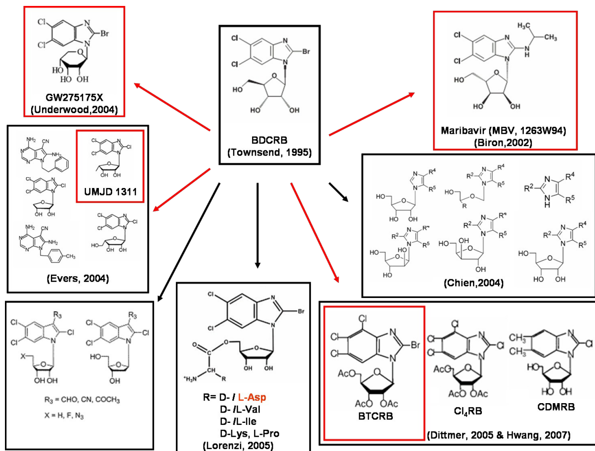
Figure 24: Dérivés des 2,5,6-trihalo-1-(bêta-D-ribofuranosyl)benzimidazoles: du BDCRB au BTCRB. En rouge sont représentées les molécules ayant manifestées une activité pharmacologique.
