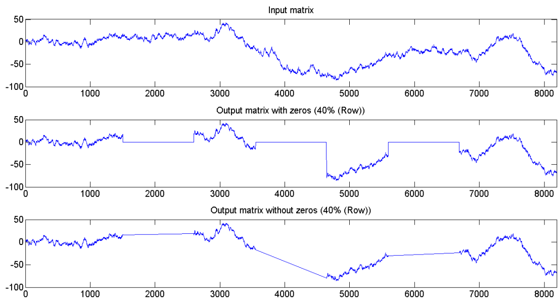
Figure 4-7. Visualisation du mouvement brownien avec 40% de dégradation du signal réparti entre 3 périodes consécutives. En haut : mouvement brownien non dégradé. Au milieu : période manquante remplacée par des zéros. En bas : périodes manquantes.
