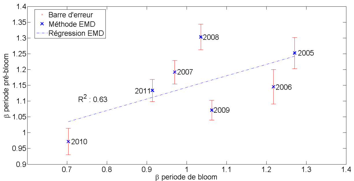
Figure 2-33. Pentés spectrales pré-bloom en fonction des pentés spectrales durant la période de bloom. Les pentés spectrales sont calculées avec la méthode EMD-HSA (p-value = 0,76).
