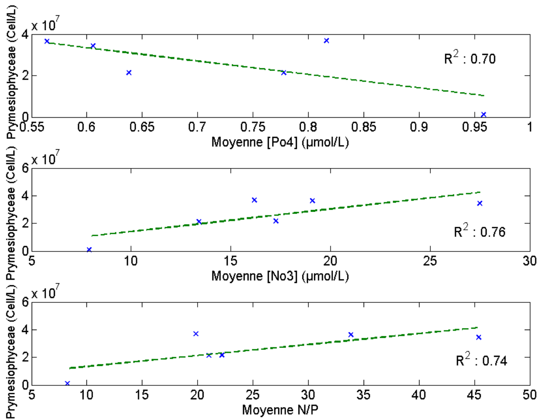
Figure 2-31. En haut : relation entre les moyennes annuelles de phosphates MAREL Carnot et les concentrations cellulaires de pymesiophycées (p-value = 0,12). Au milieu : relation entre les moyennes annuelles de nitrates MAREL Carnot et les concentrations cellulaires de pymesiophycées (p-value = 0,14). En bas : relation entre les moyennes annuelles du rapport N/P et les concentrations cellulaires de pymesiophycées (p-value = 0,43).
