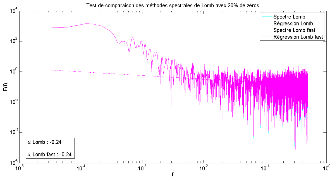
Figure 4-33. Comparaison des méthodes de Lomb classique (en cyan) et Fast Lomb (en magenta), réalisées sur un mouvement brownien dégradé avec 20% de zéros répartis de manière aléatoire.
