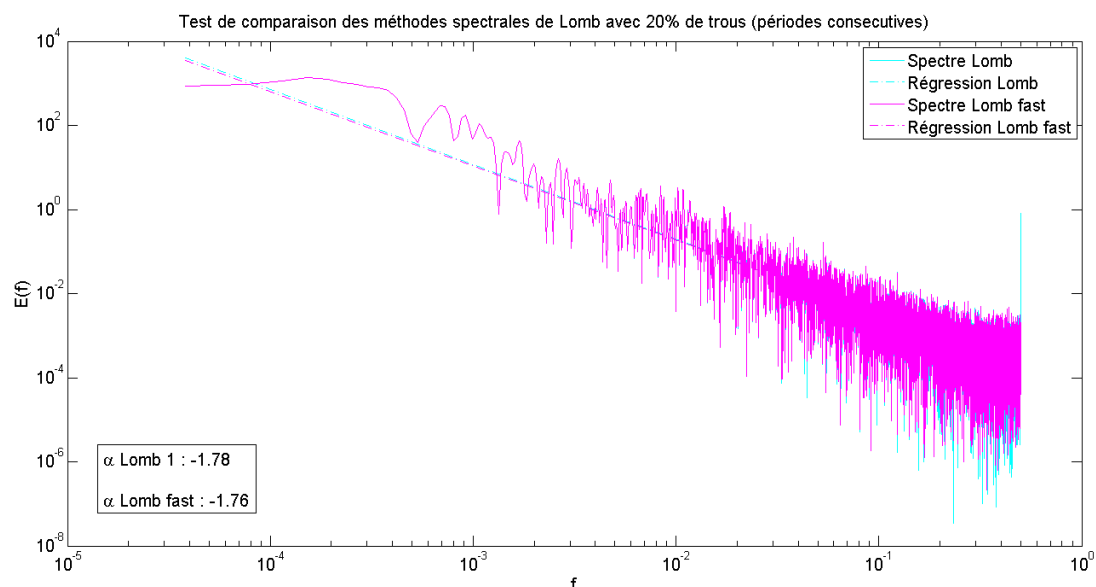
Figure 4-21. Comparaison des méthodes de Lomb classique (en cyan) et Fast Lomb (en magenta), réalisées sur un mouvement brownien dégradé avec 20% de périodes manquante réparties de manière consécutive.
