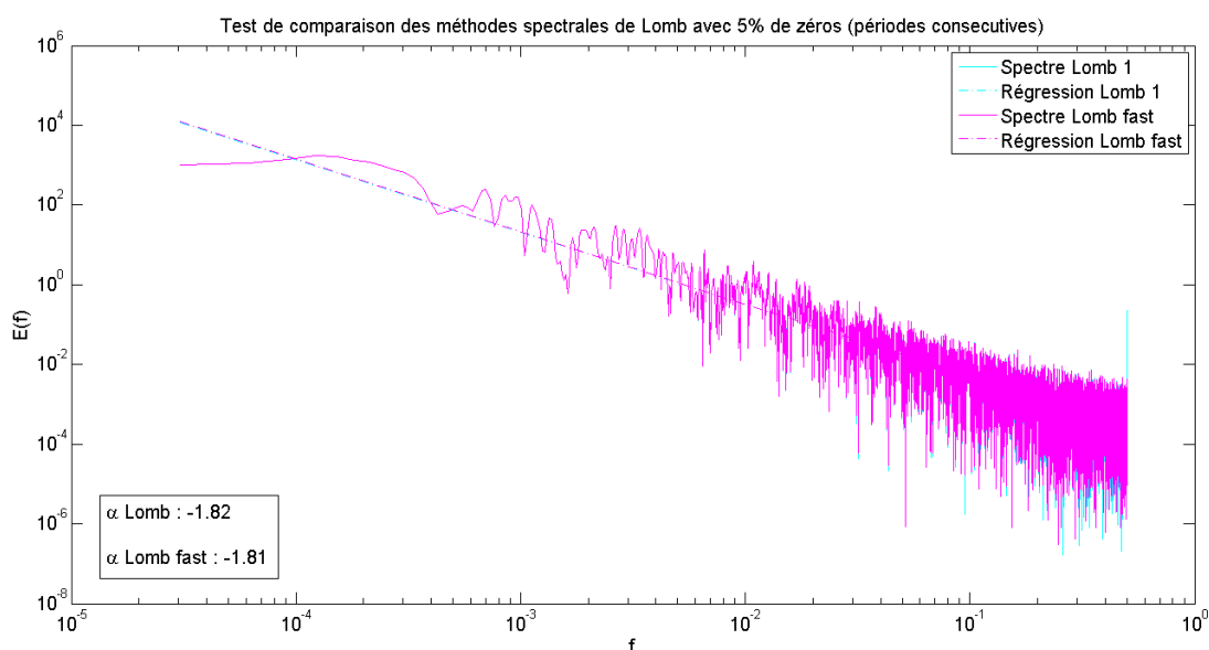
Figure 4-9. Comparaison des méthodes de Lomb classique (en cyan) et Fast Lomb (en magenta), réalisées sur un mouvement brownien dégradé avec 5% de zéros répartis de manière consécutive.
