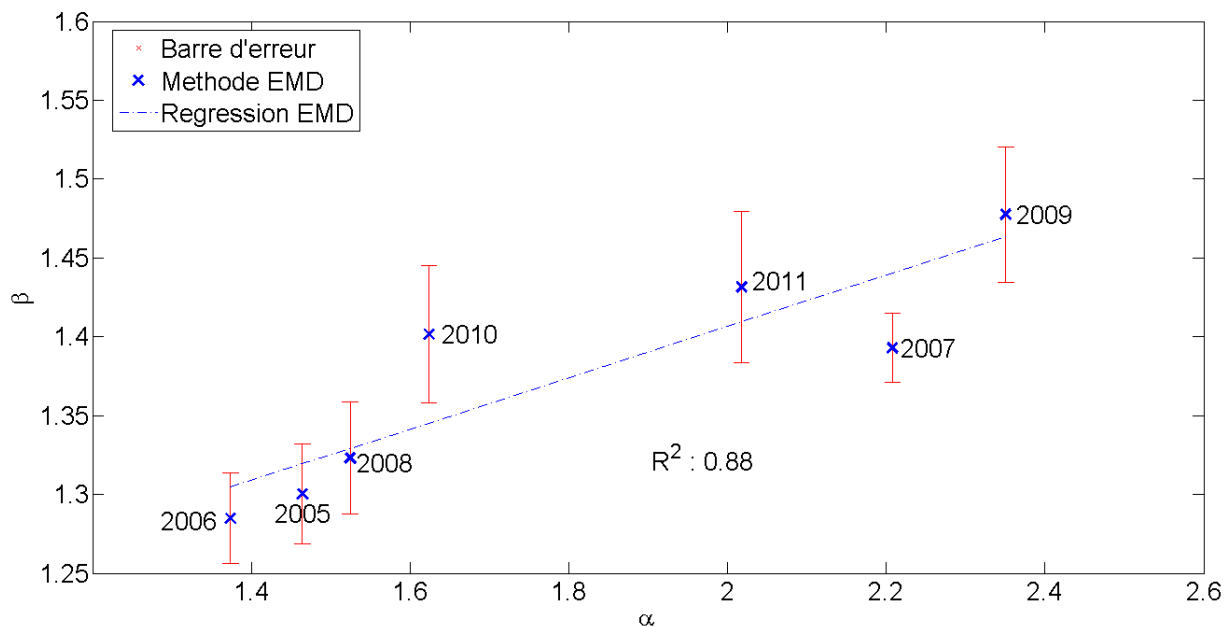
Figure 2-34. Pentes spectrales ( \beta ) issues des hivers météorologiques en fonction des coefficients \alpha issus des PDF de fluorescence.
