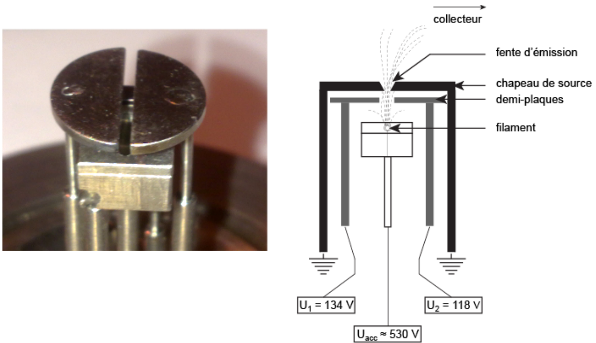
Figure II.59 : Vue générale d'une source similaire à celle opérant dans le spectromètre de masse et schéma montrant la position des différents éléments la composant et leur potentiel électrique.
