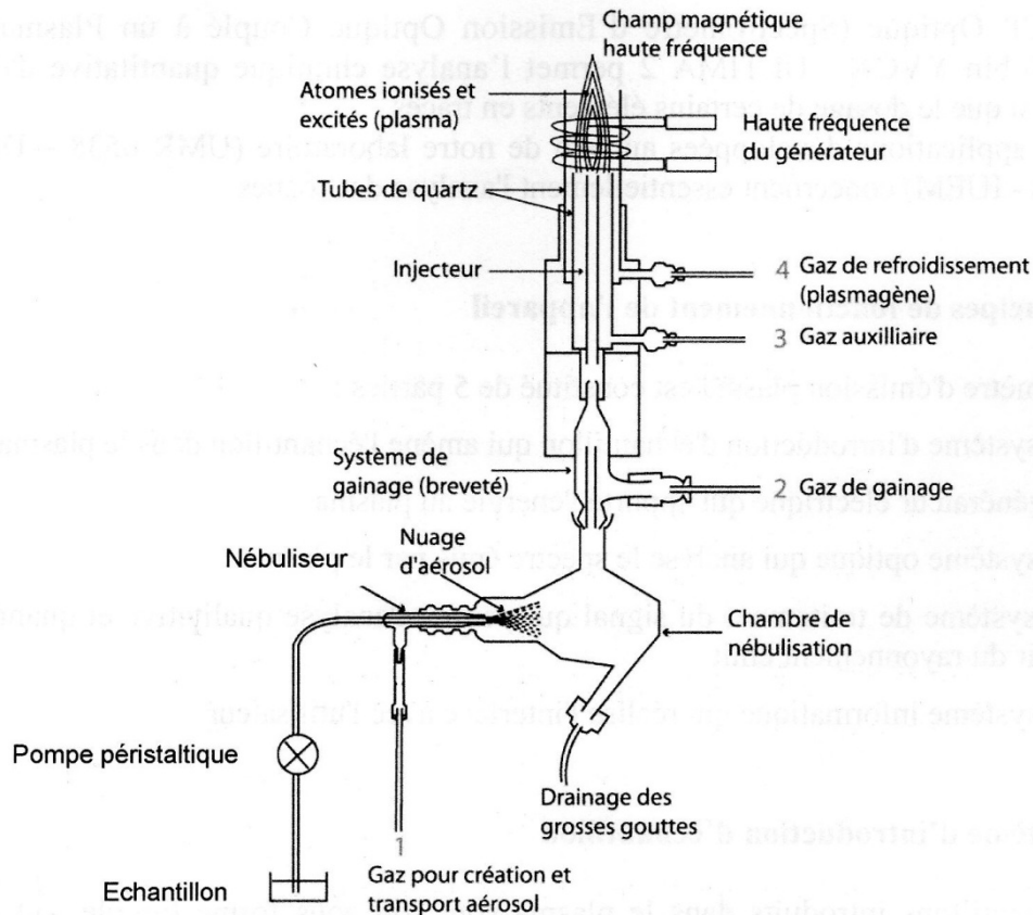
Figure II.68 : Schéma de principe du système de nébulisation et d'introduction de l'échantillon dans la torche à plasma de l'ICP optique Horiba Jobin YVON / Ultima 2.
