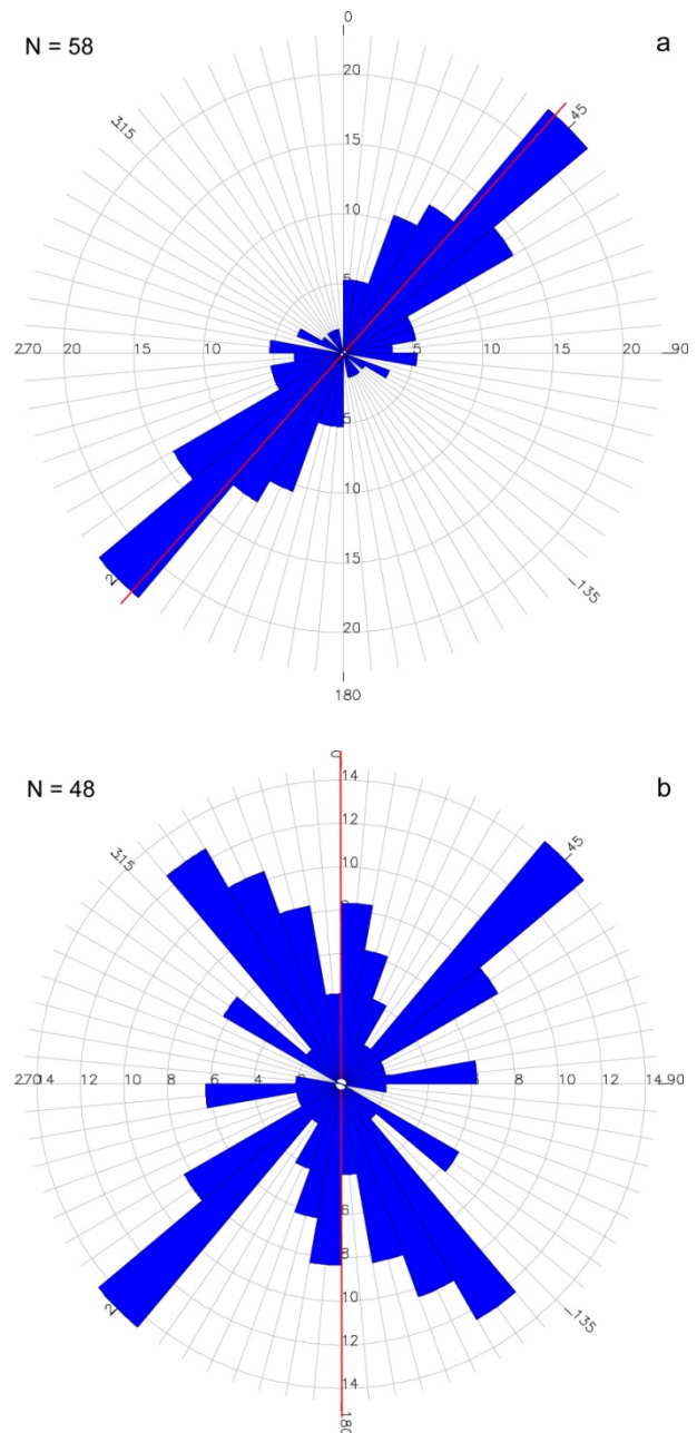
Figure II.42 : rose diagrams représentant les orientations des dykes mesurés dans les séries d'Ayosa (a) et de Cho Marcial (b) le long de la route de la Cordillera Dorsal . Ces diagrammes ont été réalisés respectivement à partir de populations de 58 (a) et 48 (b) dykes. La largeur des « pétales » des deux diagrammes vaut 10°. Les lignes rouges représentent la moyenne de l'orientation de chaque population. Les effectifs de chaque classe sont donnés en pourcent.
