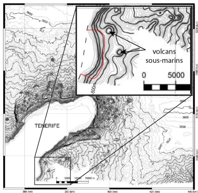
Figure II.30 : Carte bathymétrique de l'extrémité NE de Tenerife (Llanes et al., 2003). La zone correspondant au débouché de la loupe de glissement de Guïmar a été grossie. La ligne rouge souligne le contour du delta de laves formé par le remplissage de la vallée de Guïmar. La ligne en pointillé représente l'interpolation d'un paléotrait de côte entre les extrémités des parois de la loupe du glissement de Guïmar. La première isobathe correspond à une profondeur de 25 m.
