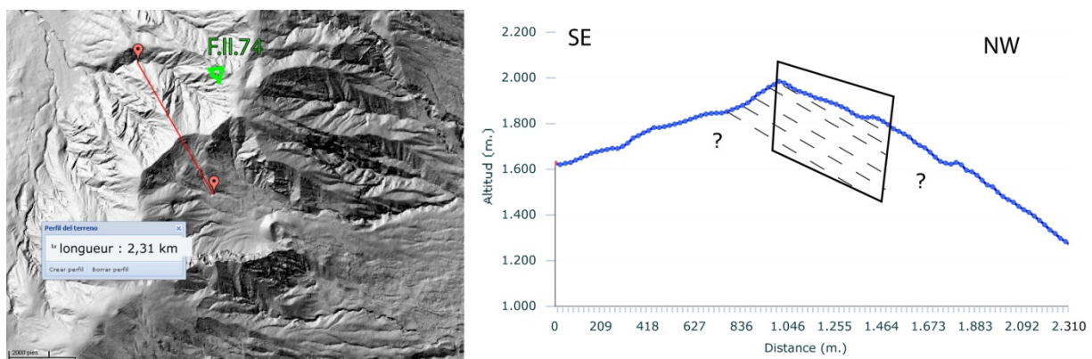
Figure II.37 : Profil topographique du flanc NW de Cho Marcial réalisé le long de la crête située au premier plan de la Figure II.38. Le cadre noir représente approximativement le champ de la photo de la figure. Les pendages de la pile de coulées observées sous la Montaña de Las Cuevitas ont été représentés par les droites en pointillés.
