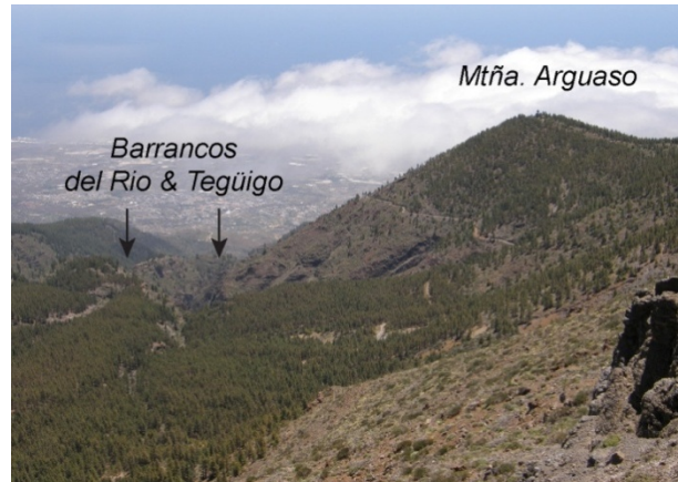
Figure II.25 : vue de la paroi Sud de Guïmar depuis la Montaña Cobre. Le barranco Tegüigo s'incise le long de ce mur entre les unités pré et post-glissement.
