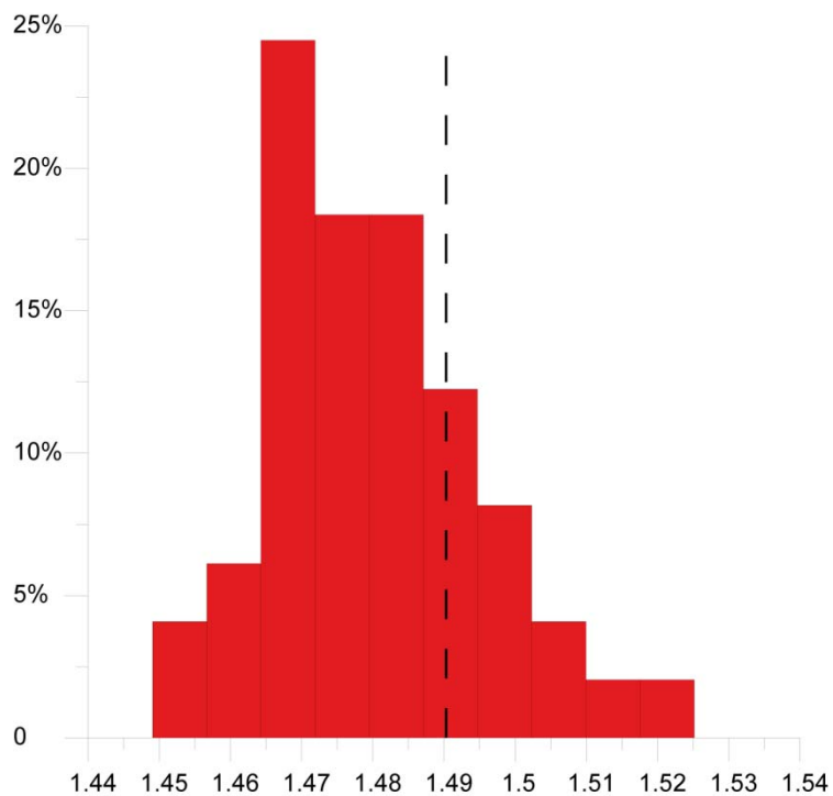
Figure II.56 : Histogramme de la distribution des teneurs en K mesurées pour le géostandard BCR-2 sur 49 séries analytiques réalisées en spectrométrie d'absorption atomique entre mai 2009 et mai 2011. Le trait en pointillé représente la valeur recommandée de K (1,49). Les 49 mesures ont une moyenne de 1.479 et un écart type relatif de 1.03% (i.e : \sigma = 0.015 ). La largeur des classes de l'histogramme du haut de la figure vaut 1\sigma et la classe majoritaire est centrée sur la moyenne, pour l'histogramme du bas, la largeur vaut \sigma/2 .
