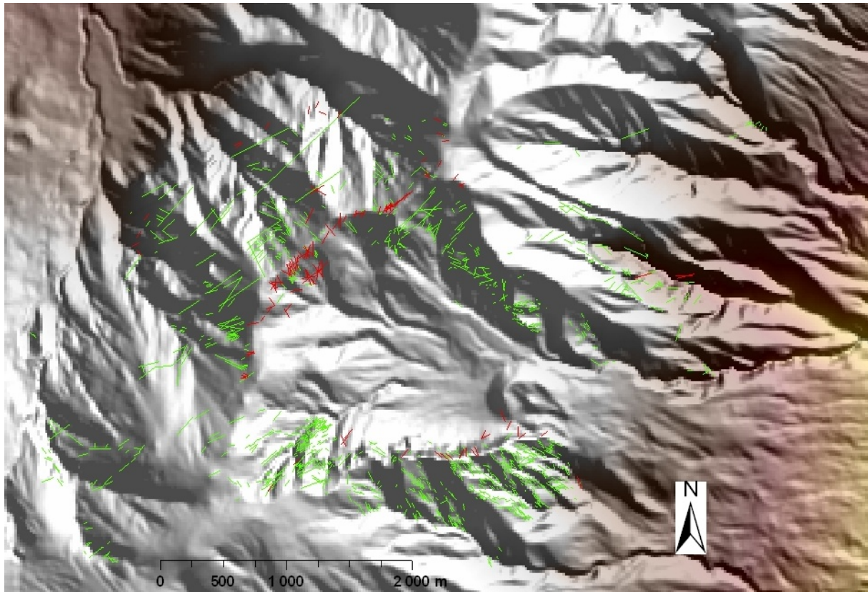
Figure II.44 : Distribution des dykes dans la zone de Cho Marcial. Les linéaments marqués en vert correspondent aux dykes télé-déTECTÉS sur les images de GRAFCAN. Les lignes rouges marquent les dykes mesurés sur le terrain.
