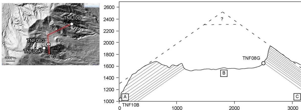
Figure II.35 : Profils topographiques radiaux à travers les flancs S et NE de Cho Marcial . Les pentages des empilements observés dans les parois internes du volcan ont été représentés. Les pointillés représentent le prolongement des pentages des coulées en surface structurale, illustrant une position possible du centre d'émission. L'échelle verticale des profils est de 1.
