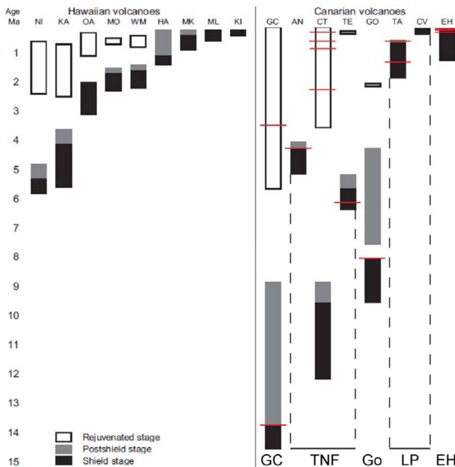
Figure I.2 : Progression des âges des plus anciennes formations datées à travers l'archipel des Canaries selon Guillou et al. (2004).
