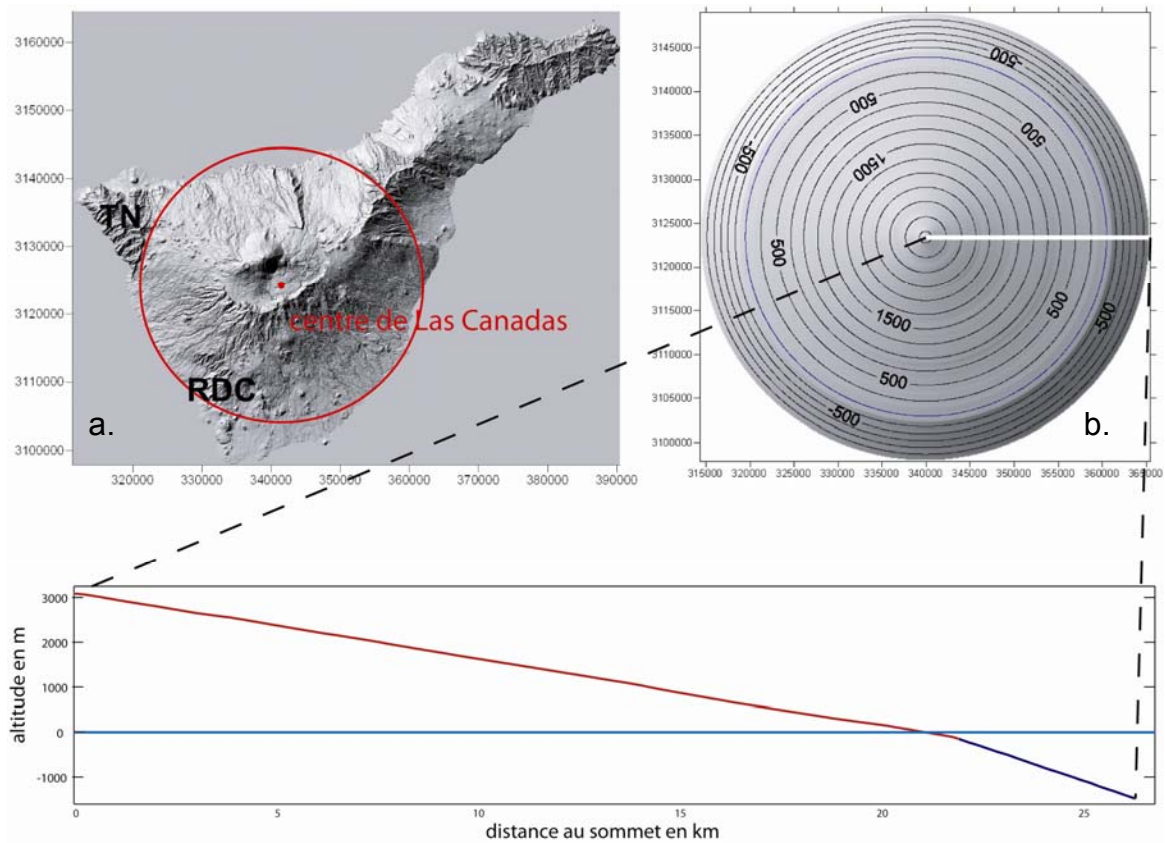
Figure II.86 : Reconstruction morphologique de Las Canadas.
