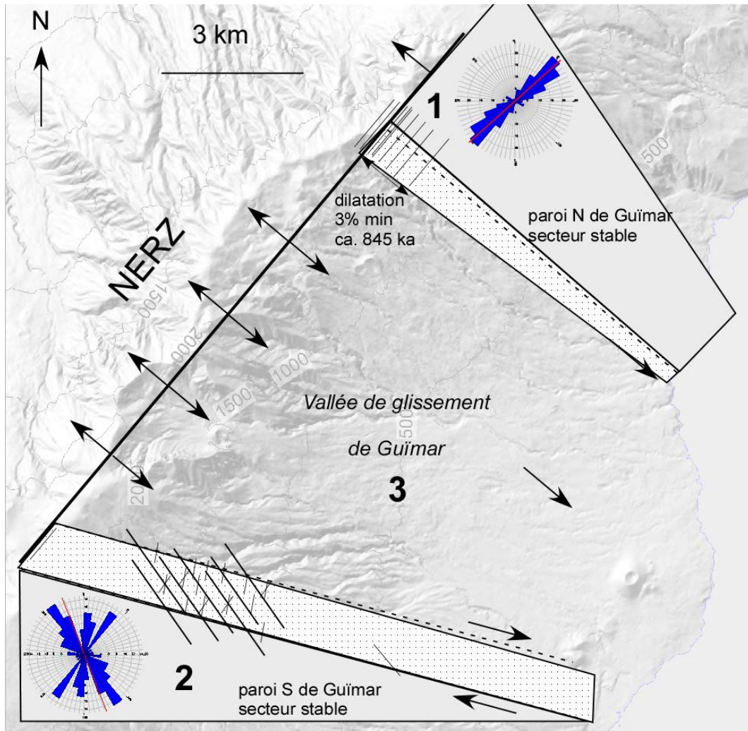
Figure III.2 : schéma structural de la vallée de Guïmar. Un ombrage de la topographie a été inséré pour faciliter la localisation. Les zones en grisé correspondent au flanc de la NERZ non affectés par le glissement de Guïmar. Les zones en pointillés correspondent aux parois de la loupe de glissement. Les lignes représentées dans les parois sont une illustration de la position dykes fictifs orientés selon les directions mesurées sur le terrain.
