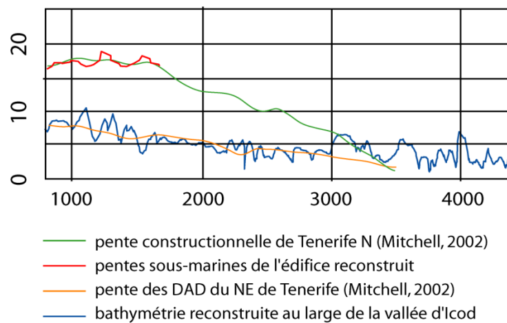
Figure II.88 : Comparatif des profils topographiques du bouclier et de la bathymétrie reconstruits.
