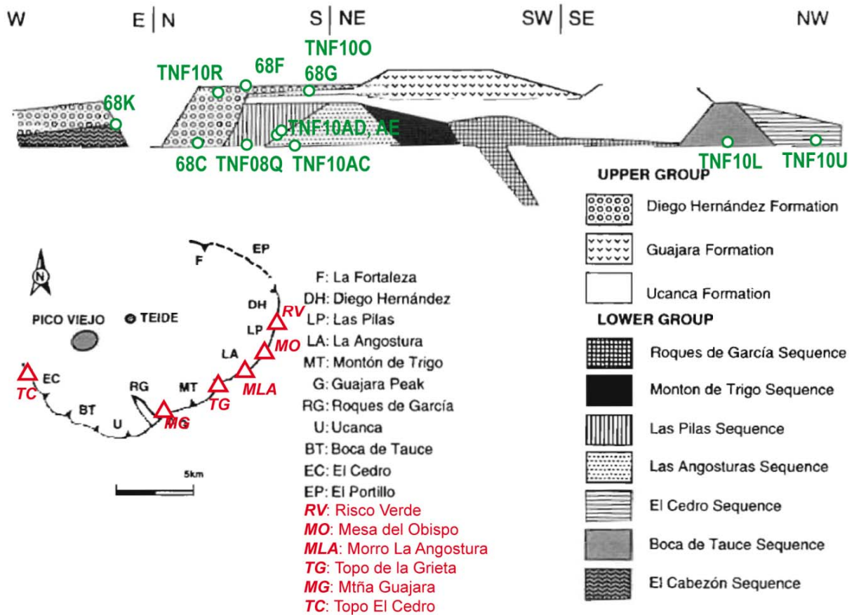
Figure II.3 : Stratigraphie de la paroi de la caldera de Las Cañadas telle que définie par Marti et al. (1994) sur laquelle nous avons ajouté les échantillons traités.
