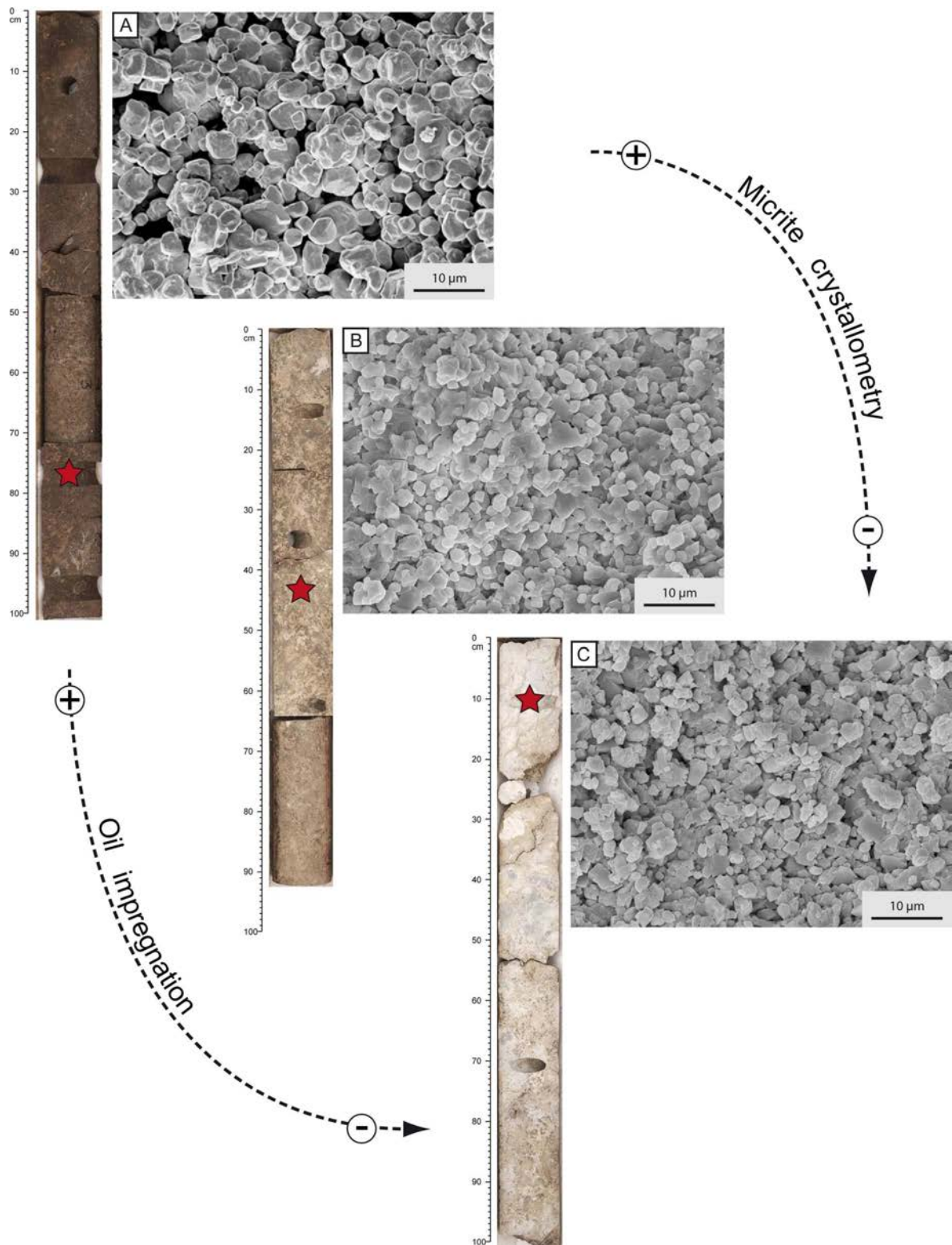
Figure 4.7. Aspect de la matrice micritique en regard de l'imprégnation de la carotte du puits G. (A) 87,7m bTMU, cristallométrie 3,64μm; (B) 8,4m bTMU, cristallométrie 2,15μm; (C) 24,1m bTMU, cristallométrie 1,79μm. Les matrices observées sont sub-arrondies à légèrement polyédrales. Les étoiles donnent la position de l'échantillon.
