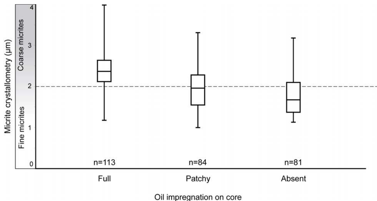
Figure 4.24: Distribution de la cristallométrie des micrites du réservoir par rapport à l'imprégnation en huile observée en carotte. Les bornes de la boîte représentent 25% et 75% de la distribution (quartiles Q1 et Q3), le trait à l'intérieur de la boîte représente la valeur médiane (50% des échantillons). Les bornes extrêmes représentent les minima et maxima de cristallométrie enregistrés pour chaque type d'imprégnation.
