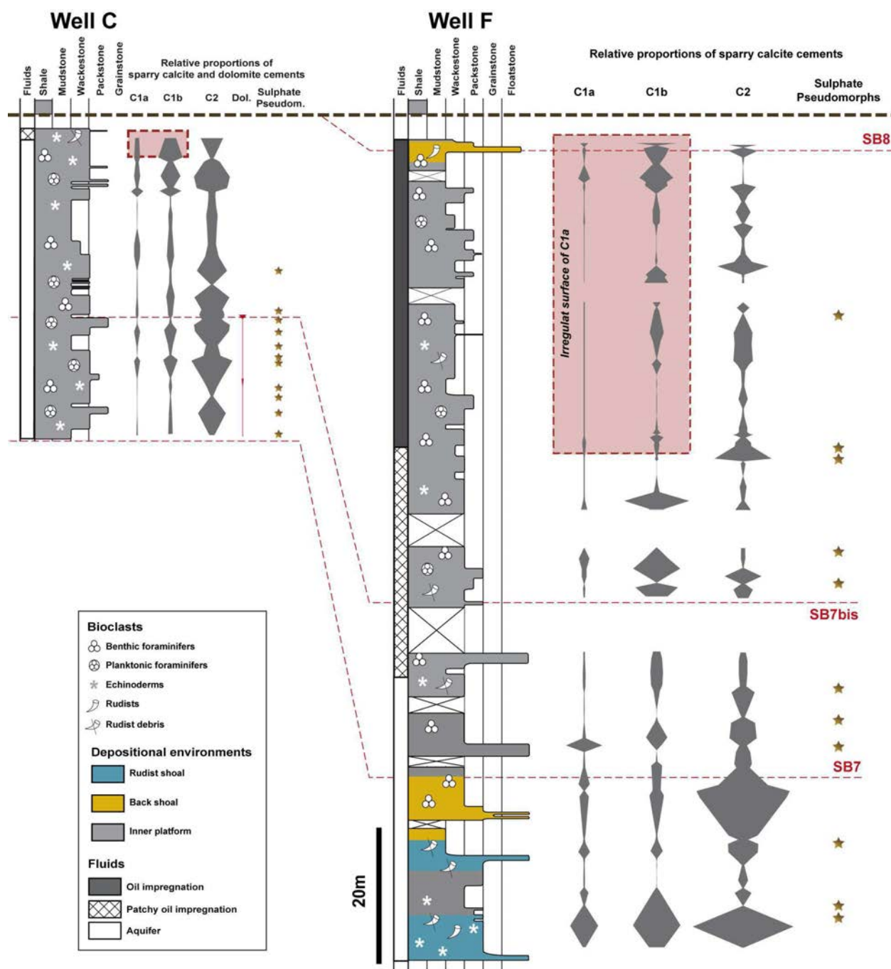
Figure 5.7. : Distribution et proportions relatives des différentes zones de cimentation (calcite-dolomite), des surfaces anhédrales de C1a et des pseudomorphoses de sulfates qui seront décrites dans les prochains paragraphes.
