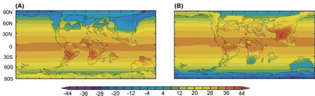
Figure 5.13 : Modélisations des variations de températures à la surface de la Terre au Crétacé supérieur (Sellwood & Valdes, 2006), entre Décembre et Février (A) et de Juin à Août (B).
