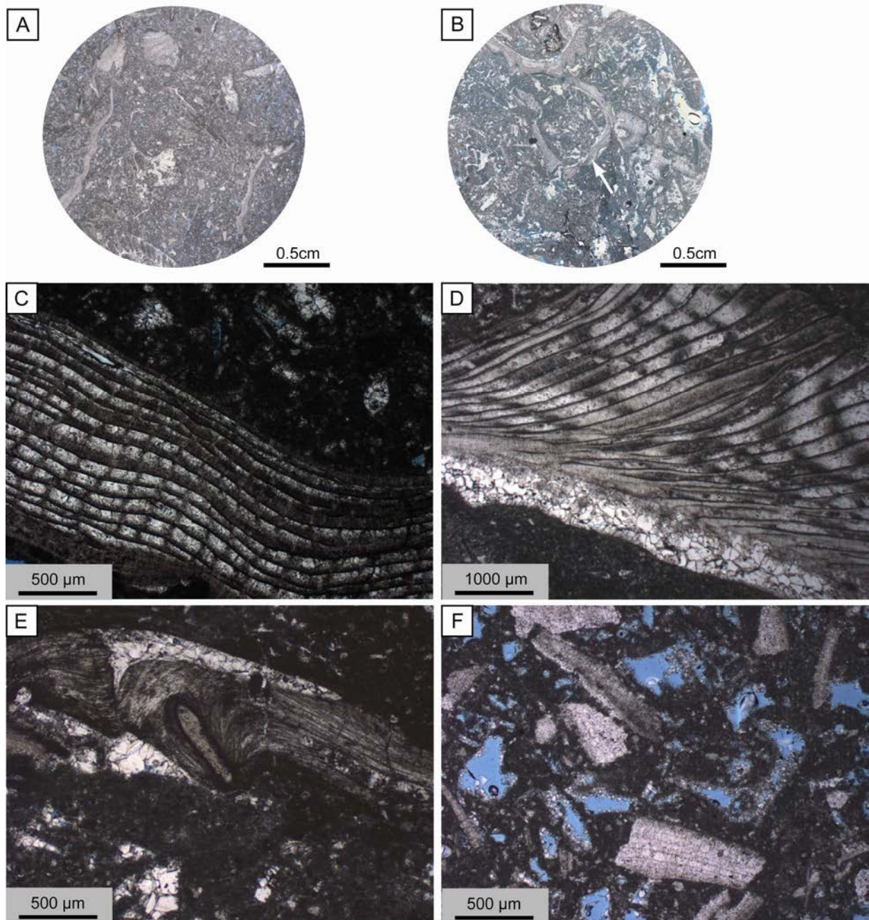
Figure 2.8. : Aspects bio-sédimentaires du faciès F8. (A-B) : Aperçu général du faciès en lame mince (échelle : 0,5cm; A : puits C; B : puits H). C : grand fragment de Radiolité (échelle : 500μm; puits D). D : grand fragment de rudiste (échelle : 1000μm; puits H). E : fragment de lamellibranche indéterminé (échelle : 500μm; puits A). F : Nombreux fragments de lamellibranches et de rudistes, symptomatiques d'un faciès de démantèlement (échelle : 500μm; puits C). La porosité observée dans ce faciès est moldique, intragranulaire et souvent matricielle.
