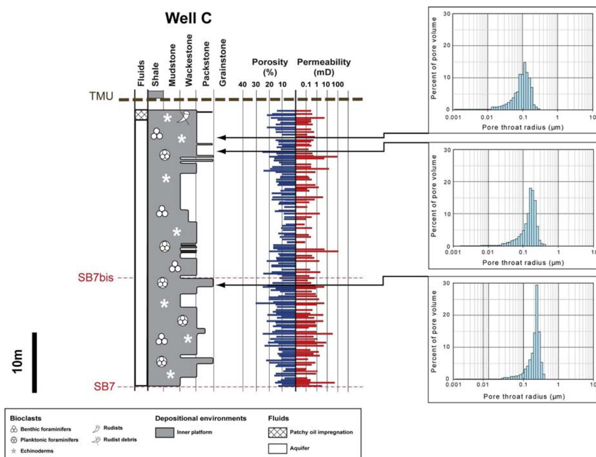
Figure 3.5 : Histogrammes de distribution des rayons de seuils de pores (PTR) pour trois échantillons du puits C. Les courbes de distribution sont toutes unimodales et présentent un aspect similaire.
