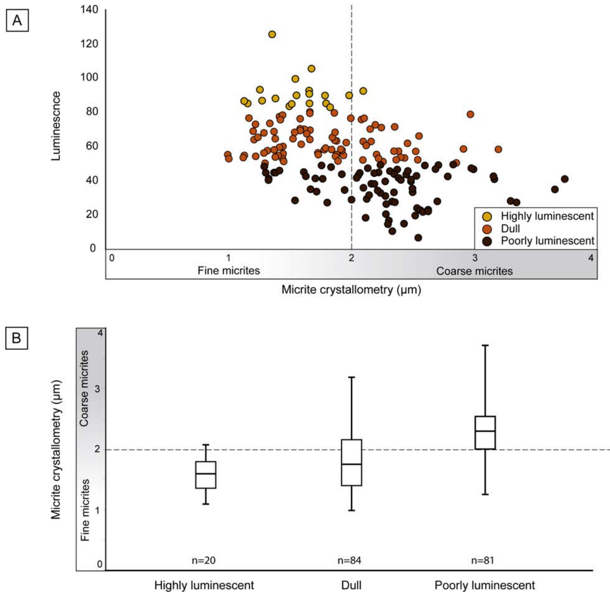
Figure 4.11. : Relations entre cristallométrie des particules micritiques et leur luminescence.
