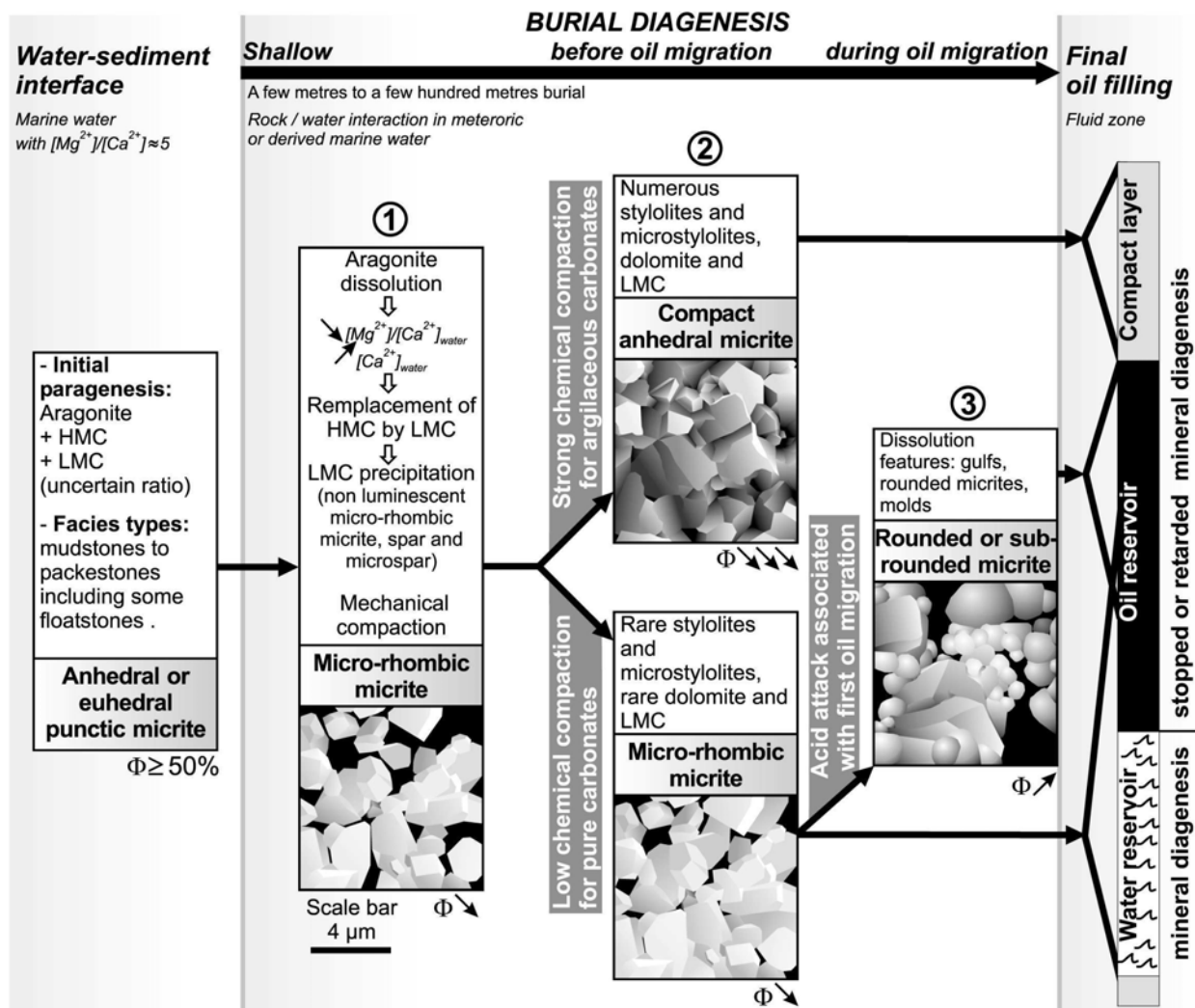
Figure 6.8 : Evolution des matrices micritiques au cours de l'enfouissement et compartimentalisation des calcaires micritiques (compact Vs microporeux) pour la Formation Mishrif d'Irak (Lambert et al. , 2006).
