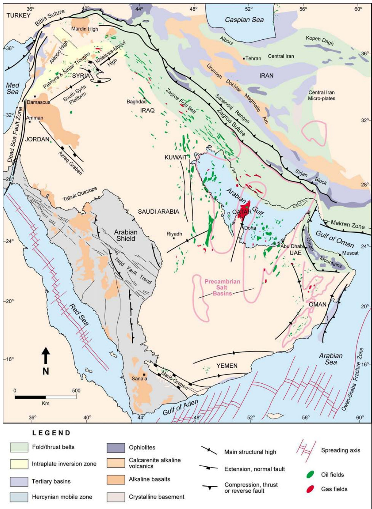
Figure 1.4 : Eléments tectoniques majeurs à l'échelle de la plaque arabe (Konert et al. , 2001).
