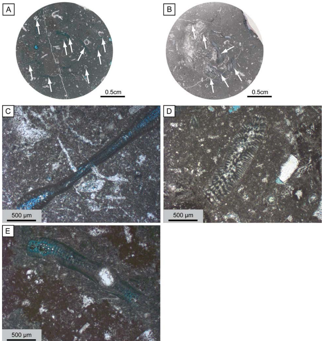
Figure 2.2. : Aspects bio-sédimentaires du faciès F2. (A-B) Aperçu général du faciès en lame mince (échelle : 0,5cm; A-B : puits F). Les flèches blanches indiquent la présence et l'abondance des grands foraminifères benthiques typiques de ce faciès. C : coupe sagittale de Cyclodomia sp. (échelle : 500µm; puits F). D : grand foraminifère benthique illustrant semble-t-il Cyclodomia sp. ou Dicyclina sp. (échelle : 500µm; puits A). E : coupe sagittale de Cyclodomia sp. montrant le proloculus de grande taille caractéristique de ce genre (échelle : 500µm; puits F). Noter la forte teneur en argile (aspect brun) de l'échantillon. La macroporosité observée dans ce faciès est essentiellement moldique. De la macroporosité intraparticulaire (loge des foraminifères) est aussi visible.
