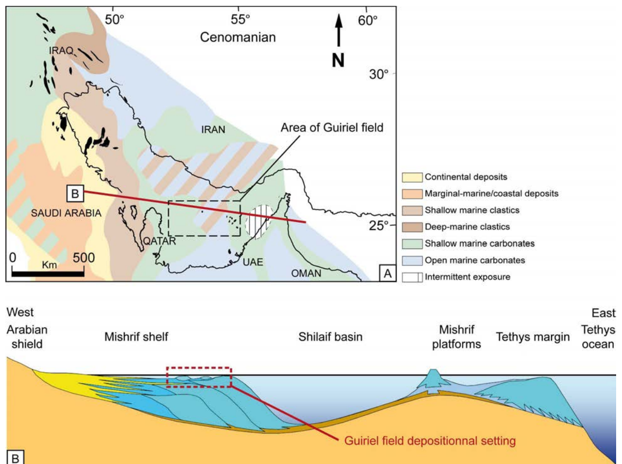
Figure 2.16 : (A) Reconstitution paléogéographique du Golfe persique au Cénomaniens montrant le développement des plates-formes carbonatées (d'après Ziegler, 2001). (B) Coupe synthétique ouest-est montrant les liens entre la plate-forme Mishrif et le bassin du Shilaif (Al-Zaabi et al. , 2010).
