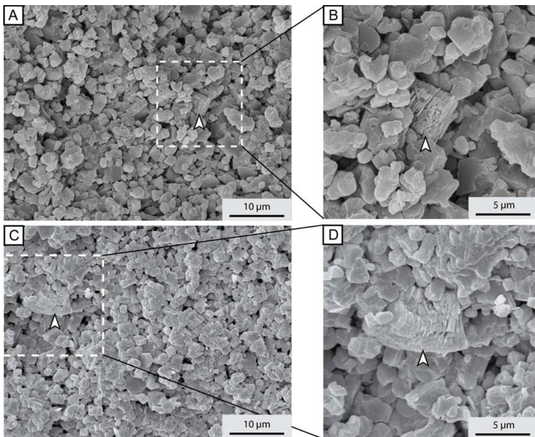
Figure 2.14 : Feuilles de kaolinite piégés dans la matrice micritique. (A-B) Puits G. 24,1 mètres sous la discontinuité sommitale; (C-D) Puits A. 32,9 mètres sous la discontinuité sommitale.
