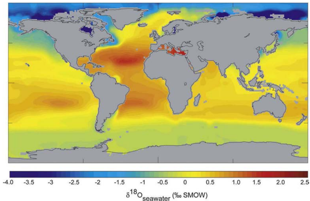
Figure 5.16 : Carte de la distribution mondiale des valeurs du ^{18}\text{O} des eaux marines actuelles (LeGrande & Schmidt, 2006; Lachniet, 2009).
