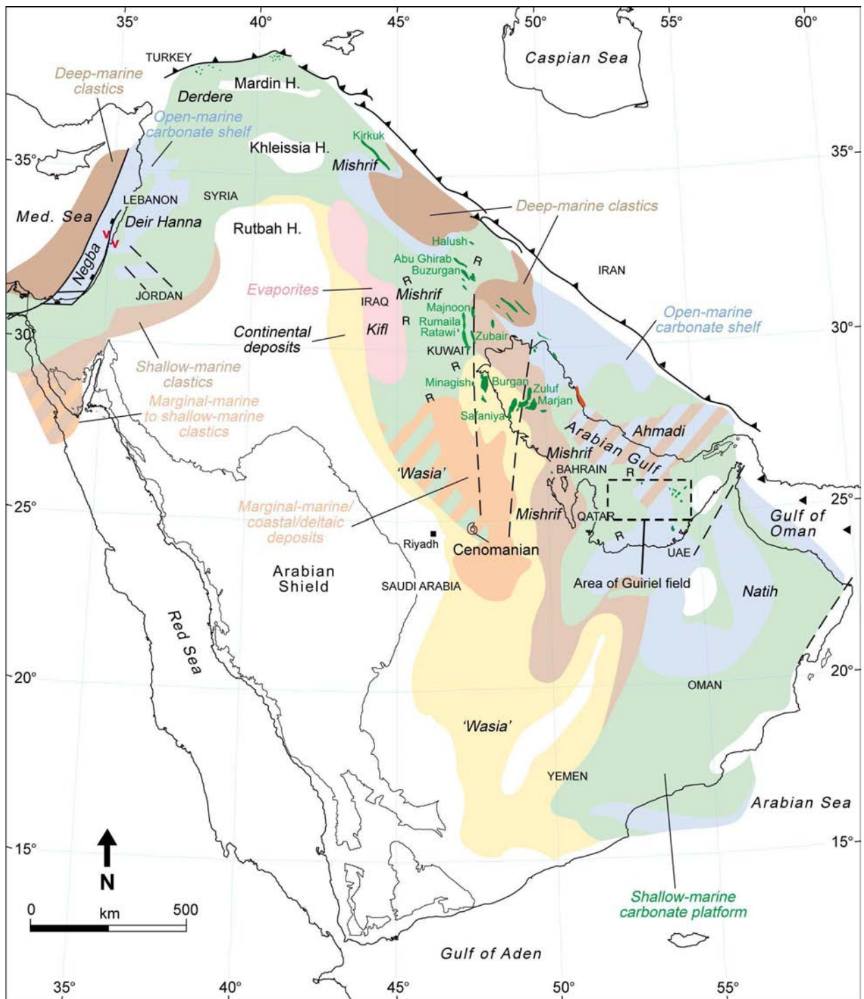
Figure 1.7 : Carte paléogéographique de la péninsule arabe pour l'intervalle Cénomanién-Turonien pointant la position de la Formation Mishrif et de ses équivalents latéraux, Natih et Sarvak (Ziegler, 2001).
