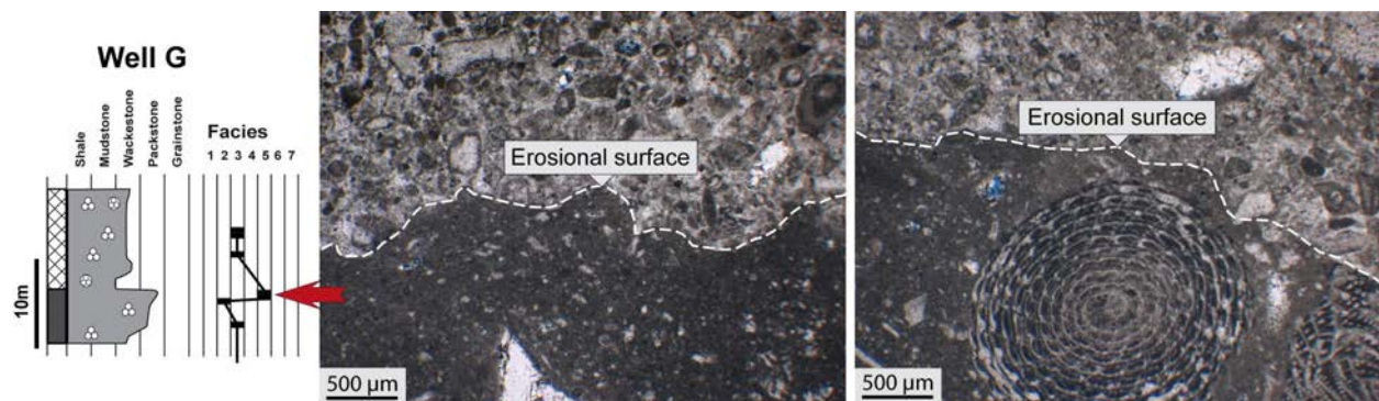
Figure 2.19 : Exemple d'un niveau de tempête avec base érosive identifié dans le puits xx.
