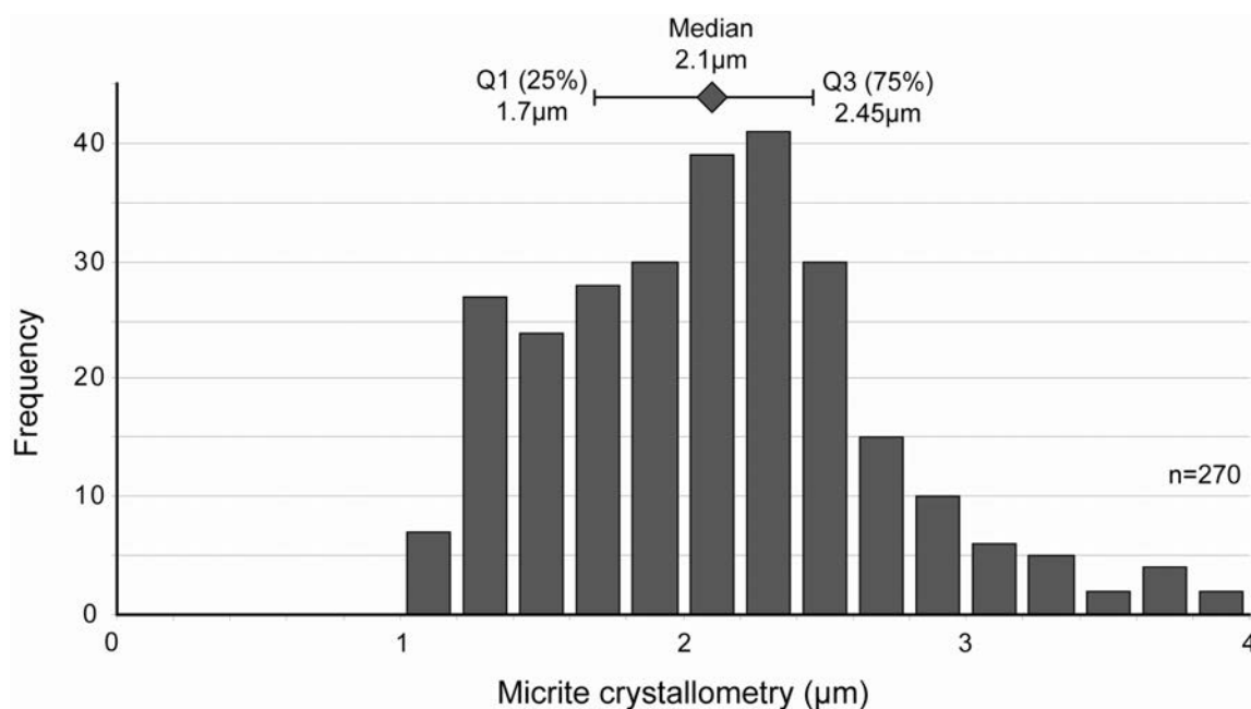
Figure 4.5. : Distribution de la cristallométrie des 270 échantillons du champ Guiriel.
