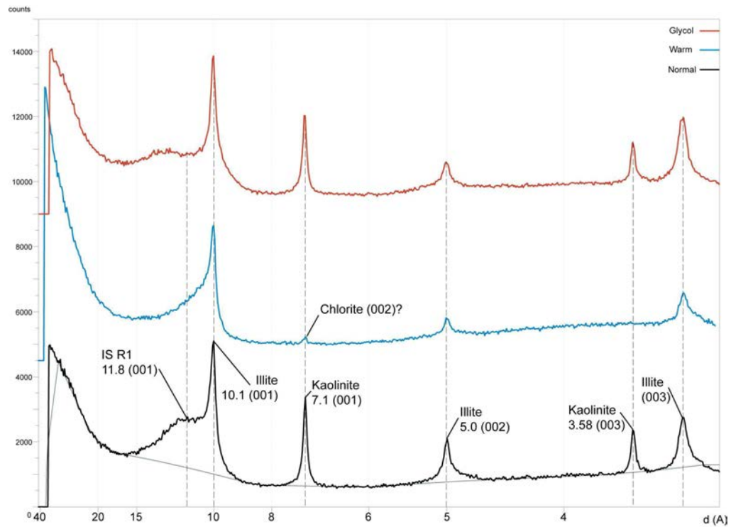
Figure 2.13 : Exemple de diffractogramme obtenu pour l'analyse des argiles en DRX. Puits C, 37 mètres sous la discontinuité sommitale.
