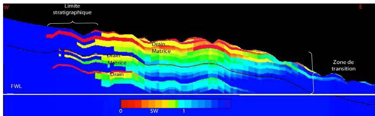
Figure 3.9 : Modèle réservoir simplifié montrant les saturations en eau (Sw) des différents drains et de la matrice du champ Guiriel, ainsi que le piège stratigraphique localisé à l'ouest du champ (Modifié d'après Botton-Dumay et al. , 2002).
