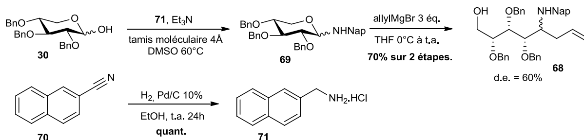
Schéma 32. Obtention du \delta -aminoalcool 68.
