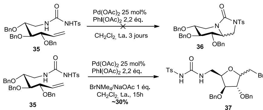
Schéma 26. Essais de diaminations sur notre substrat.
