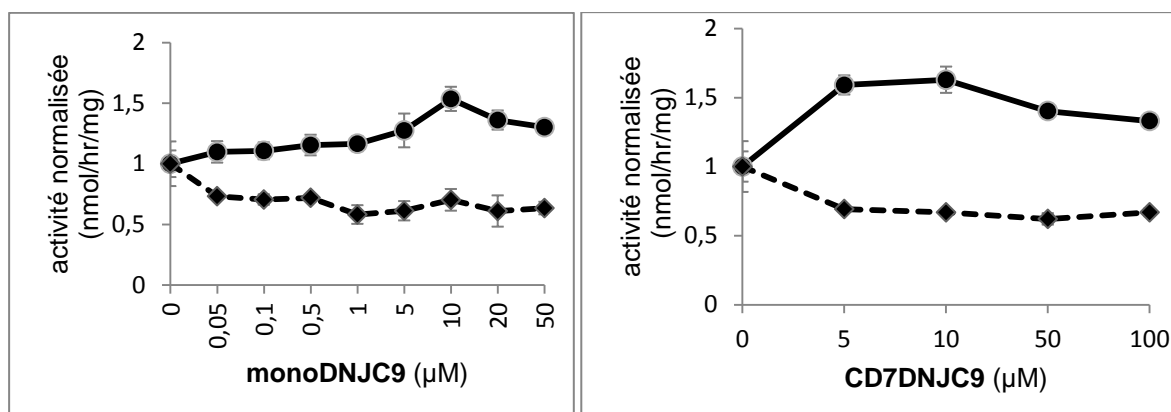
Figure 78. Activités normalisées de la GCase mutée N370S -●- et de l'α-glucosidase lysosomale --◆-- en présence des composés monoDNJC9 et CD7DNJC9 à différentes concentrations
