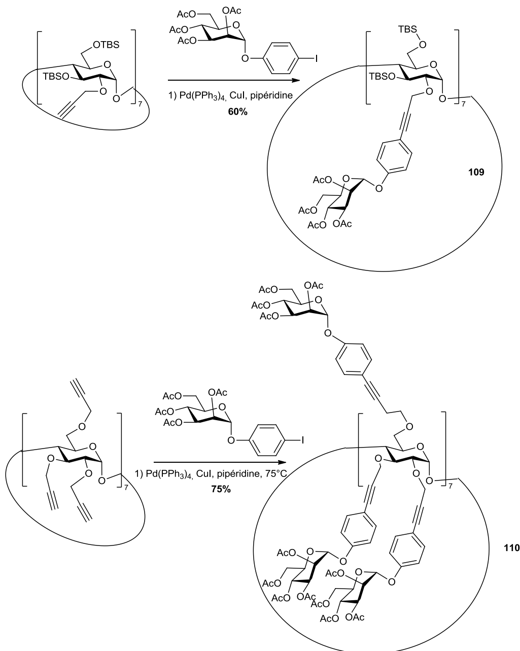
Schéma 54 Introduction des unités osidiques par couplage de Sonogashira.
