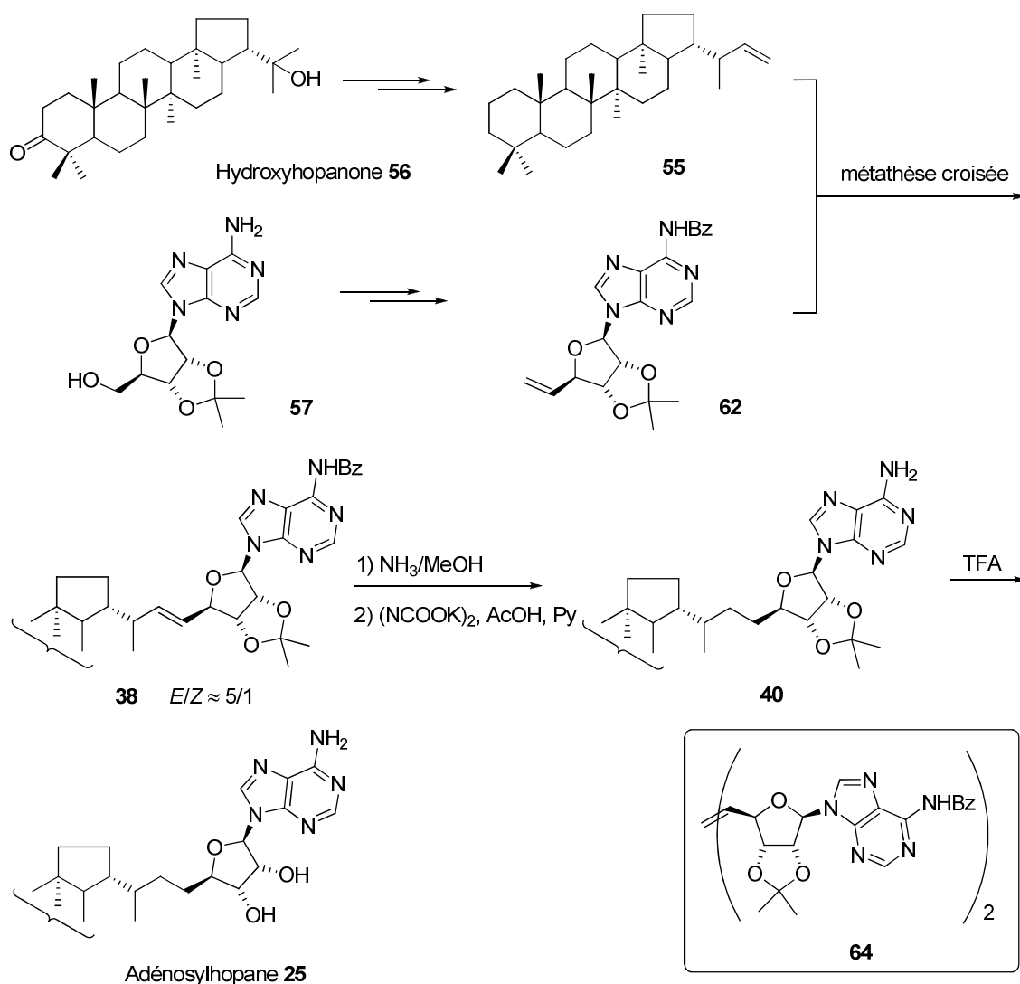
Schéma 2. Hémisynthèse de l'adenosylhopane 25 .
