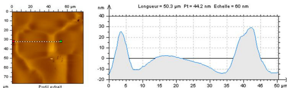
Figure 9 : Profil obtenu à partir de l'analyse de topographie dans la zone polarisée d'une lame de microscope polarisée sous air à 1 kV à 220°C pendant 5 minutes.
