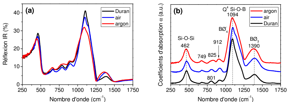
Figure 3 : Spectres de réflexion IR du verre Duran® et de 2 lames polarisées sous air et sous argon (a) et les coefficients d'absorption \alpha correspondants calculés par transformée de Kramers-Krönig (b).
