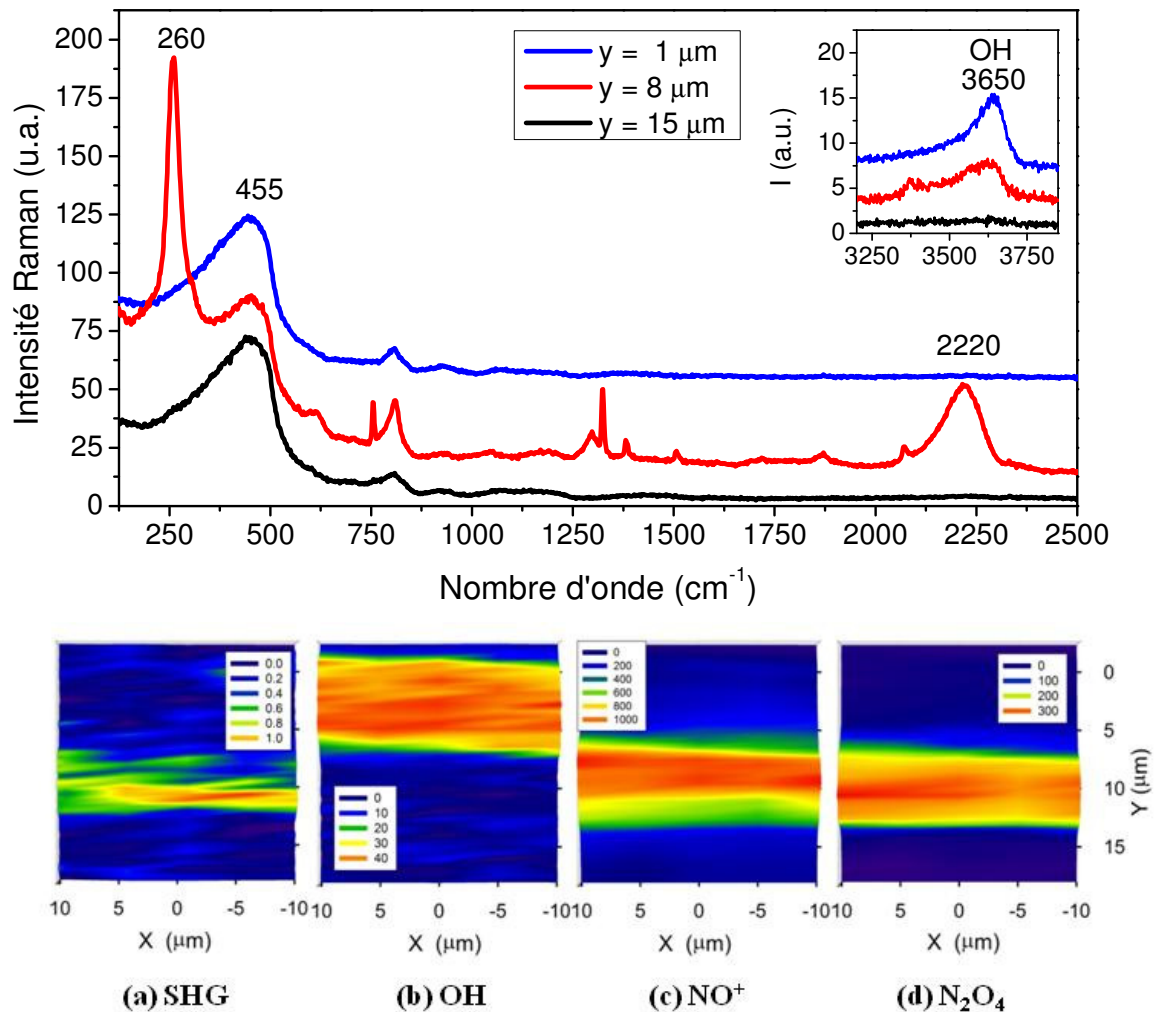
Figure 4 : Spectres Raman d'une lame Duran® polarisée sous air et cartographies associées (micro-Raman et micro-SHG).
