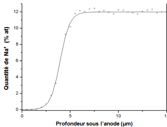
Figure 7 : Exemple du profil de la quantité de sodium en fonction de la profondeur sous l'anode (en % at).
