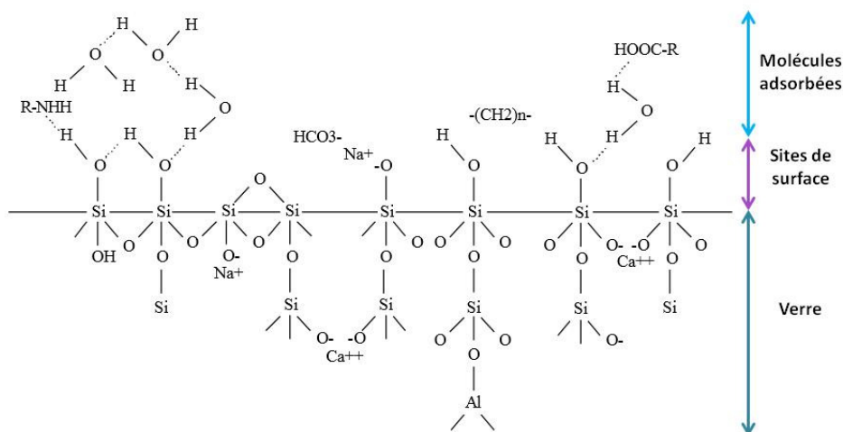
Figure 32 : Représentation schématique d'une surface de verre sodocalcique réelle. [18]
