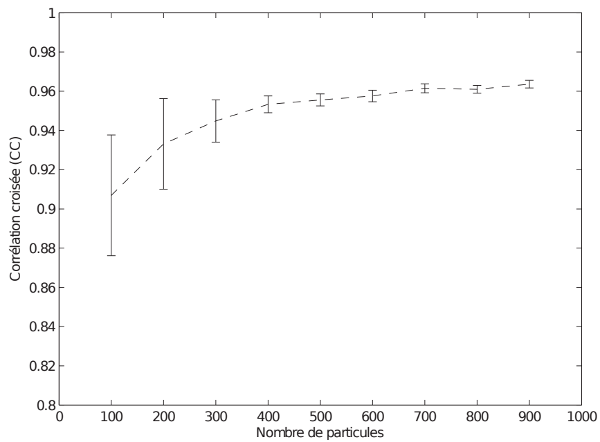
FIGURE 4.9 – Ce graphique représente la mesure de similarité (corrélation) de tractographies de 100 à 900 particules avec les tractographies initiales avec 1000 particules. Cette expérience montre comment le nombre de particules influence la précision de la solution estimée. Le principal bénéfice d’une diminution du nombre de particules est la réduction du temps de calcul.
