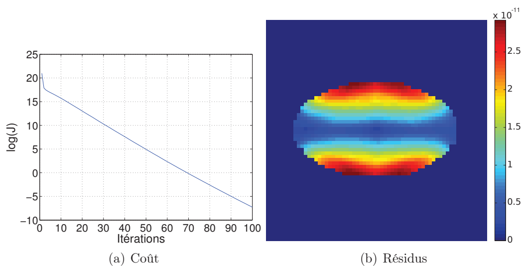
FIGURE 7.6 – Valeurs de la fonction de coût J pour les 100 premières itérations et des résidus après 100 itérations pour l'expérience uni-directionnelle.
