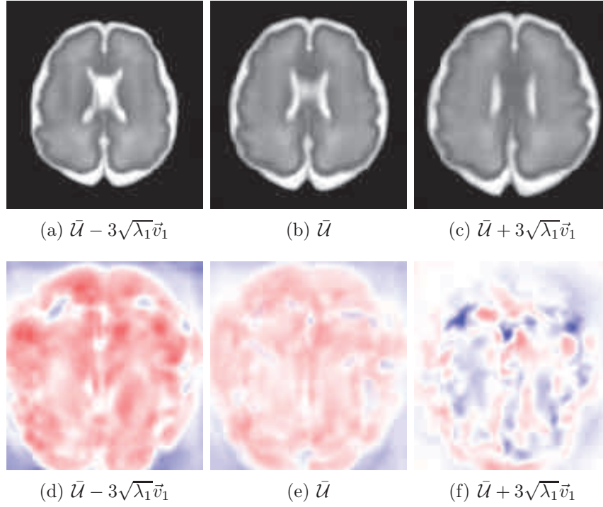
FIGURE 7.3 – Illustration du premier mode de déformation difféomorphique. La première ligne montre des images IRMs pondérées en T2 ; la deuxième ligne affiche le jacobien en base logarithmique (les couleurs rouge, bleue et blanche représentent respectivement une expansion, une contraction et une absence de changement).
