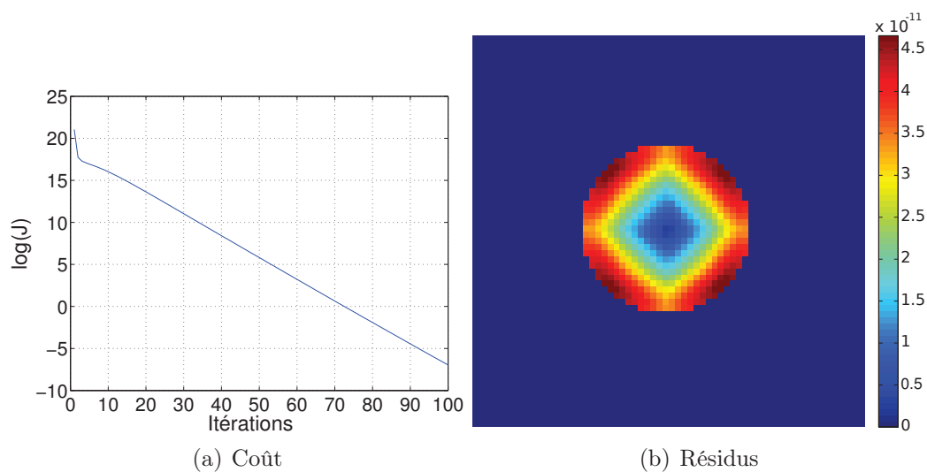
FIGURE 7.10 – Valeurs de la fonction de coût J pour les 100 premières itérations et des résidus après 100 itérations pour l’expérience bi-directionnelle.
