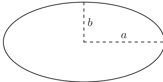
FIGURE B.1 – Exemple d'ellipse paramétrée par ses deux axes de longueurs respectives a et b .
