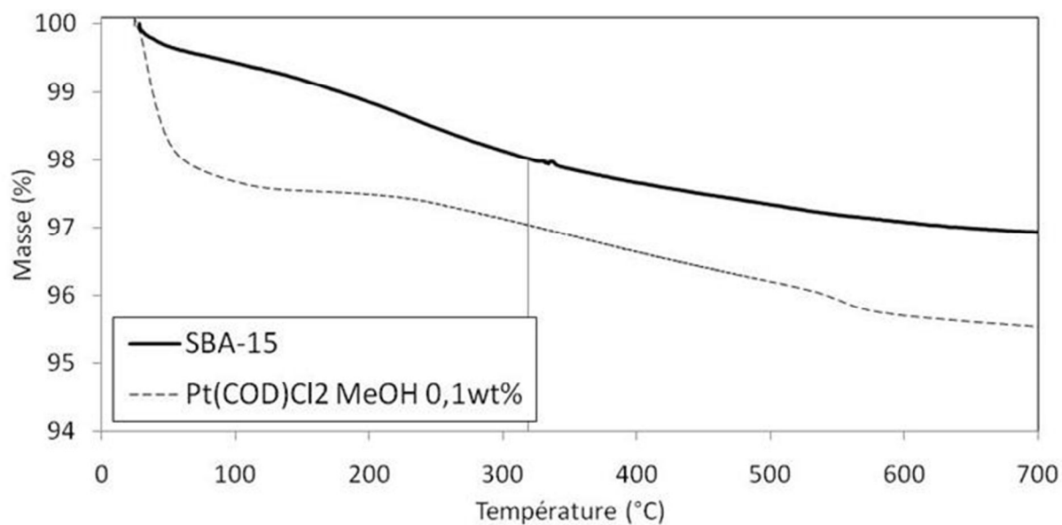
Figure A.22 : Courbe ATG sous air de la silice mésoporeuse SBA-15 et du catalyseur Pt/SBA-15 préparé à partir de Pt(COD)Cl 2 . Les traits verticaux représentent les pertes de masses du précurseur Pt(COD)Cl 2 seul (cf. chapitre 2).
