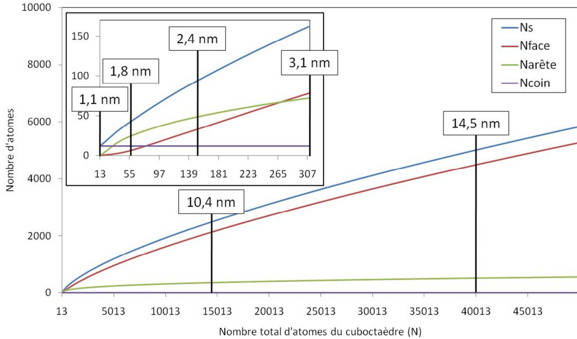
Figure 4.37 : Evolution du nombre d'atomes de surface ( N_s ), de faces ( N_{\text{face}} ), d'arêtes ( N_{\text{arête}} ) et de coins ( N_{\text{coin}} ) d'un cuboctaèdre en fonction de son nombre total d'atomes ( N ). Les tailles moyennes du cuboctaèdre correspondantes retrouvées dans les échantillons d'EuroPt-1 sont indiquées.
