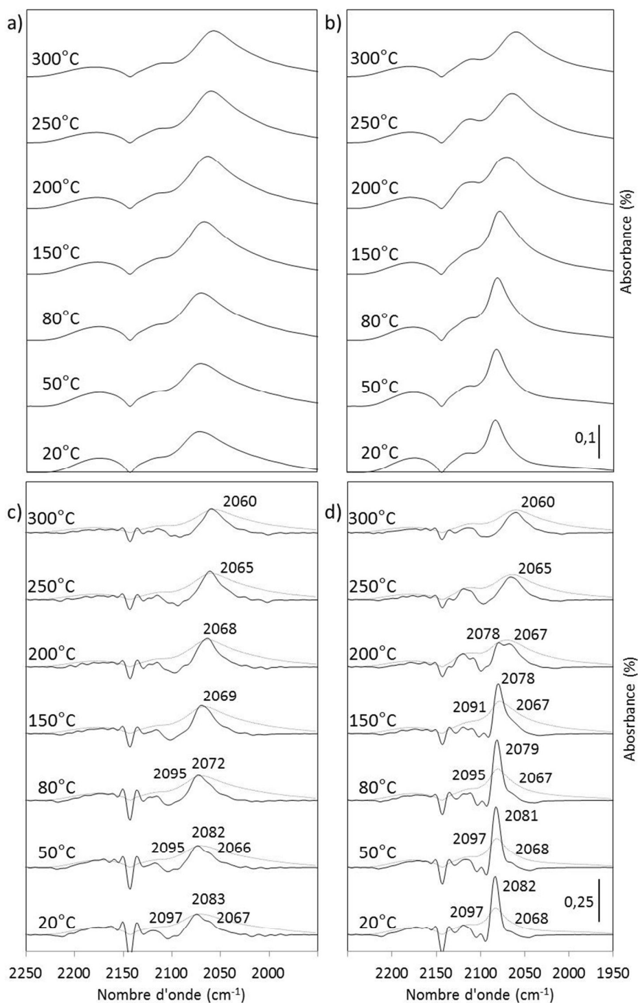
Figure 4.7 : Spectres IR recentrés sur la fenêtre d'adsorption du CO ( 1950\text{--}2250\text{ cm}^{-1} ) mesurés entre 20 et 300^\circ\text{C} sous une atmosphère de CO (4 % dans l'hélium) pour EuroPt-1 a) réduit et b) non réduit ; et déconvolution de ces mêmes spectres (EuroPt-1 c) réduit et d) non réduit) suivant la méthode de « déconvolution par transformée de Fourier ».
