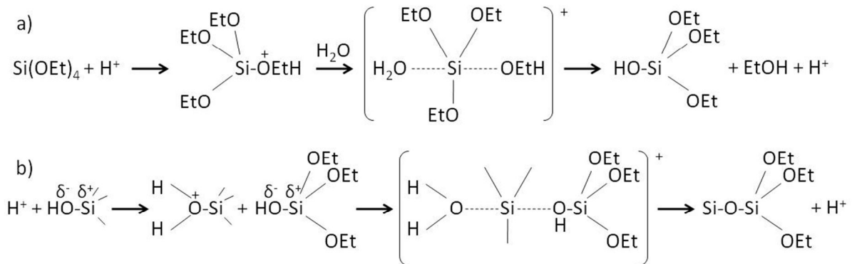
Figure 3.11 : Mécanismes de substitution nucléophile SN2 des étapes a) d'hydrolyse et b) de condensation d'un procédé sol-gel hydrolytique acide (Et = CH 2 CH 3 ).
