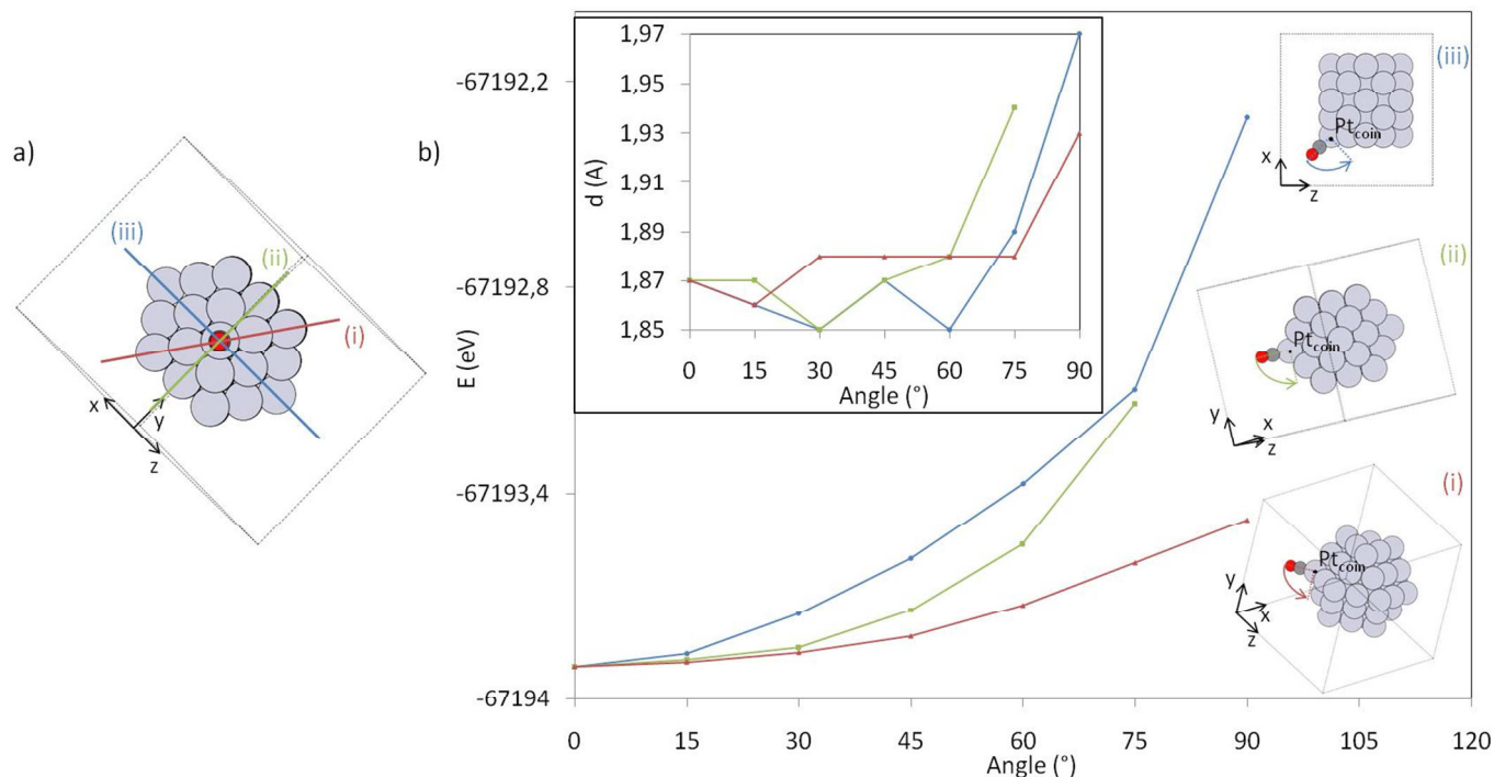
Figure 4.17 : a) Vue du système « Pt55 + 1CO coin » selon l'axe de la molécule de CO, et b) calcul DFT du couple (E, d) avec la variation de l'angle (\overrightarrow{\text{Pt}_{\text{coin}}\text{C}_{\text{init}}}, \overrightarrow{\text{Pt}_{\text{coin}}\text{C}_{\text{f}}}) selon trois plans : (i) celui passant par les atomes de coins et d'arêtes, et ceux passant par (ii) le centre des faces (111) et (iii) le centre des faces (100).
