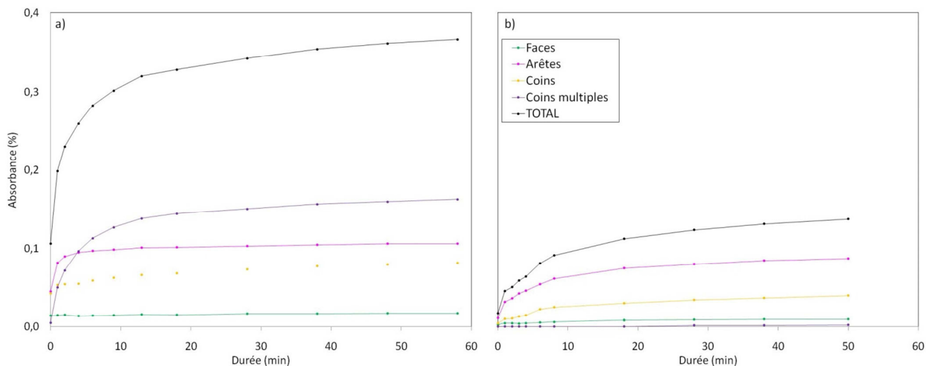
Figure 4.22 : Evolution de l'adsorption du CO sur les différents sites d'un cuboctaèdre de platine (faces, arêtes, coins et coins multiples) et leur somme, mesurée à température ambiante sous 0,5 % CO dans l'hélium, en fonction de la durée, pour EuroPt-1 a) réduit et b) non réduit.
