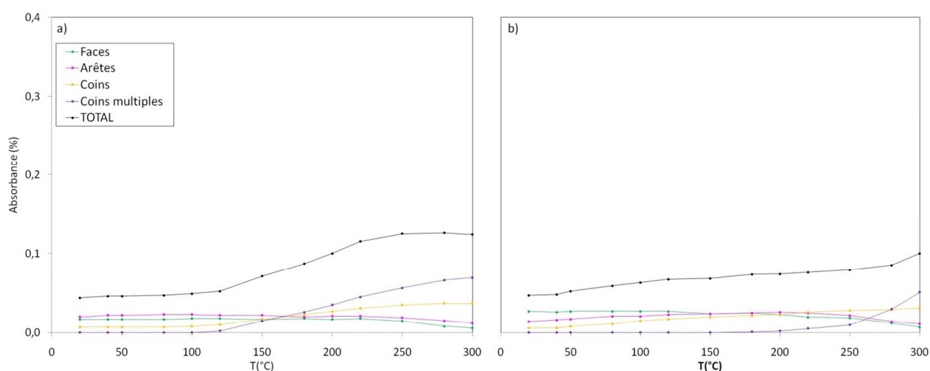
Figure 4.35 : Evolution de l'adsorption du CO sur les différents sites des cuboctaèdres de platine (faces, arêtes, coins et coins multiples) et leur somme, mesurée sous 4% CO dans l'hélium, en fonction de la température (5°C/min) avec stabilisation (palier de 5 min à chaque point), pour EuroPt-1 calciné à 700°C (« calc700°C ») a) réduit et b) non réduit.
