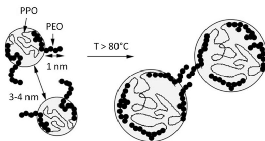
Figure 3.9 : Représentation schématique de la déshydratation des micelles avec la température. Figure adaptée de [27].
