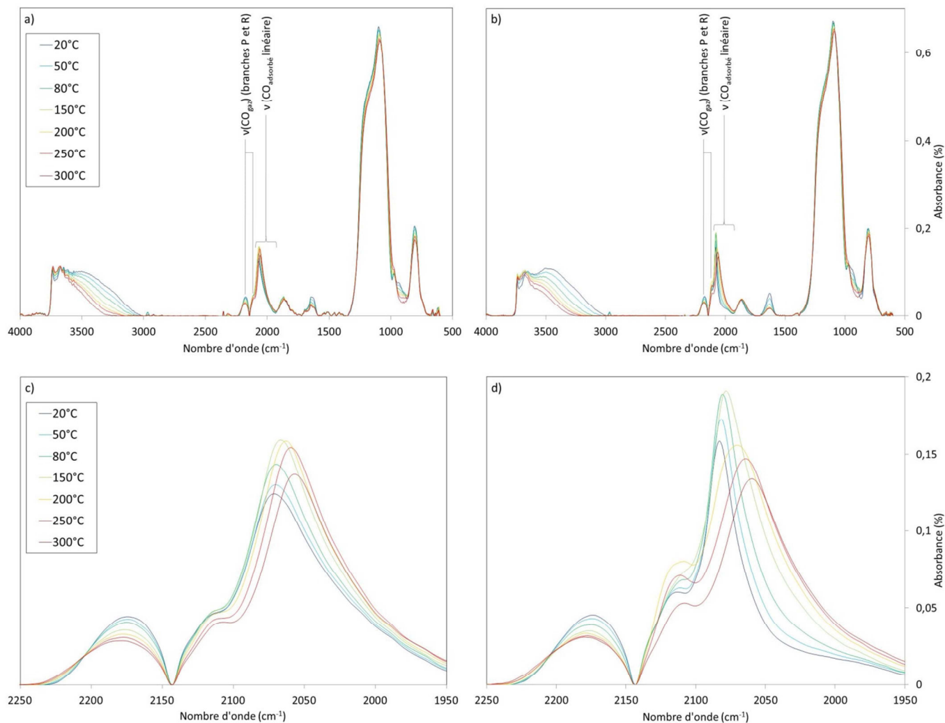
Figure 4.6 : Spectres IR superposés d'EuroPt-1 a) réduit et b) non réduit mesurés sous une atmosphère de CO à 4 % dans l'hélium, de 20 à 300°C, et c) et d) agrandissements entre 2250 et 1950 \text{cm}^{-1} respectifs.
