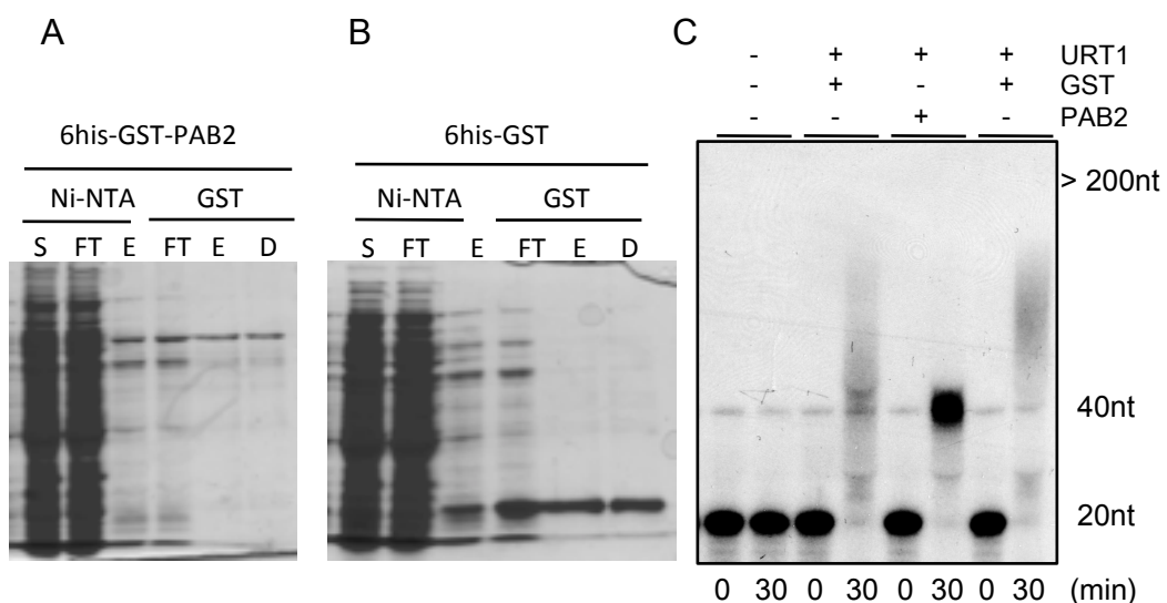
Figure D2 : PAB2 inhibe l'activité de URT1
