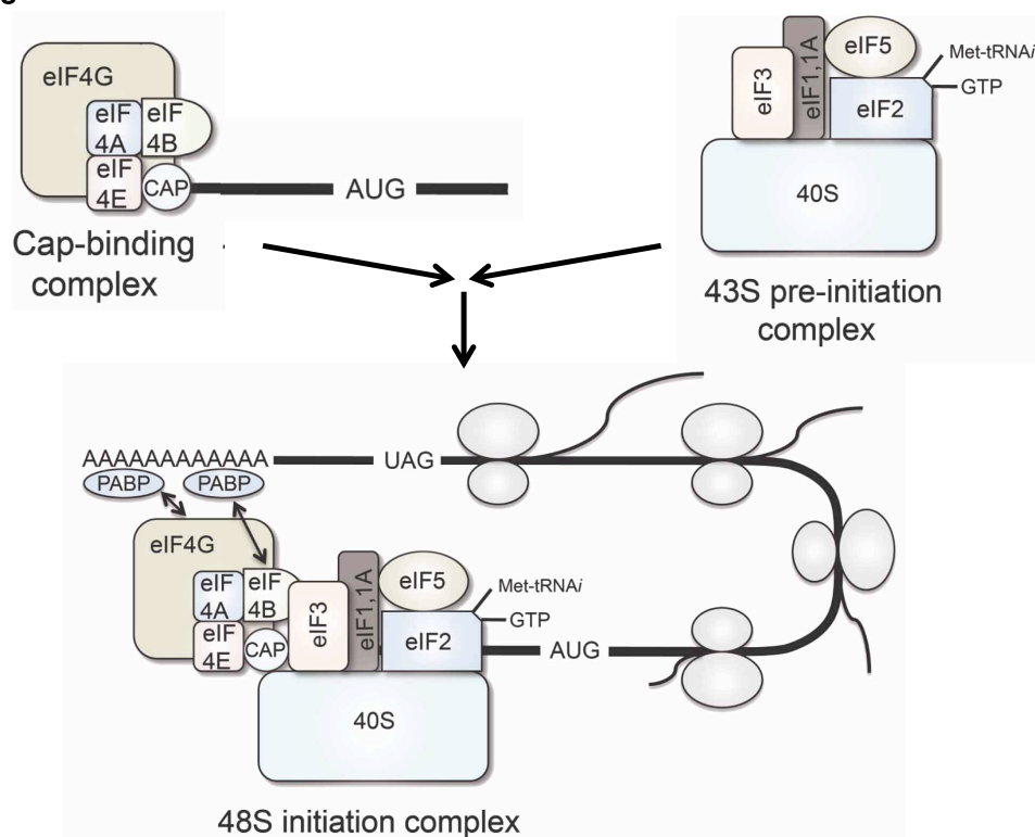
Figure IC.4 : Assemblage du complexe d'initiation de la traduction
