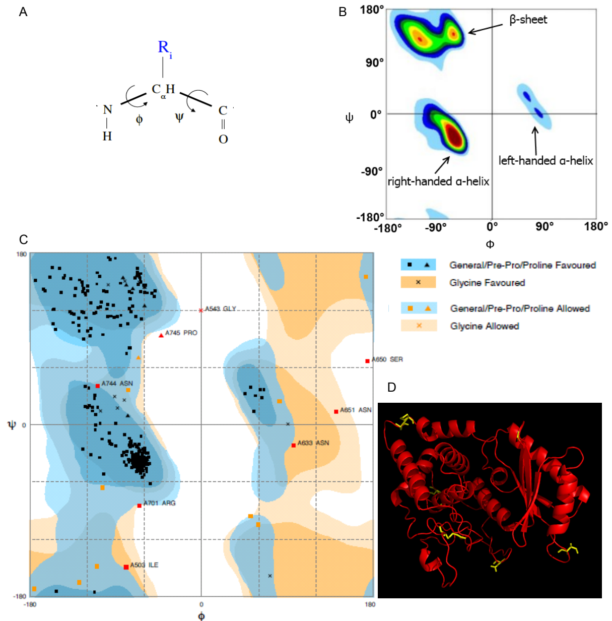
Figure 2B.1 : Représentation du diagramme de Ramachandran de la structure 3D modélisée du domaine nucléotidyltransférase de URT1
