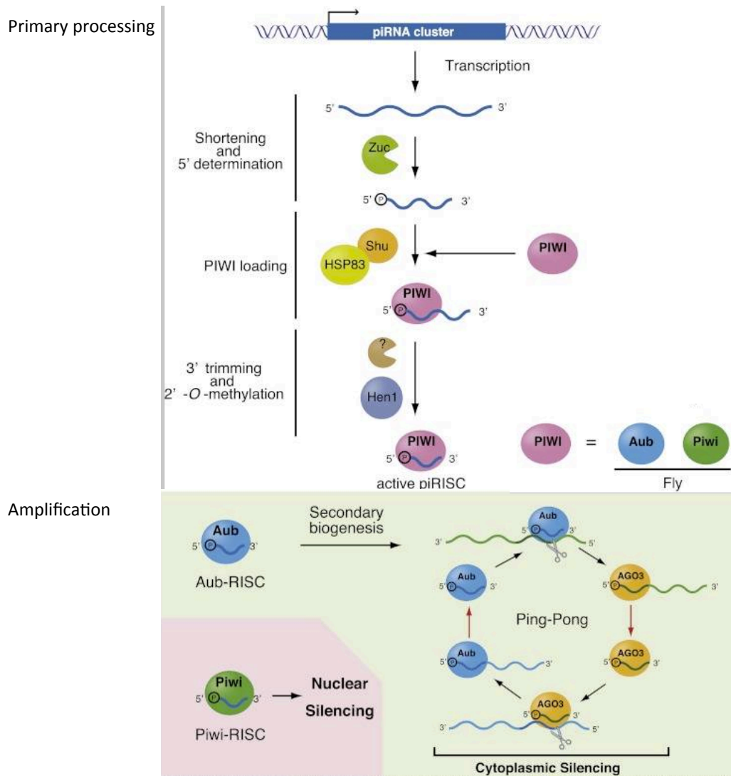
Figure IB.2 : La voie de biogenèse des piARN
