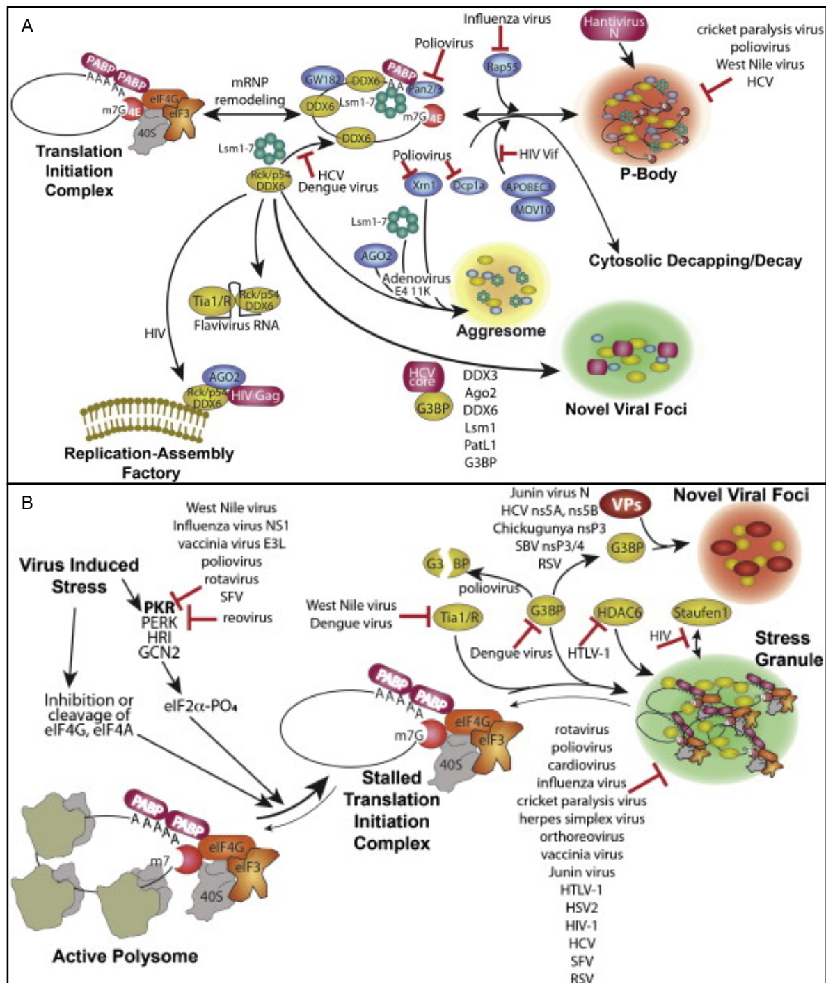
Figure 1C.8 : Les composants des processing bodies et des granules de stress peuvent être détournés par les virus pour leur réplication
