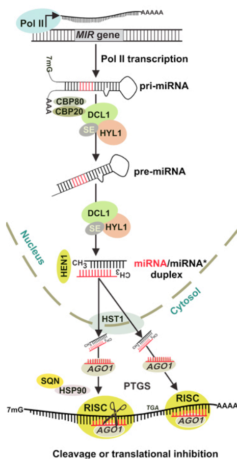
Figure IB.3 : La voie de biogenèse et le fonctionnement des microRNA et des siARN chez les plantes
