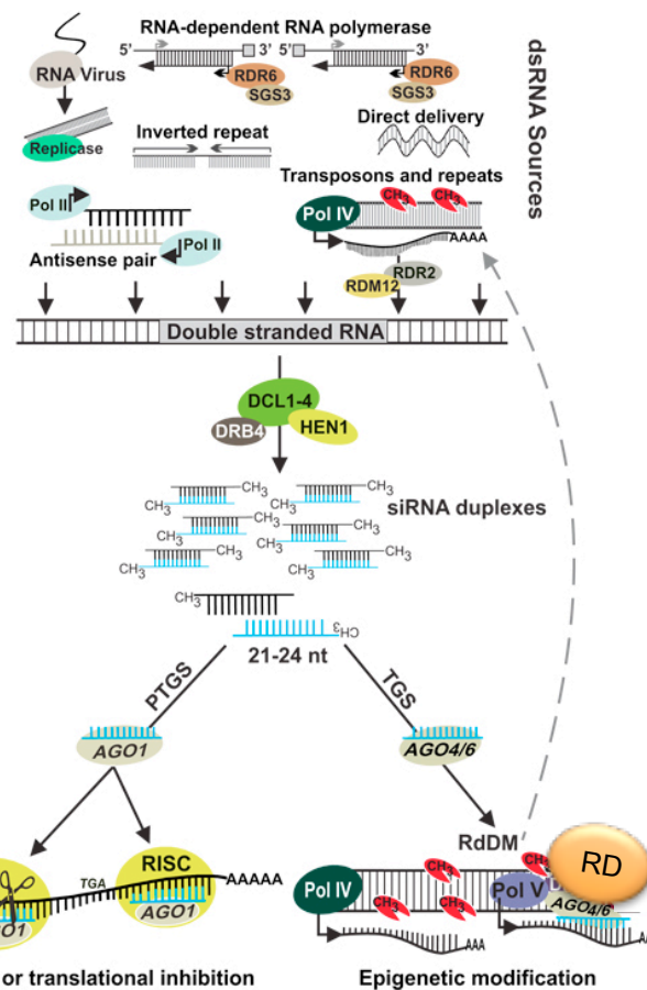
Figure IB.3 : La voie de biogenèse et le fonctionnement des microRNA et des siARN chez les plantes
