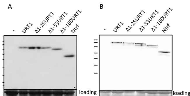
Figure 3.2 : L'expression de URT1 et de ses délétions avec une étiquette YFP fusionnée en N et en C terminale est similaire
