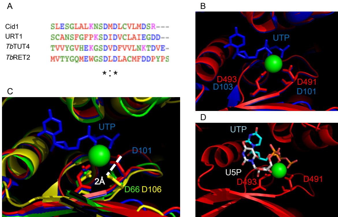
Figure 2B.4 : Transposition des ligands UTP, magnésium et U5P dans le site actif de URT1 modélisé
