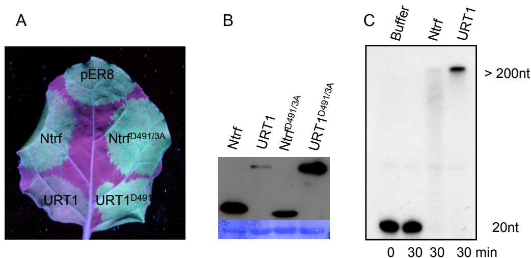
Figure D3 : La région en N terminal de URT1 est essentielle à l'activité optimale de URT1
