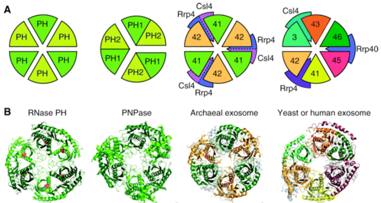
Figure 1A4 : Architecture de la RNase PH, des PNPases et de l'exosome
