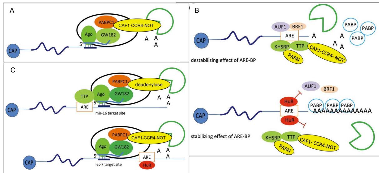
Figure 1A.3 : La régulation de la déadénylation
