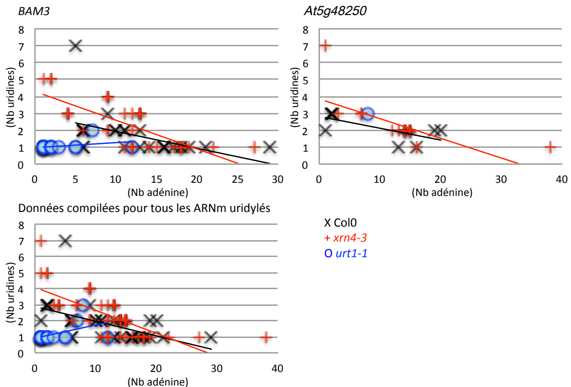
Figure 2A.2 : Le nombre d'uridines ajoutées en 3' est plus important lorsque le nombre d'adénines est faible pour les ARNm associés aux polysomes dans le mutant xrn4-3
