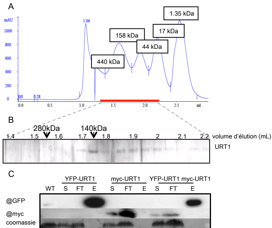
Figure 2B.13: URT1 est active sous forme de monomère
