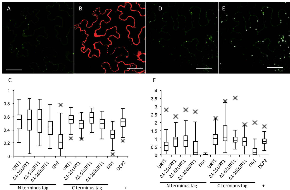
Figure 3.6: Une partie de la région N terminale de URT1 est essentielle à la localisation de URT1 au niveau des processing bodies
