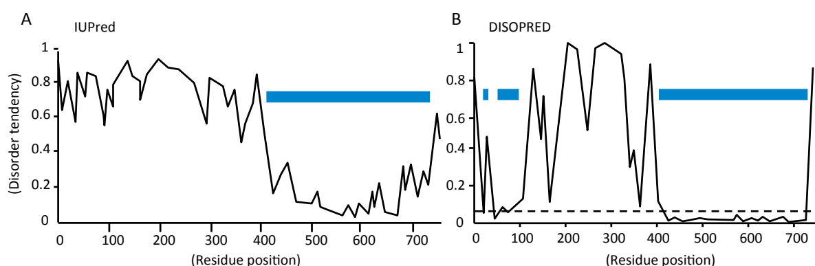
Figure 1.4 : La région N terminale de URT1 est prédite intrinsèquement désorganisée
