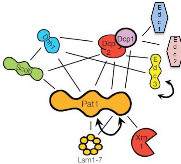
Figure IA.7 : Les facteurs interagissant avec le complexe d'élimination de la coiffe pour la dégradation 5'-3' chez S. cerevisiae
