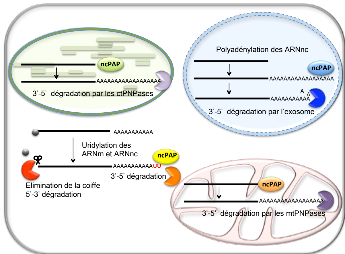
Figure IA.10 : L'implication des ncPAP dans la dégradation des ARN
