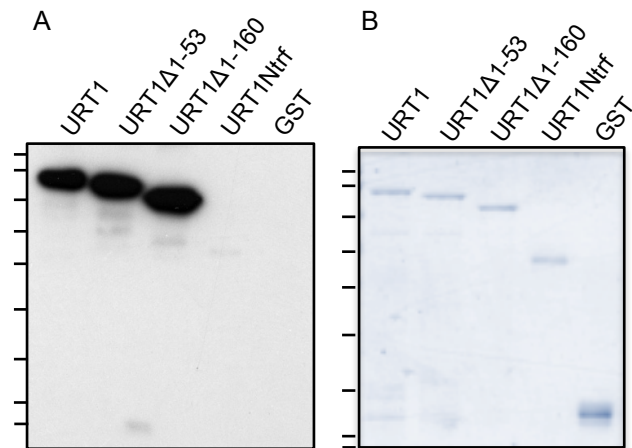
Figure D5 : Les anticorps dirigés contre URT1 ne reconnaissent pas le domaine nucléotidyltransférase
