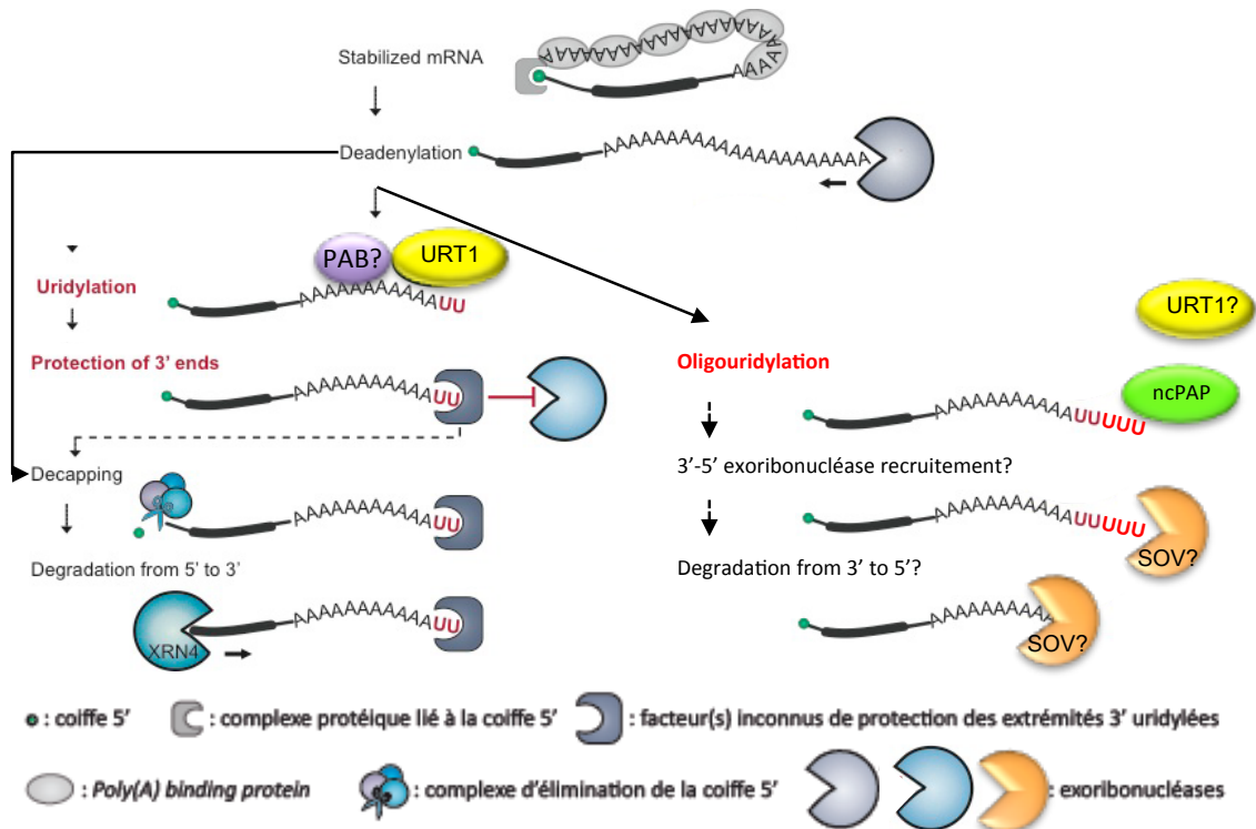
Figure D8 : Le mécanisme d'uridylation des ARNm oligoadénylés par URT1 chez A. thaliana
