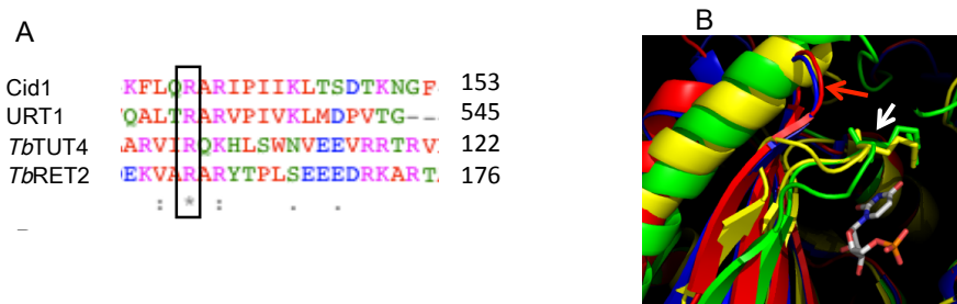
Figure 2B.12 : URT1 ne possède pas d'équivalent à l'arginine nécessaire à la spécificité du substrat ARN de TbTUT4 et TbRET2
