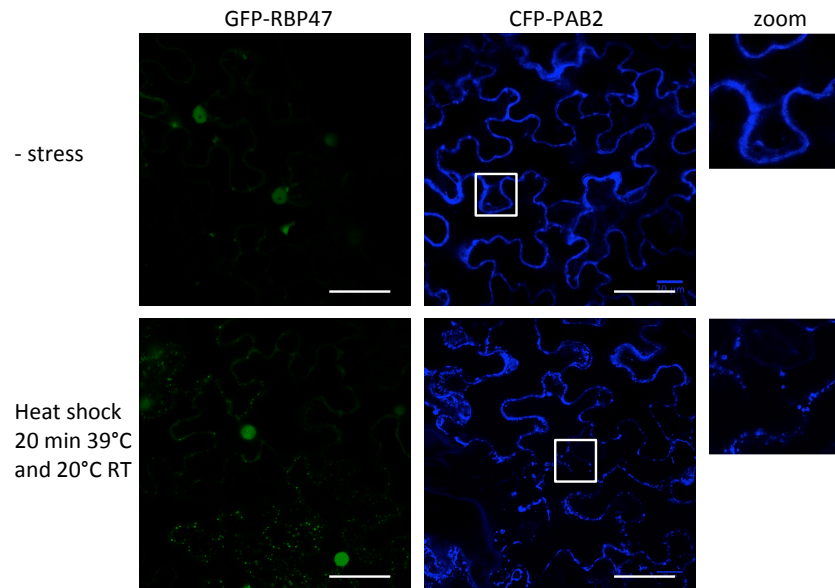
Figure 3.9 : La localisation des marqueurs des granules de stress après un stress thermique
