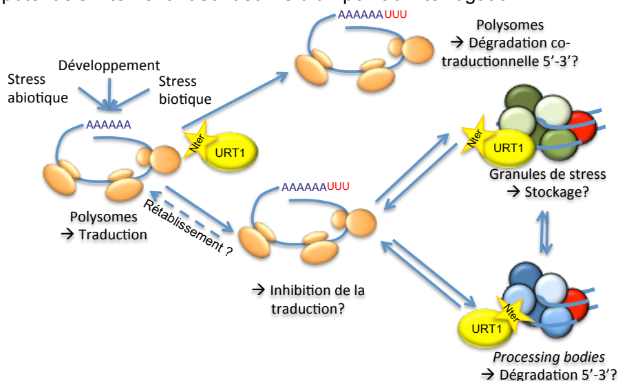
Figure D9 : Les rôles hypothétiques de l'uridylation des ARNm déadénylés par URT1 chez A. thaliana dans « le cycle de l'ARNm »
