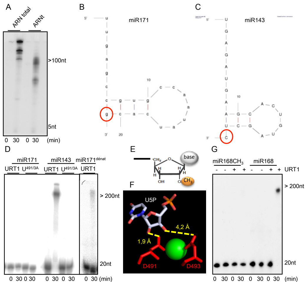
Figure 2B.11: URT1 est capable d'uridyler in vitro les ARN ayant une extrémité 3' libre et non-modifiée
