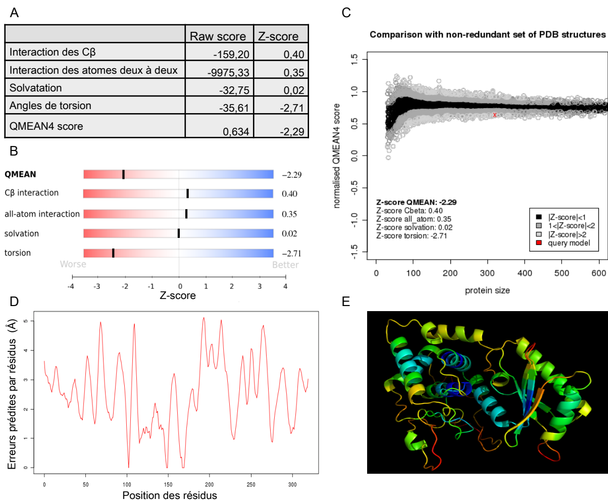
Figure 2B.2 : Validation statistique du modèle de URT1 et mise en évidence des erreurs prédites par résidus
