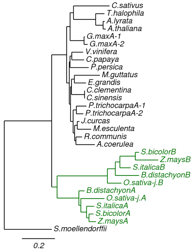
Figure 1.6: Les monocotylédones possèdent deux homologues de URT1 (URT1A et URT1B)
