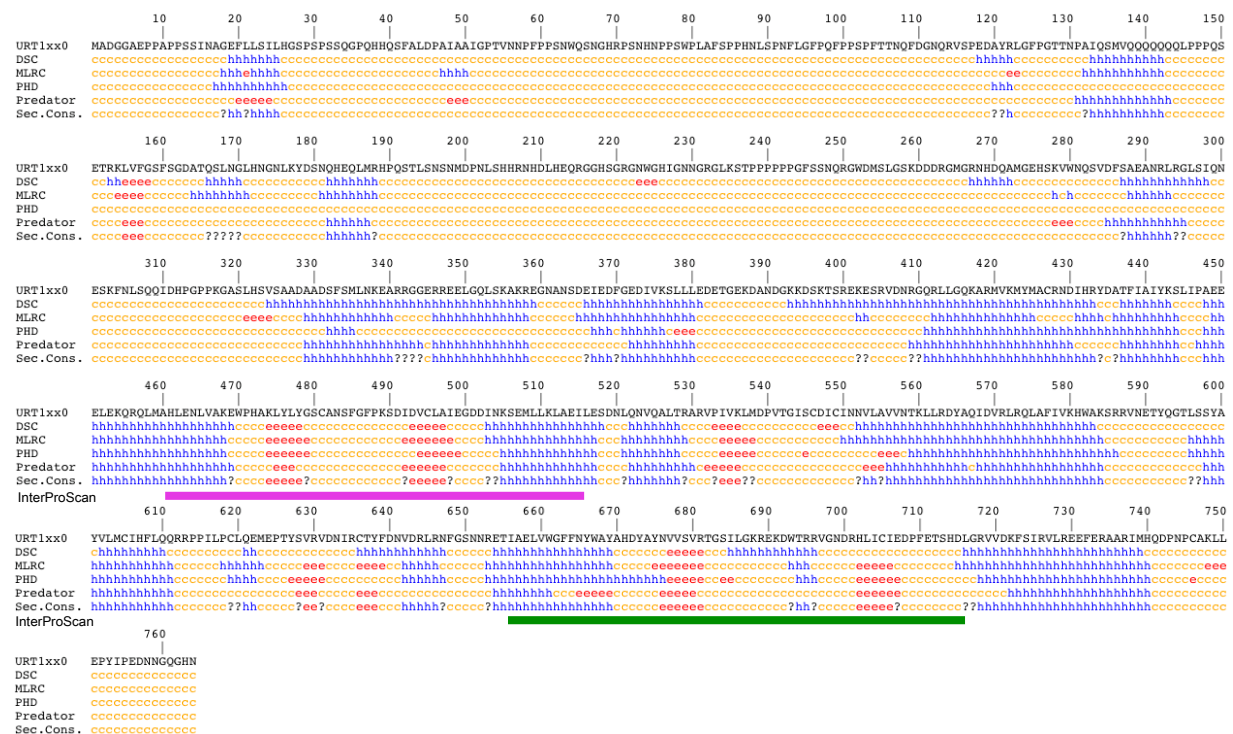
Figure 1.2 : Prédiction des structures secondaires de URT1
