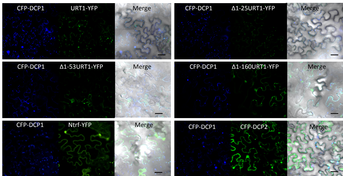
Figure 3.5: La co-expression de DCP1 ne change pas la localisation des différentes délétions de URT1
