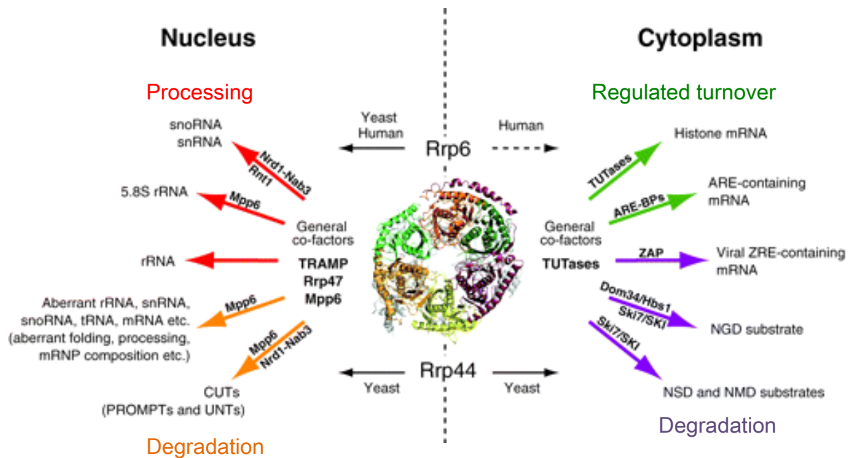
Figure 1A.5 : Les cofacteurs de l'exosome chez S. cerevisiae et l'homme selon la localisation de l'exosome
