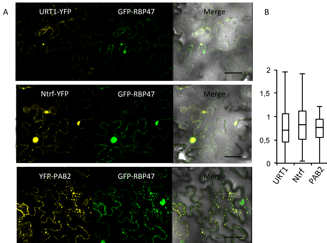
Figure 3.10 : Ntrf serait suffisant à la localisation de URT1 au niveau des granules de stress avec le marqueur des granules de stress RBP47
