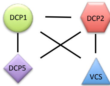
Figure 1A.8 : Les facteurs du complexe d'élimination de la coiffe chez A. thaliana
