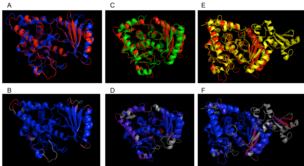
Figure 2B.3 : Alignement 3D du modèle du domaine nucléotidyltransférase de URT1 et des trois autres uridylyltransférases résolues au niveau atomique
