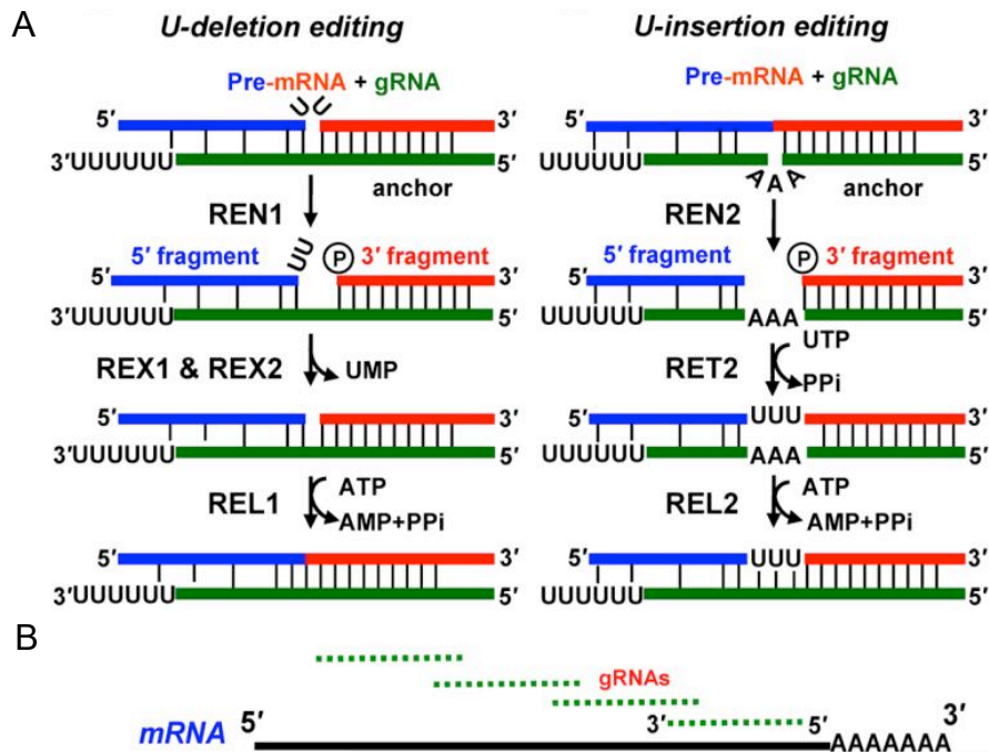
Figure IB.4 : L'édition des ARNm chez les trypanosomes par la délétion ou l'insertion d'uridines
