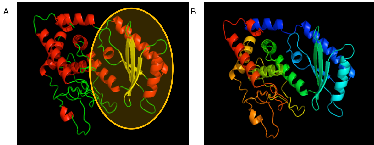
Figure 2B.5 : Représentation de la structure 3D modélisée du domaine nucléotidyltransférase de URT1
