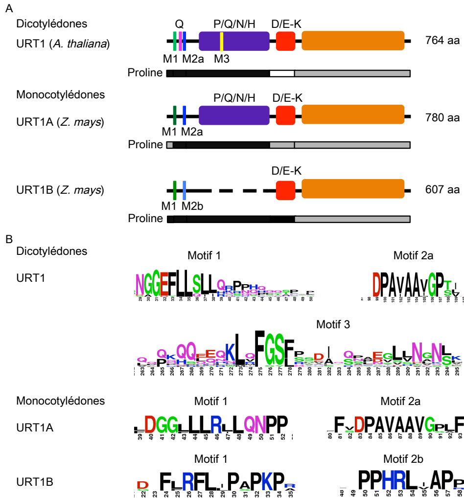
Figure 1.7: La région N terminale de URT1 contient des régions et des motifs conservés chez les Angiospermes
