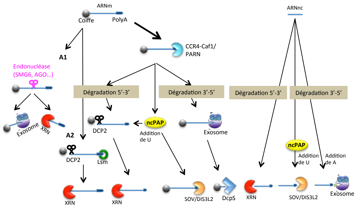
Figure IA.1 : Les voies principales de la dégradation des ARN
