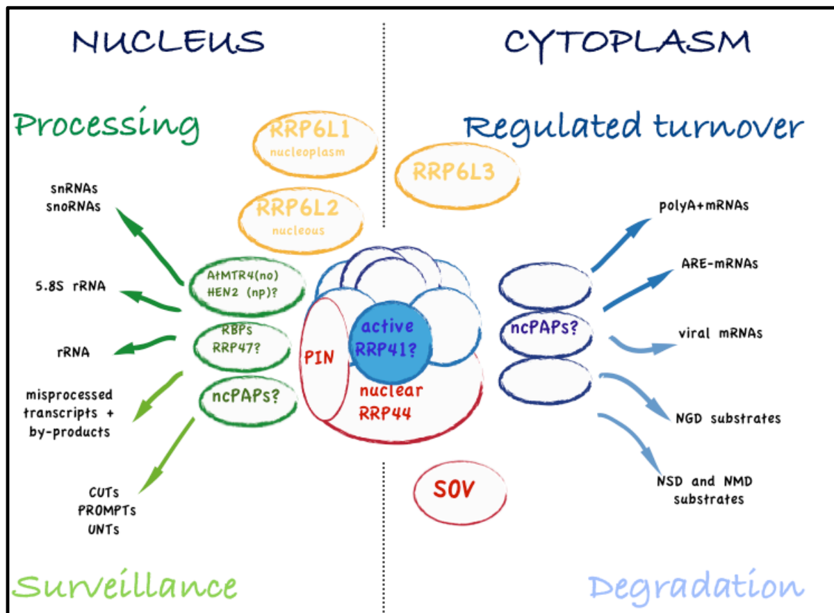
Figure 1A.6 : Les cofacteurs de l'exosome chez A. thaliana selon la localisation de l'exosome
