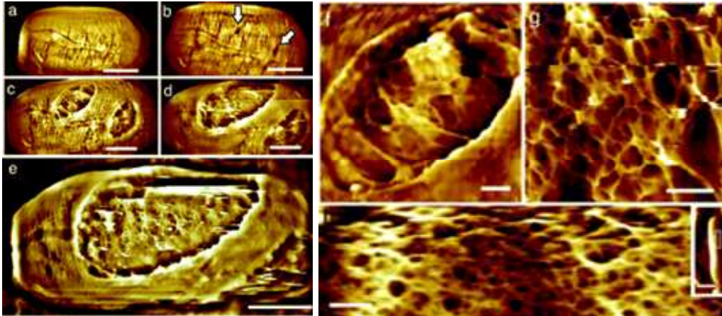
Figure 12 : Germination d'une spore de Bacillus atrophaeus observée par microscopie à force atomique. (a) 3h40, (b) 5h45, (c) 7h05, (d) 7h30, (e) 7h45, (f) 7h15, (g) 7h50, (h) surface d'une cellule végétative de B. atrophaeus . Echelle : 500 nm (a-e), 100 nm (f-h) et 1 µm (h encadré). D'après (Plomp et al. , 2007).
