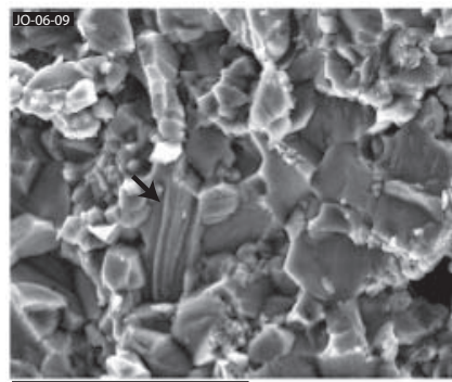
b-Cristaux de calcite microsparitique et sparitique ; notons les plans de clivage visibles sur le cristal repéré. (MEB).
