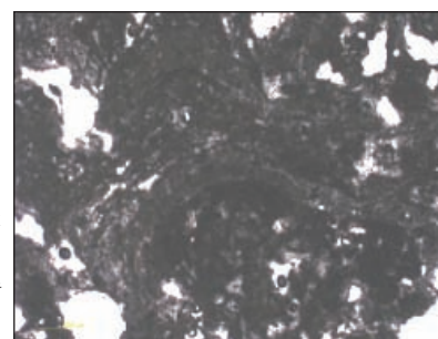
Figure B.89. Structures à croissance microbienne dans le travertin de l'état 4 de la salle T6.
