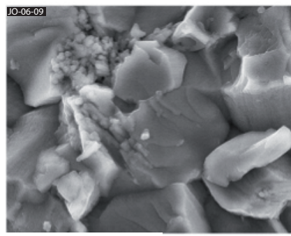
d-Bourgeonnement de nanoparticules responsables d'une précipitation micritique associée à une précipitation microsparitique périphérique (MEB).
