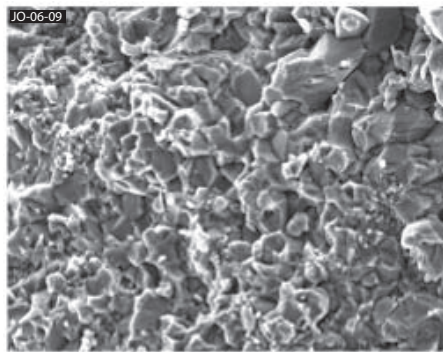
a-Cristallisation de calcite microsparitique dans un ciment micritique (MEB).
