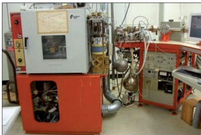
Figure A.63. Spectromètre de masse du laboratoire Leibniz- dation radiométrique et de recherche à l'Université de Kiel (Allemagne).
