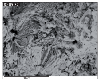
h-Précipitation radiale de cristaux fibreux autour de petites sphérules (MEB).
