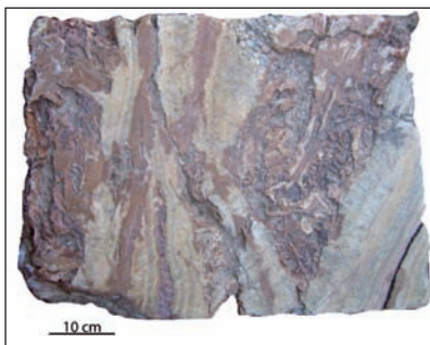
Figure B.23. Calcite filonienne de Jebel Oust.
