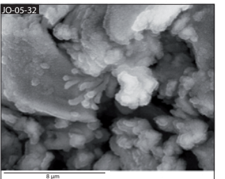
j-Bourgeoisement de nanoparticules bactériennes responsables d'une micritisation (MEB).
