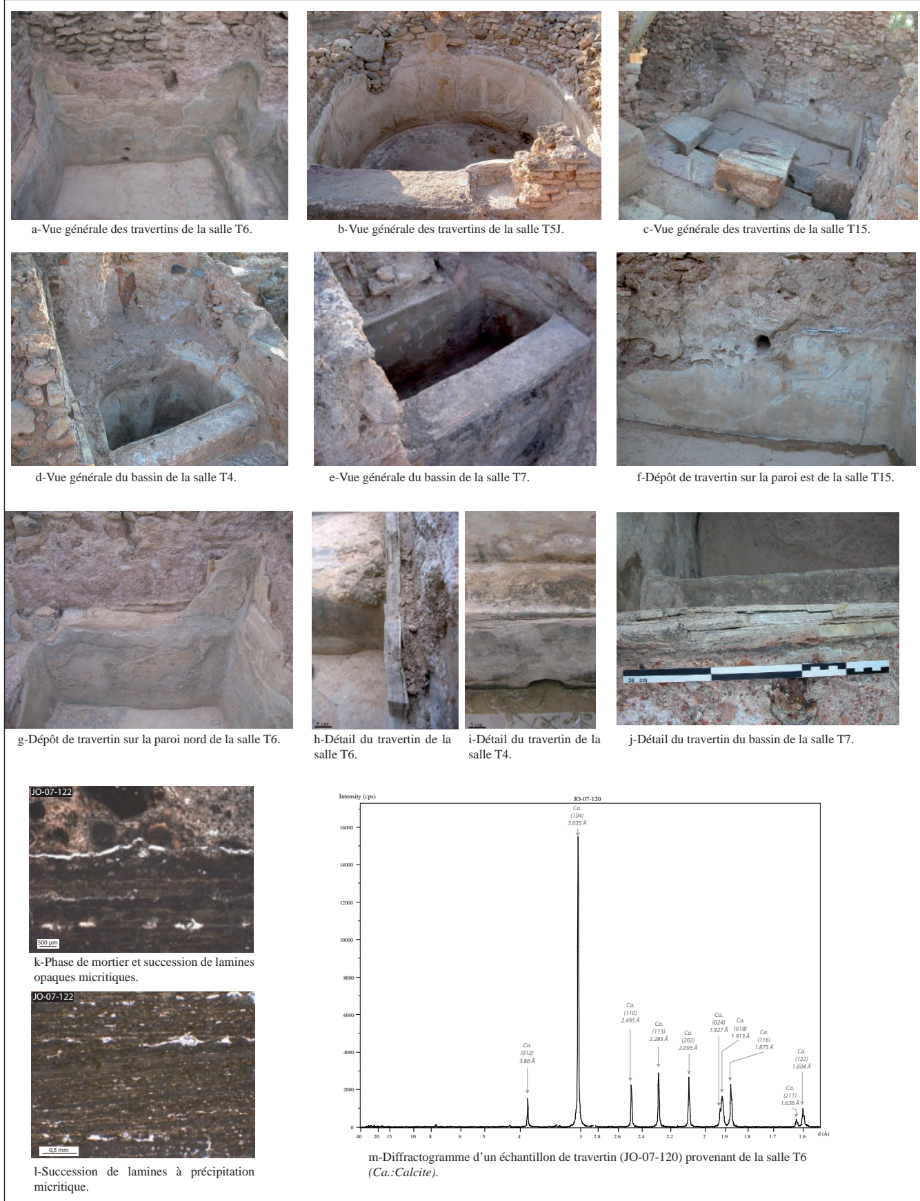
Figure B.73. Planche pétrographique du faciès D défini dans les thermes antiques de Jebel Oust ; voir les commentaires dans le texte.
