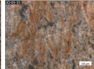
f-Cristaux sparitiques buissonnants ( shrub crystals ) (LP).
