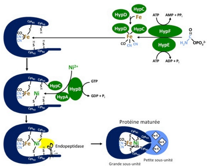
Figure 33 : Maturation et assemblage de la grande sous-unité (d'après O. Lentz)
