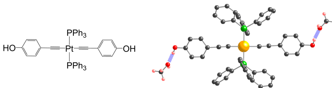
Figure 4 : Structure cristalline de 36. La liaison H entre les alcools est représentée en bleu hachuré. Les hydrogènes (excepté ceux des alcools et du MeOH) ont été omis par souci de clarté.
