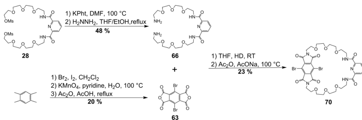
Schéma 2 : Synthèse du macrocycle pyroméllitique à anse amide.
