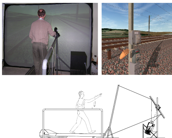
FIGURE 1.5 – Le simulateur FIACRE forme les agents de la SNCF à intervenir sur les voies ferrés. L’utilisation de ce système entraîne un gain de temps, et est plus rentable financièrement.
