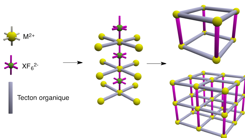
Figure 6 : Représentation schématique d'un processus possible pour la formation d'un réseau cuboïde à base de \text{MXF}_6 .
