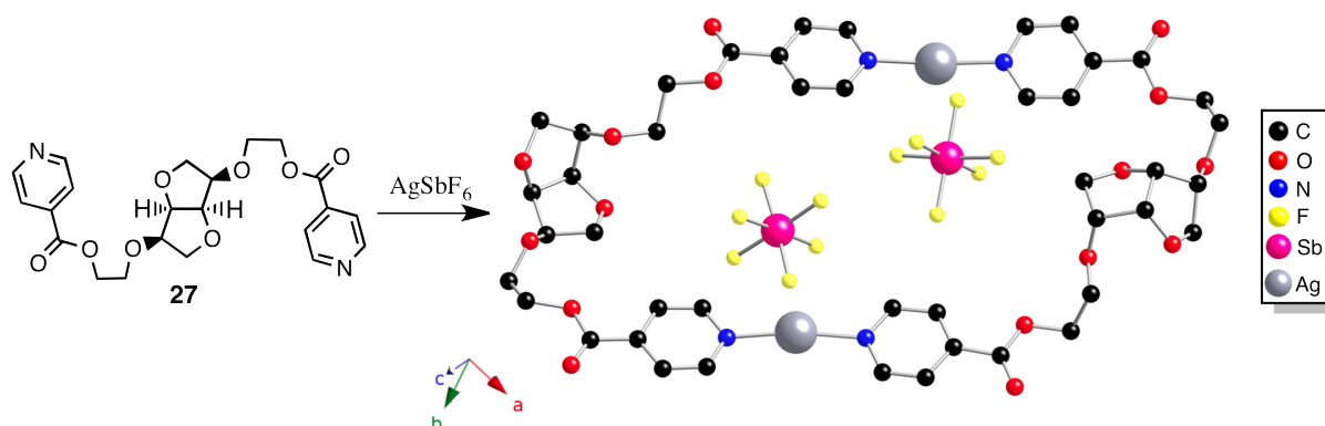
Figure 57 : Portion de la structure cristalline de 27 \cdot \text{AgSbF}_6 montrant le métallamacrocycle formé. Les atomes d'hydrogène sont omis par soucis de clarté.
