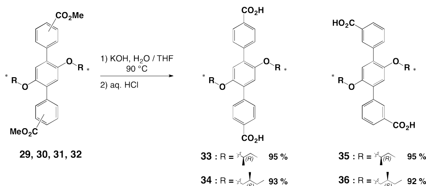
Figure 7 : Schéma réactionnel pour la préparation des tectons 33 à 36.
