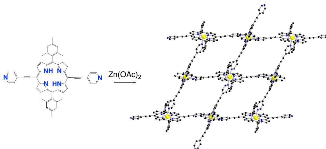
Figure 22 : Portion de la structure cristalline d'un réseau 2-D obtenu en combinant un tecton dérivé de porphyrine et un sel de Zn(OAc)_2 . [80]
