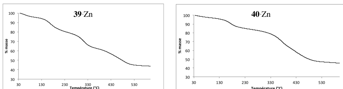
Figure 16 : Courbes des ATG de 39·Zn et 40·Zn .
