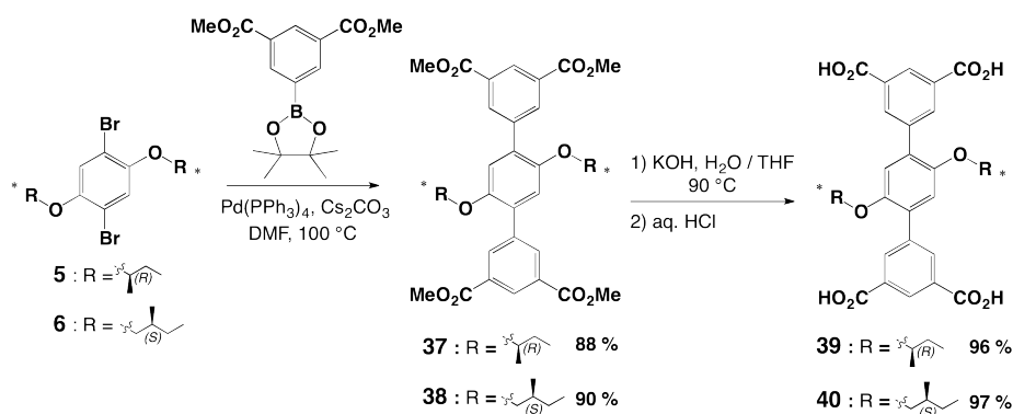
Figure 8 : Schéma réactionnel pour la préparation des tectons 39 et 40.
