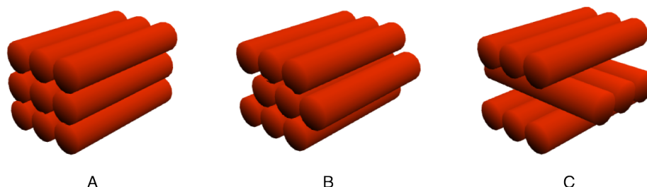
Figure 14 : Arrangements possibles de réseaux 1-D au sein d'un cristal en mode : carré (A), hexagonal (B) ou décalé (C).
