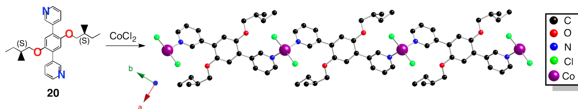
Figure 39 : Portion de la structure cristalline de 20 · \text{CoCl}_2 . Les atomes d'hydrogène et les molécules de solvant sont omis par soucis de clarté.
