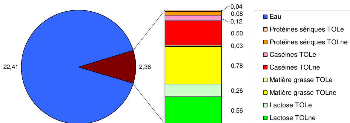
Figure 5-11 : Contribution des principaux composés hydrogénés à l'activité tritium du lait de Larçon prélevé le 4 juin 2012. Valeurs exprimées en Bq kg -1 de lait frais
