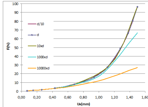
Figure 8.14.: Variation du paramètre d'incompressibilité d (la courbe avec losange correspond à la valeur de référence d = 10^{-4} \text{ MPa}^{-1} )
