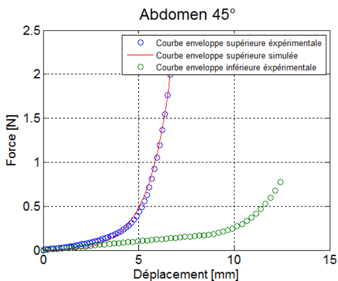
Figure 9.11.: Courbes force-déplacement expérimentales et simulées obtenues de l'essai d'extension de la peau saine de l'abdomen selon 45^\circ . Seule la courbe enveloppe inférieure et la courbe enveloppe supérieure sont présentées
