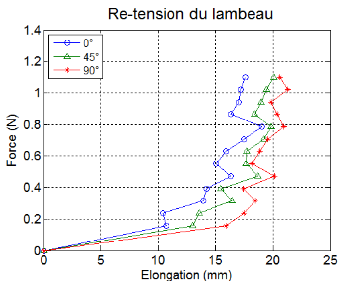
Figure 7.15.: Courbes force-élongation diamétrale du lambeau de peau pour les angles 0°, 45° et 90° tirées de 7.13 - chargement multiaxial
