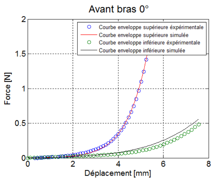
Figure 9.13.: Courbes force-déplacement expérimentales et simulées obtenues de l'essai d'extension de la peau saine de l'avant bras selon 0°. Seule la courbe enveloppe inférieure et la courbe enveloppe supérieure sont présentées
