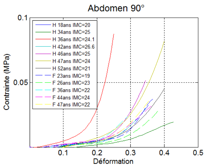
Figure 6.12.: Courbes contrainte-déformation de la peau de l'abdomen de tous les sujets volontaires chargée selon la direction cranio caudale
