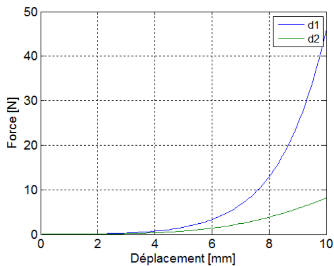
Figure 9.8.: Simulation d'un essai d'extension pour deux valeurs différentes du module d'incompressibilité d avec le modèle d'Ogden
