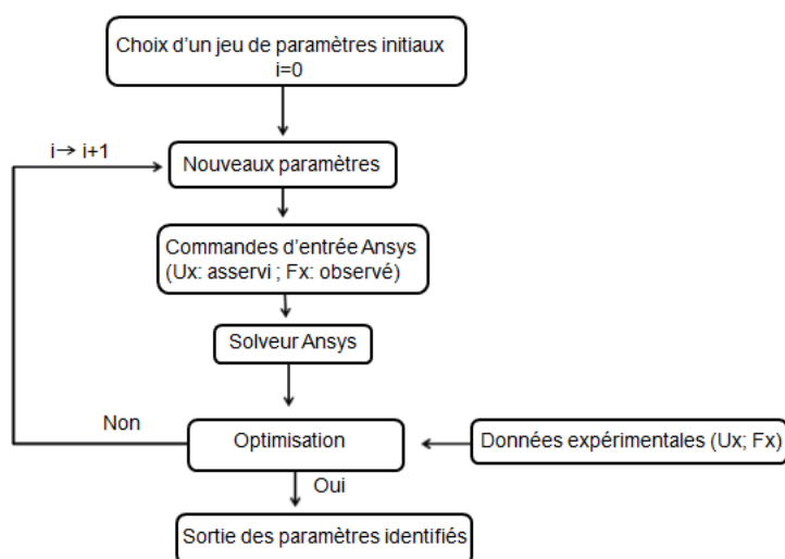
Figure 9.7.: Schéma du fonctionnement de MIC2M
