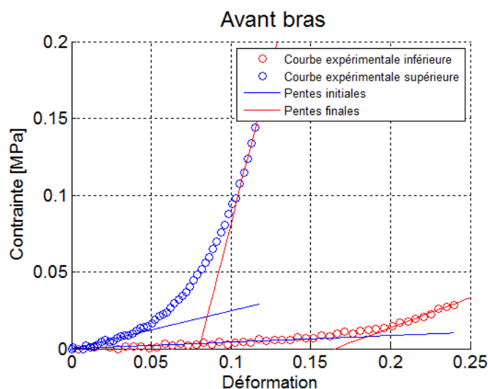
Figure 6.21.: Pentés initiales et pentés finales de la courbe supérieure et de la courbe inférieure représentant la famille des courbes contrainte-déformation de l'avant bras tous sujets, toutes zones et toutes orientations confondus
