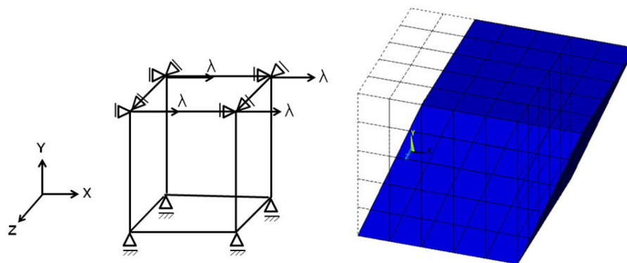
Figure 8.6.: Essai de cisaillement simple sous ANSYS® utilisateur pour un modèle néo-hookéen isotrope avec un matériau quasi-incompressible et une élongation imposée \lambda = 1.4 : conditions aux limites, maillage non déformé et maillage déformé
