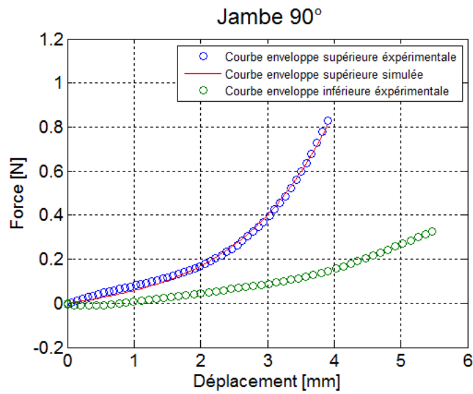
Figure 9.18.: Courbes force-déplacement expérimentales et simulées obtenues de l'essai d'extension de la peau saine de la jambe selon 90°. Seule la courbe enveloppe inférieure et la courbe enveloppe supérieure sont présentées
