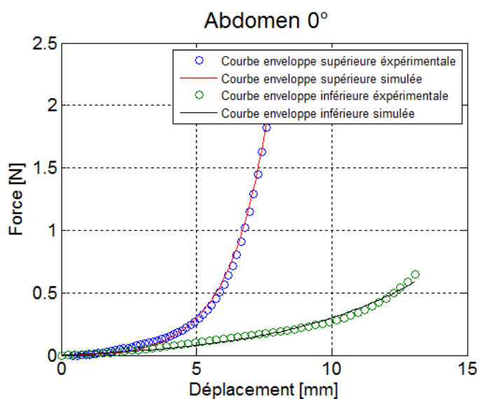
Figure 9.10.: Courbes force-déplacement expérimentales et simulées obtenues de l'essai d'extension de la peau saine de l'abdomen selon 0^\circ . Seule la courbe enveloppe inférieure et la courbe enveloppe supérieure sont présentées
