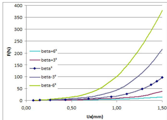
Figure 8.18.: Variation du paramètre \beta (la courbe avec losange correspond à la valeur de référence \beta = 41^\circ )
