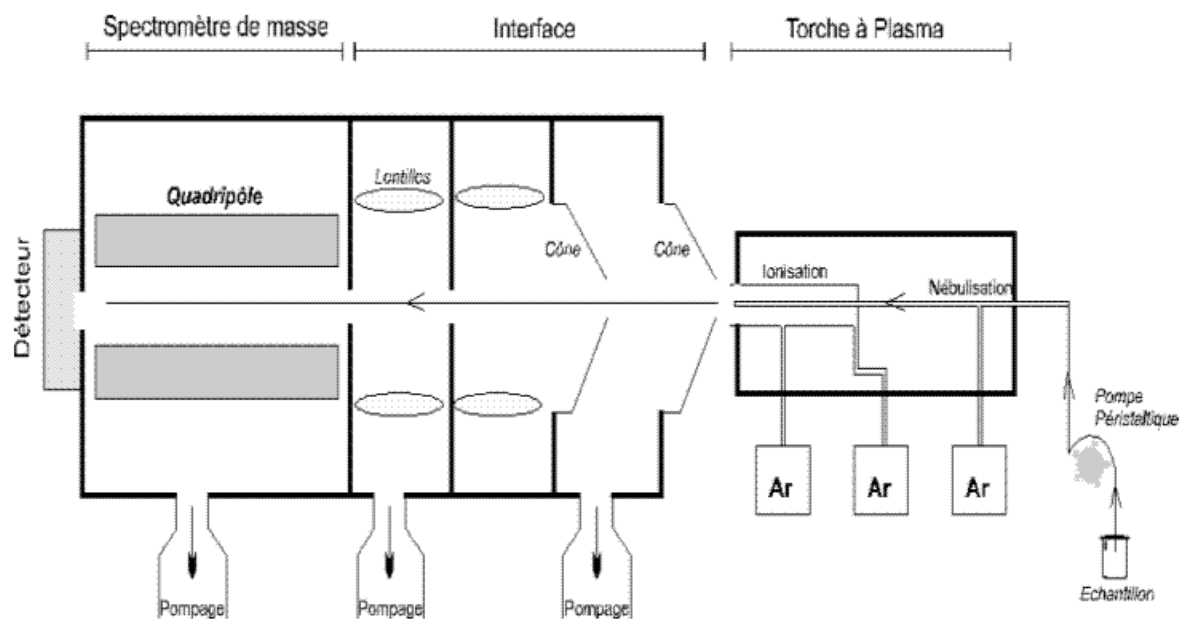
Figure 6 – Schéma conceptuel du spectromètre de masse ICP-MS.
