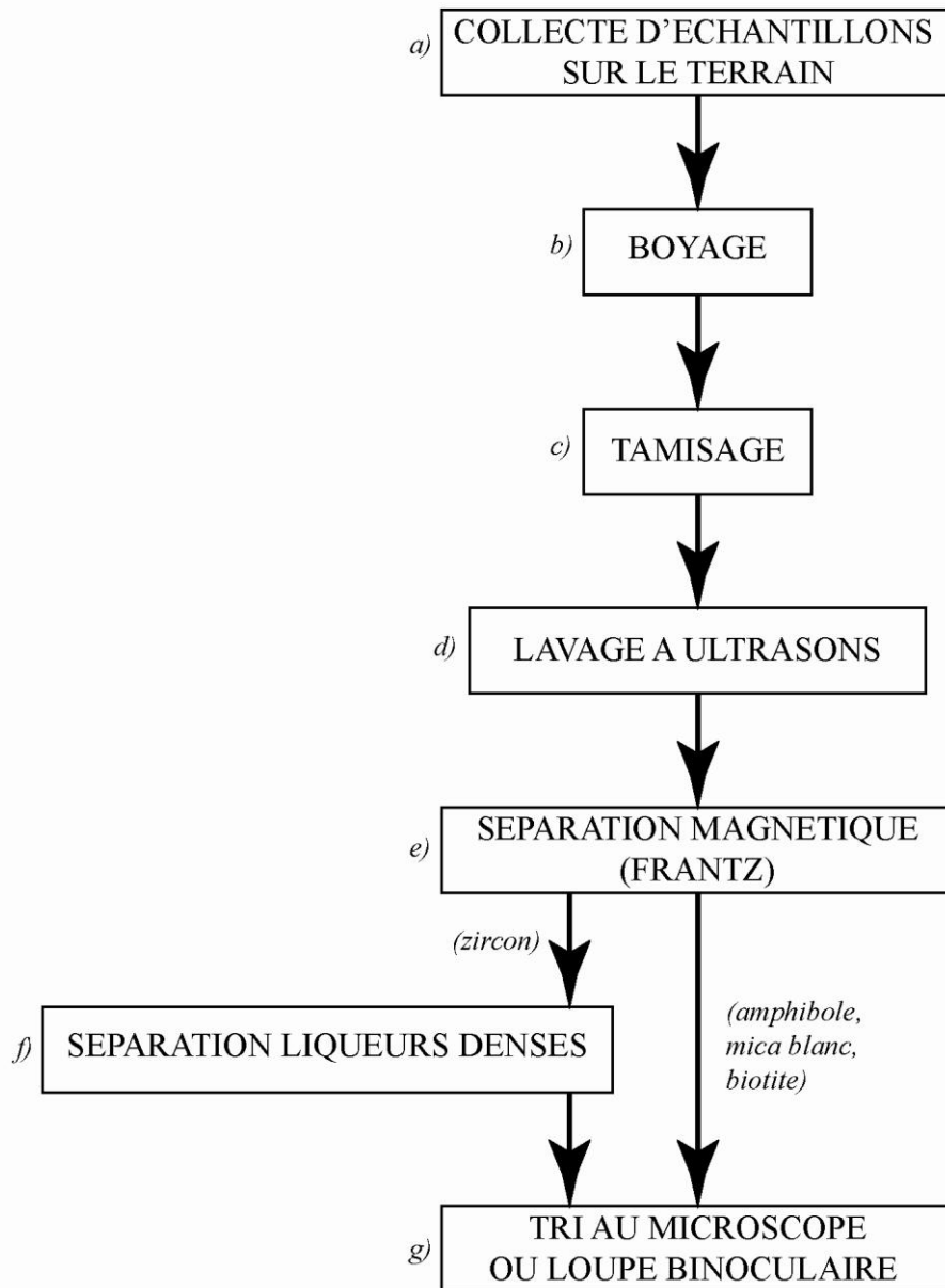
Figure 7 - Etapes successives de séparation minérales.
