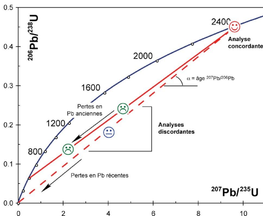
Figure 12 – Diagramme illustrant le principe d'utilisation de la courbe concordia.
