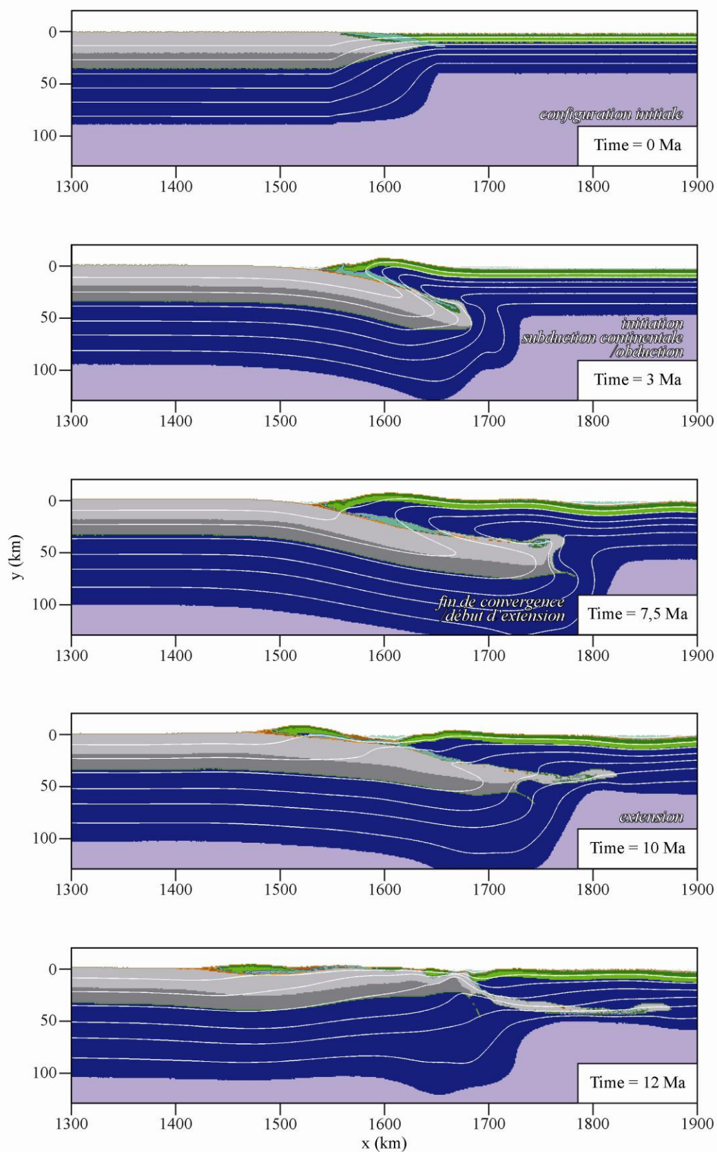
Figure 69 – Evolution temporelle du modèle 1 caractérisé par une lithosphère océanique vieille mais d'un âge thermique de 5 Ma sur la totalité de son étendu.
