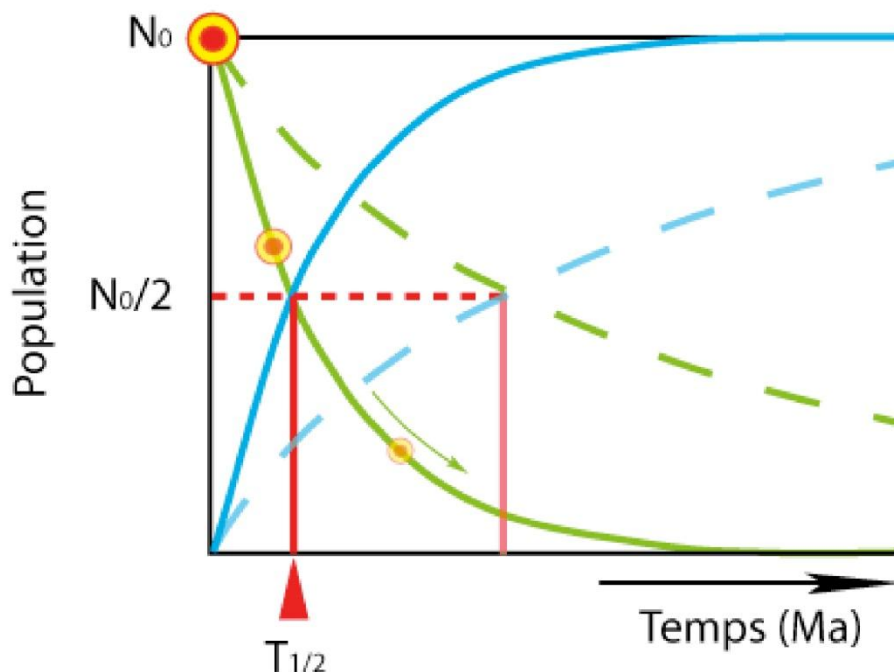
Figure 11 - Graphique représentant la décroissance de la quantité d'uranium et l'augmentation de plomb au cours du temps.
