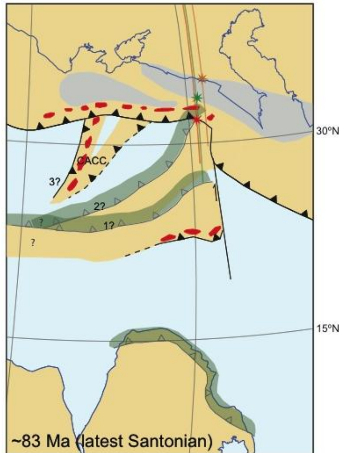
Figure 67 - Reconstitution du bloc TAP-SAB et des bassins océaniques environnants au Santonien, suite à l'obduction, d'après les données paléomagnétiques (Meijers et al., en révision). Les étoiles et marges d'erreur associées indiquent les paléo-latitudes des roches calcaires en discordance sur l'ophiolite obduite, mises en place juste après l'obduction). La position 1 décrit la position la plus méridionale et 2 la plus septentrionale du bloc TAP-SAB. L'obliquité du bloc est déduite d'une déclinaison de 40° impliquant une rotation de même valeur au moment de la fermeture de la branche nord de l'océan Téthys. La position 3 décrit la possibilité d'une zone de subduction très oblique, par rapport à la marge eurasiennne, en bordure occidentale du bloc de Kirshehir (ou Central Anatolian Crystalline Complex, CACC, Lefebvre, 2011).
