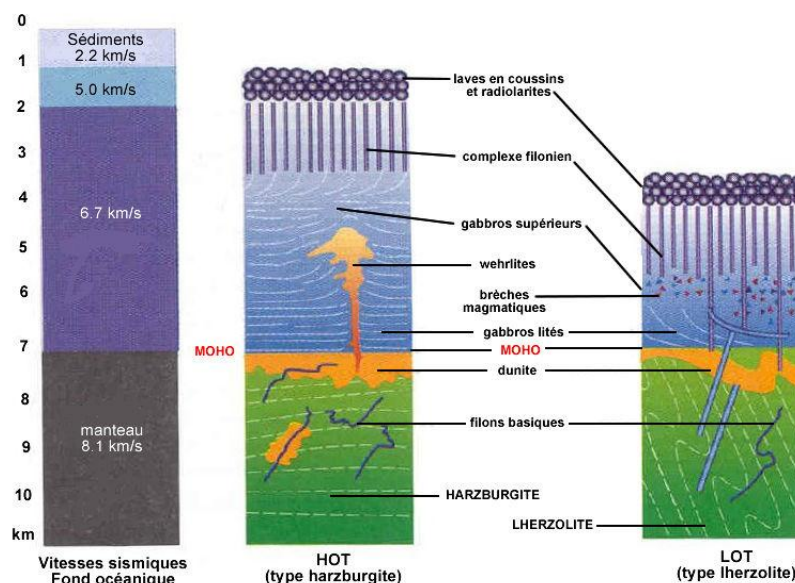
Figure 2 - Profils lithosphériques comparés HOT et LOT, et section définie par la sismique pour un fond océanique 'normal' composé d'une épaisse couche de produits d'origine magmatique (gabbros et basaltes), d'après Viissers & Nicolas (1995) et Nicolas (1997).
