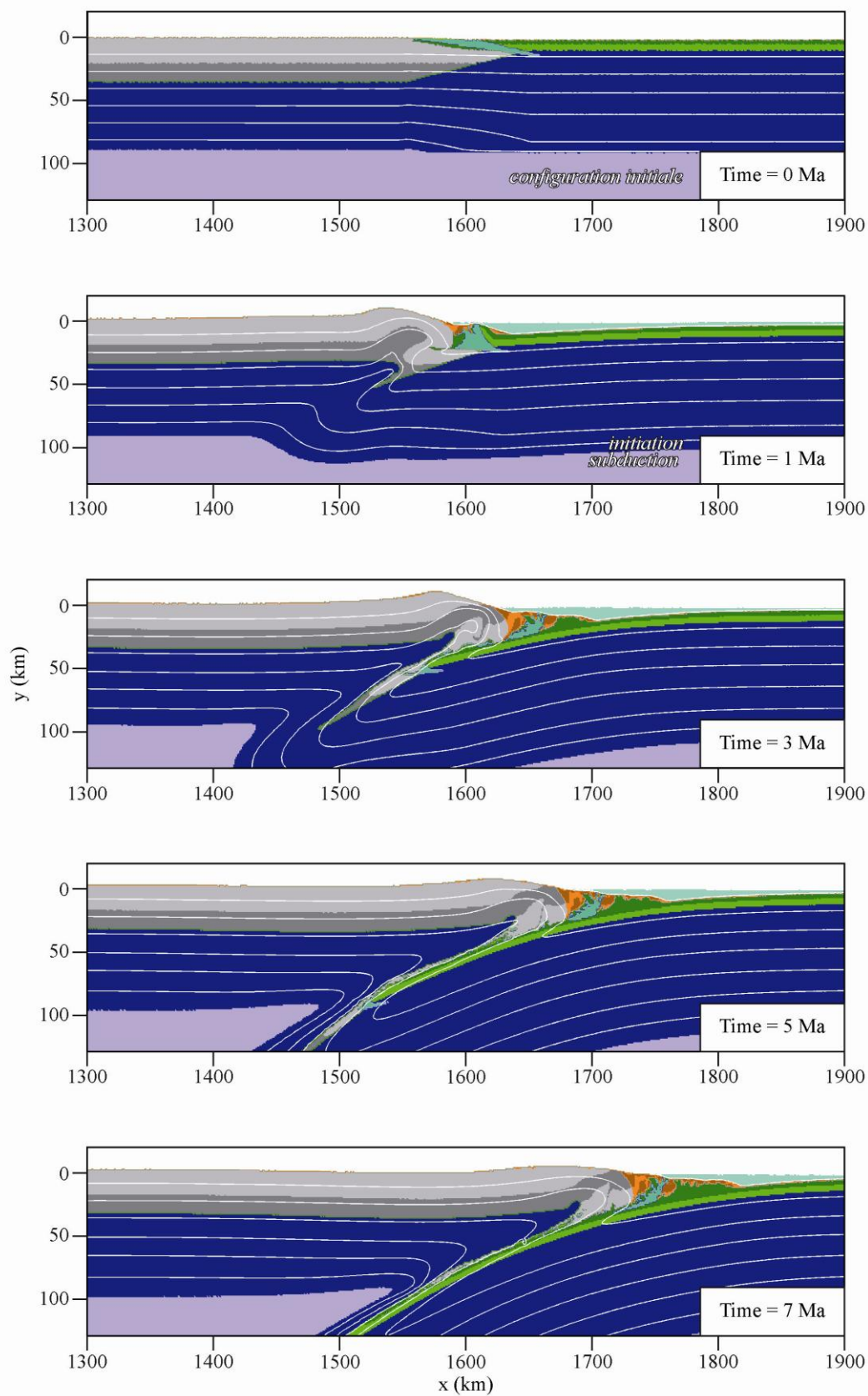
Figure 71 - Evolution temporelle du modèle 3 caractérisé par une lithosphère océanique vieille n'ayant pas subi de rajeunissement thermique.
