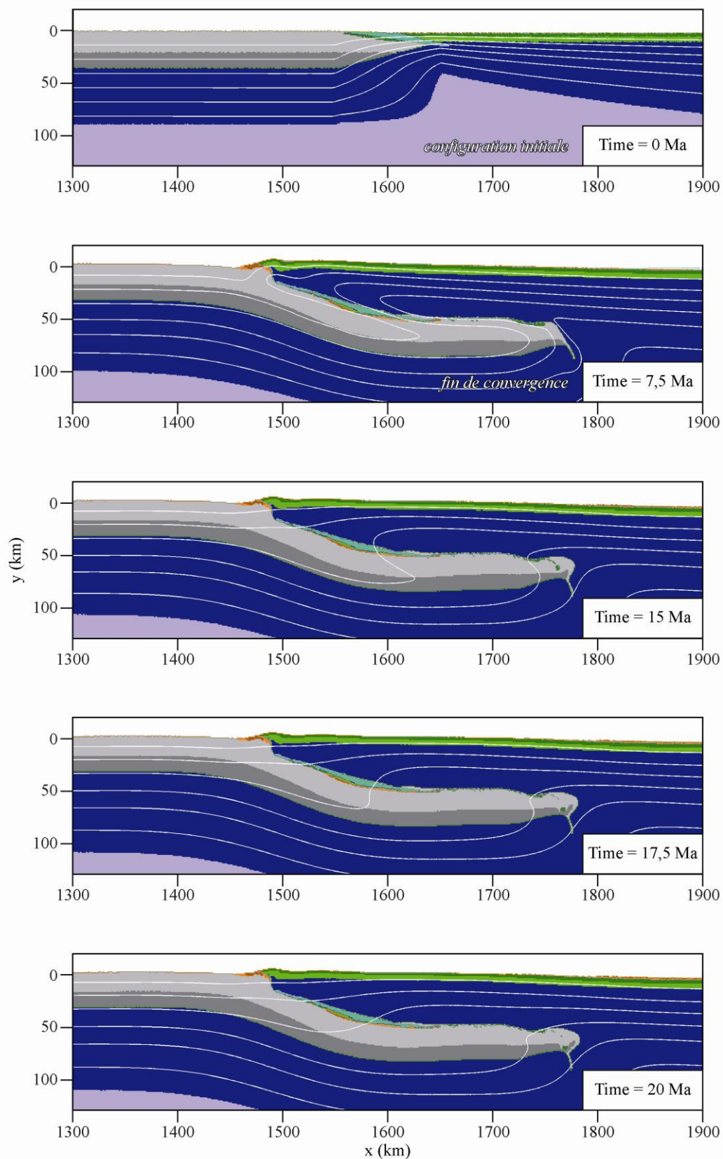
Figure 72 - Evolution temporelle du modèle 2 caractérisé par une lithosphère océanique vieille mais d'un âge thermique de 5 Ma sur restreint à un domaine proche de la marge continentale. Ce modèle se distingue du modèle 2 par l'absence de la pas d'extension post-obduction.
