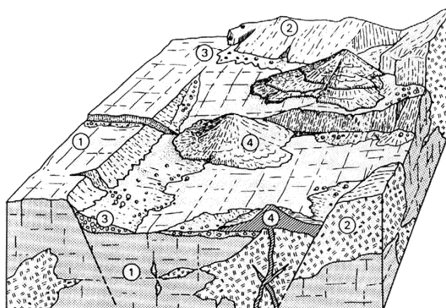
Figure 3 - Schéma d'une ophiolite de ride lente (LOT), d'après l'observation des ophiolites alpines (Lagabrielle, 1987; Lagabrielle et al. , 1989; Lagabrielle & Lemoine, 1997). 1, lherzolite serpentinisée (manteau) ; 2, gabbros ; 3, brèches (talus de debris) ; 4, volcans à laves en coussins.
