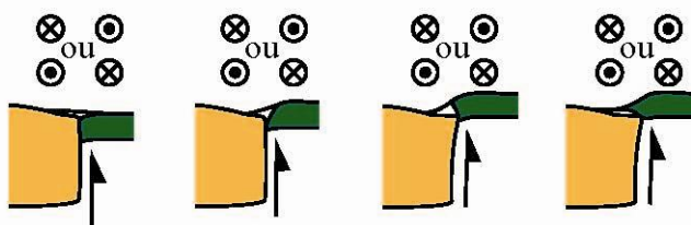
Figure 4 - Schémas illustrant les quatre catégories d'obduction.
