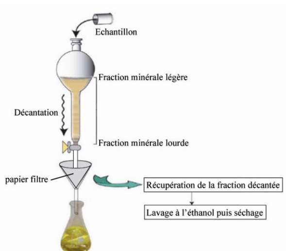
Figure 9 - Dispositif de séparation par liqueur dense.
