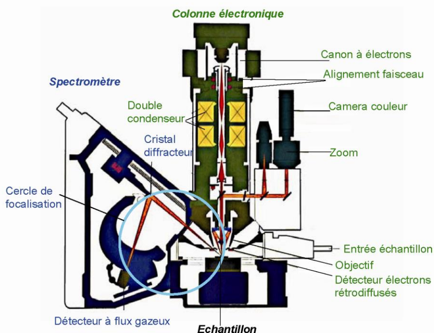
Figure 5 - Schéma des composants d'une microsonde électronique.
