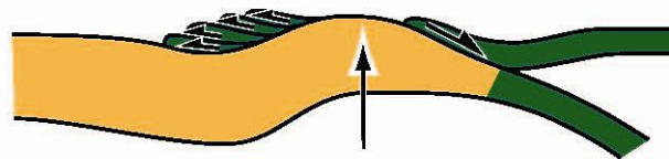
(2) glissement gravitaire/obduction passive
