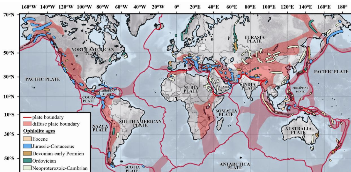
Figure 1 – Distribution des ophiolites Neoproterozoïque et Phanérozoïque d’après Vaughan & Scarrow (2003), modifiée.
