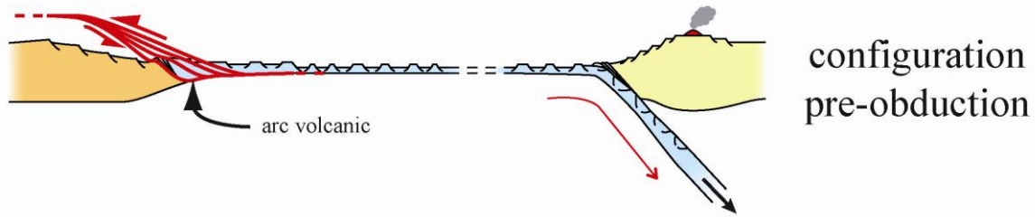
Figure 68 – Représentation schématique de la configuration pré-obduction (en haut) et la distribution des champs de composition de référence utilisée au cours des modélisations (en bas).
