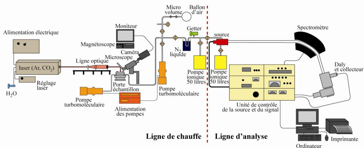
Figure 10 - Schéma du dispositif d'analyse ^{40}\text{Ar}/^{39}\text{Ar} .
