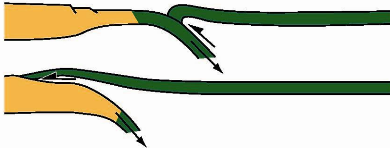
(2) glissement gravitaire/obduction passive
