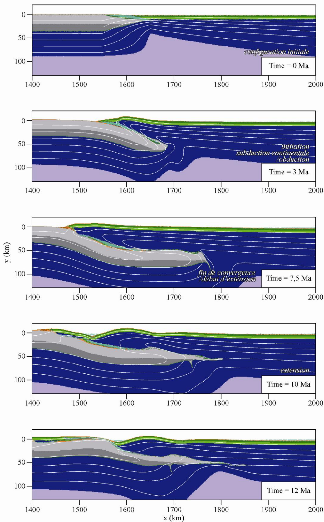
Figure 70 - Evolution temporelle du modèle 2 caractérisé par une lithosphère océanique vieille mais d'un âge thermique de 5 Ma sur restreint à un domaine proche de la marge continentale.
