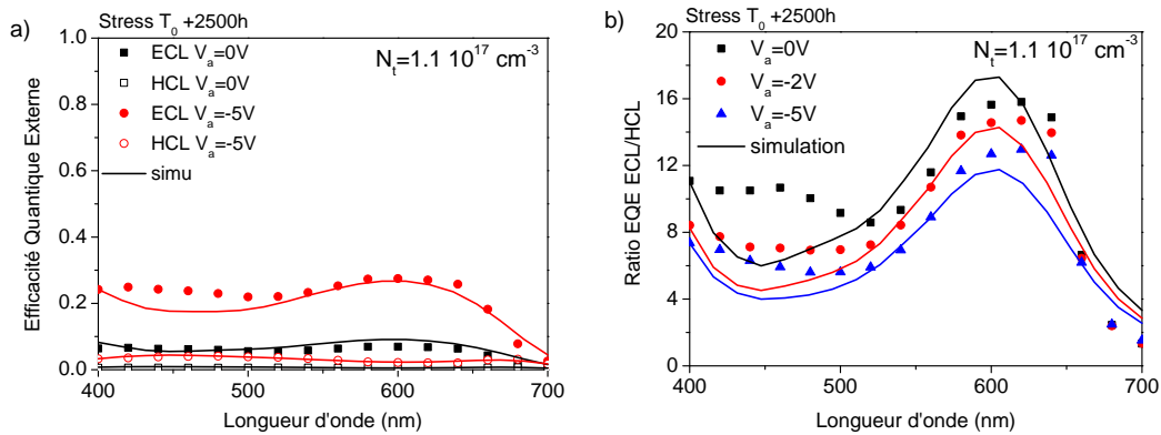
FIGURE 3.43 – Après 2500 heures de stress, mesures d'efficacité quantique externe (0 V et -5 V) a) et calcul de leur ratio entre les deux côtés d'éclairément (ECL et HCL) b). Les courbes d'efficacité ont été simulées avec une densité de pièges profonds accepteurs de 1,1 \times 10^{17} \text{ cm}^{-3} .
