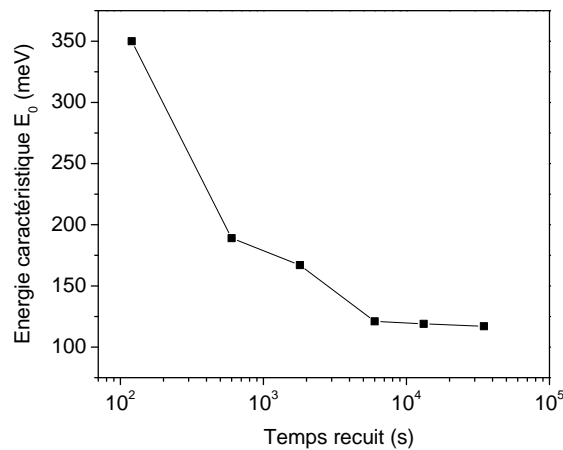
FIGURE 2.39 – Extraction de l'énergie caractéristique E_0 des queues de bande en dessous de 1,6 eV en fonction du temps de recuit de la couche active.
