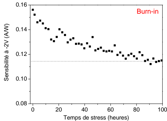
FIGURE 3.62 – Mesures de sensibilité en régime inverse ( V_a = -2 V) au cours du stress lumineux et électrique d'une photodiode organique (condition standard).
