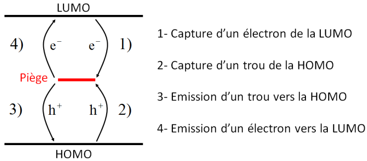
FIGURE 1.46 – Illustration des processus de capture et d'émission de charges par un état de gap, décrits par le formalisme de Shockley Read Hall.
