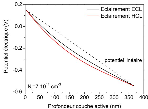
FIGURE 3.55 – Simulation numérique du potentiel électrique dans la photodiode avec une densité de pièges accepteurs de 7 \times 10^{14} \text{cm}^{-3} pour un éclairément de 10^{-3} AM 1.5.
