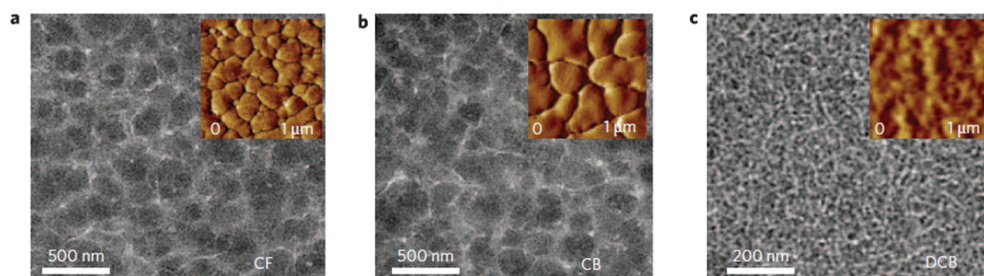
FIGURE 1.13 – Caractérisation MET d'un mélange PCDTBT :PC 70 BM dissout dans différents solvants : a) CF, b) CB et c) DCB. Images MET extraites de [Park 2009].
