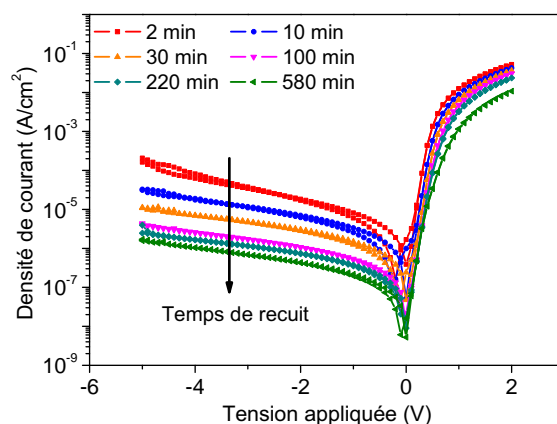
FIGURE 2.30 – Caractéristique courant tension dans l'obscurité pour les différents temps de recuits à 85°C. Contrairement au photocourant, le courant d'obscurité en régime inverse décroît continuellement au cours des différentes étapes de recuit et ce sur plusieurs décades.
