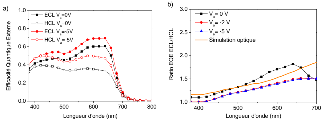
FIGURE 3.51 – Mesures d'efficacité quantique externe (0 V et -5 V) a) et calcul de leur ratio selon les deux côtés d'éclairage (ECL et HCL) b).
