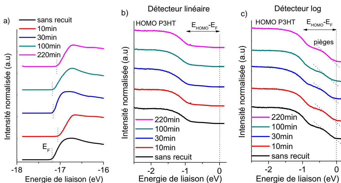
FIGURE 2.44 – Distribution énergétique du signal mesuré par UPS de la couche de P3HT pour différents temps de recuit. Le bord du signal au niveau duquel est extrait le niveau de Fermi est donné en figure a). En figure b) et c) le spectre est centré sur la HOMO du P3HT avec respectivement l'utilisation du détecteur linéaire et du détecteur log. Sur la figure .c, les queues de bande sont indiquées par une ligne en pointillé. Le décalage sur l'échelle des ordonnées est arbitraire et permet une meilleure visualisation des mesures.
