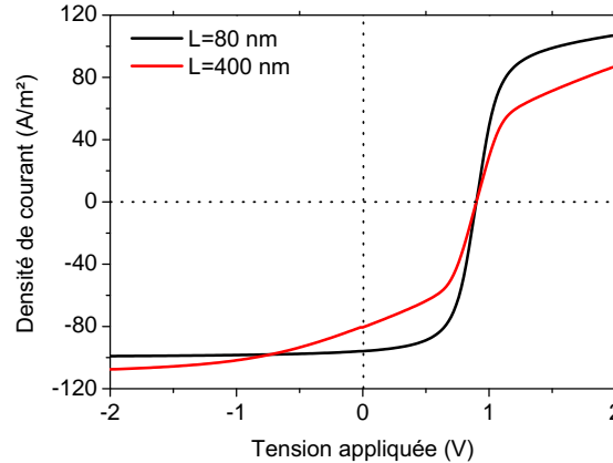
FIGURE 1.35 – Simulation numérique du photocourant dans une structure directe sous éclairage AM 1.5 avec les paramètres de simulation suivants : E_g=1,6 eV, \Phi_C-\Phi_{SC} = -0,4 eV, \Phi_A-\Phi_{SC} = 0,5 eV, \mu_{n,p} = 5 \cdot 10^{-4} \text{ cm}^2 \text{ V}^{-1} \text{ s}^{-1} , ITO=120 nm, PEDOT=40 nm, Alu=100 nm. Deux épaisseurs de couche actives sont simulées : 80 nm et 400 nm.
