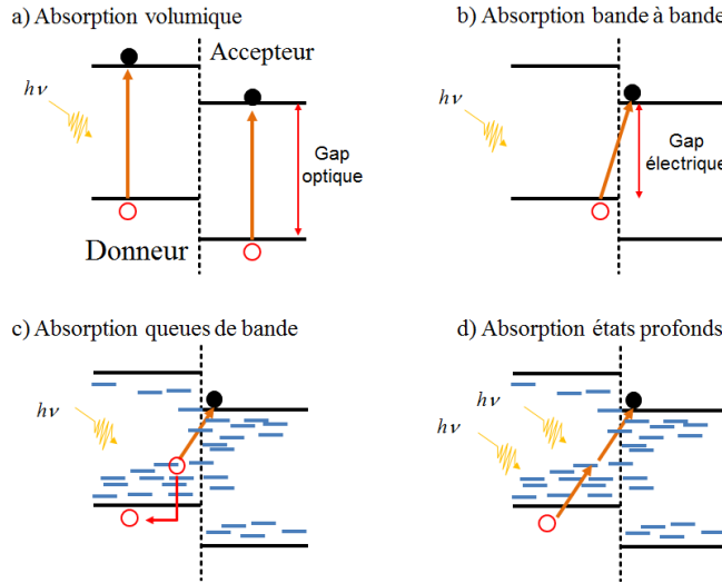
FIGURE 2.5 – Illustration des différentes transitions optiques dans les photodiodes organiques : a) absorption en volume, b) absorption bande à bande, c) absorption dues aux queues de bande d) absorption des états profonds par contribution de plusieurs photons.
