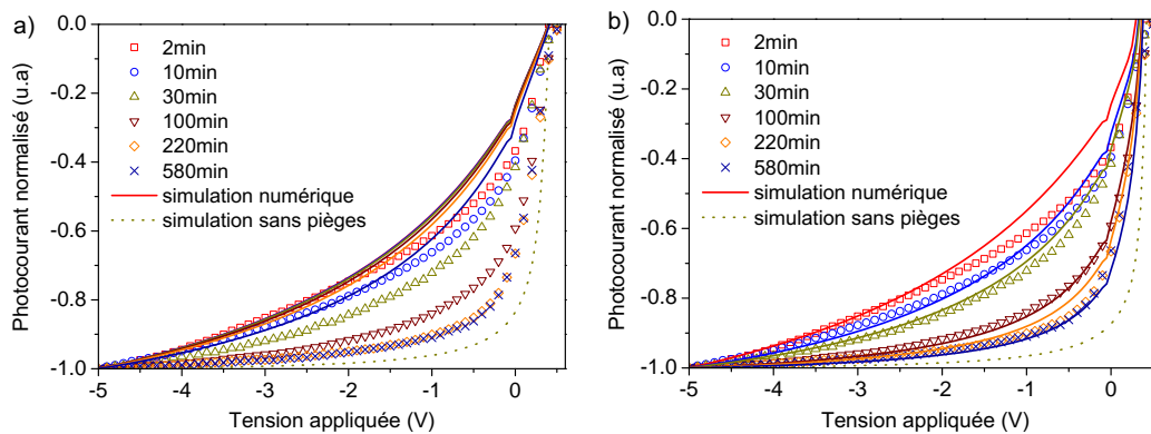
FIGURE 2.49 – Comparaison du photocourant expérimental en fonction de la tension de polarisation avec les résultats de la simulation numérique. Seule l'évolution de la taille des domaines est prise en compte a) tandis que les queues de bande extraites à partir de la réponse spectrale de la photodiode ont été implémentées pour prendre en compte la variation du taux de recombinaisons assistées par pièges en b).
