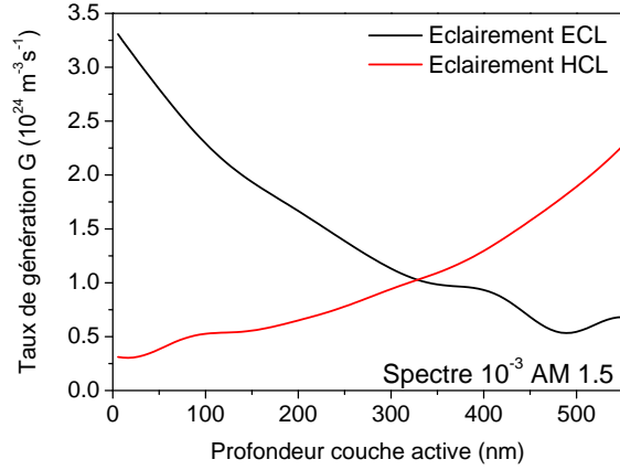
FIGURE 3.15 – Simulation optique du taux de génération G de paires électron-trou dans la couche active de la photodiode d'épaisseur 550 nm.
