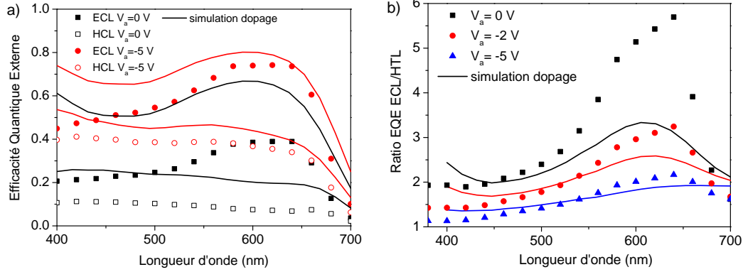
FIGURE 3.20 – Simulation numérique des EQE pour les deux côtés d'éclairage à différentes polarisations en régime inverse en tenant compte d'une densité de dopage de type P de 3,0 \times 10^{15} \text{cm}^{-3} a) et du ratio d'EQE entre les deux côtés d'éclairage b). Les courbes simulées sont comparées aux caractéristiques expérimentales.
