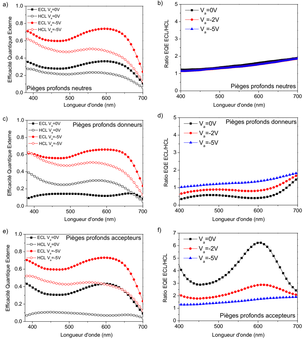
FIGURE 3.17 – Simulation numérique des EQE pour les deux côtés d'éclairément à différentes polarisations en régime inverse, en tenant compte d'une densité de pièges profonds de 3,0 \times 10^{15} \text{cm}^{-3} . Les trois types de pièges sont simulés : neutre, donneur et accepteur.
