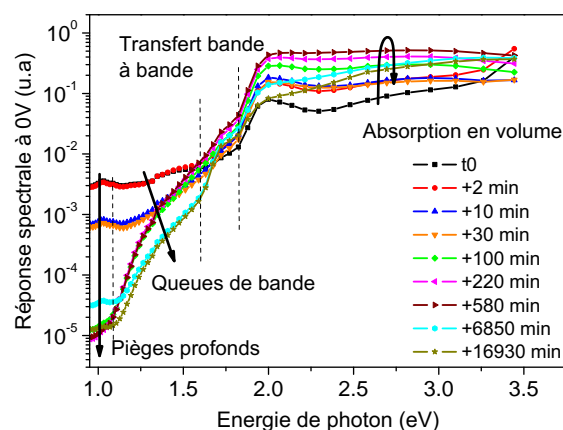
FIGURE 2.38 – Réponse spectrale de la photodiode organique à 0 V en fonction de l'énergie du photon incident. Un détecteur silicium a été utilisé jusqu'à 900 nm (1,37 eV) et un autre, InGaAs jusqu'à 1400 nm (0,89 eV). Les différentes transitions optiques sont identifiées sur le graphique.
