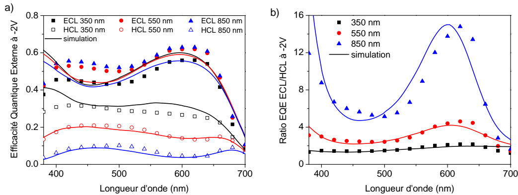
FIGURE 3.60 – Simulation numérique des EQE a) et de leur ratio respectif b) à -2 V selon les deux côtés d'éclairage pour 3 épaisseurs différentes de couche active en P1:PC 60 BM : 350 nm, 550 nm et 850 nm. Une concentration de pièges profonds accepteurs de 5,0 \times 10^{15} \text{ cm}^{-3} est prise en compte.
