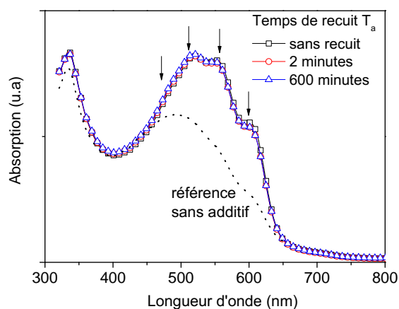
FIGURE 2.27 – Mesure de l'absorption de la couche active P3HT:PC 60 BM par spectrométrie UV-visible. L'ordre cristallin mesuré par les pics d'absorption du P3HT (flèches) reste inchangé au cours des différents recuits. Un spectre d'absorption d'une même couche sans additif et sans recuit est donné (courbe en pointillés).
