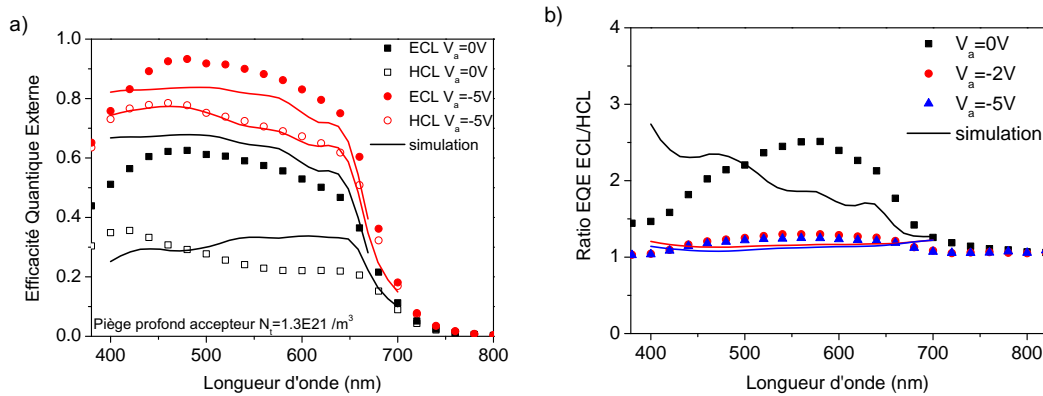
FIGURE 3.33 – Simulation numérique des EQE des photodiodes organiques en structure directe a) et leur ratio selon le côté d'éclairage b).
