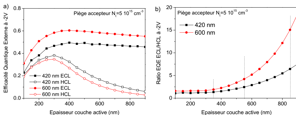
FIGURE 3.61 – Simulation numérique des EQE (à 420 et 600 nm) a) et de leur ratio respectif b) à -2 V selon les deux côtés d'éclairage en fonction de l'épaisseur de la couche active. Une concentration de pièges profonds accepteurs de 5,0 \times 10^{15} \text{ cm}^{-3} est prise en compte.
