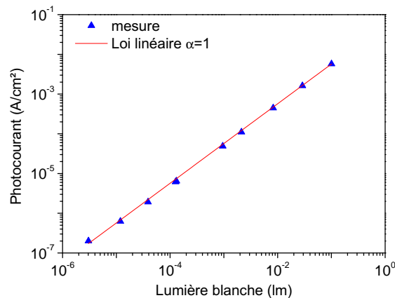
FIGURE 1.30 – Mesure de linéarité d'une photodiode en P3HT:PC 60 BM en polarisation nulle. L'éclairément est réalisé par une lampe halogène et la puissance lumineuse est diminuée par des filtres neutres.
