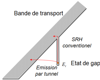
FIGURE 2.58 – Illustration du mécanisme d'émission tunnel d'un état de gap comparé au mécanisme thermique utilisé dans le formalisme SRH.
