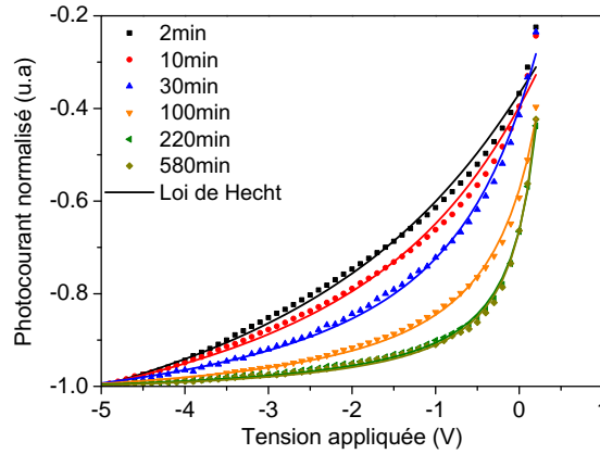
FIGURE 2.36 – La formule de Hecht est ajustée sur les courbes de photocourant normalisées en fonction du temps de recuit.
