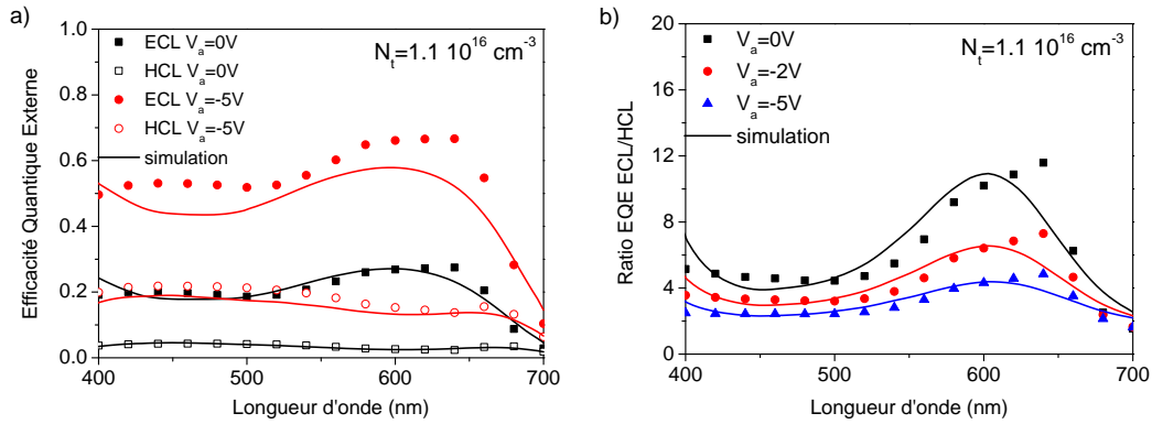
FIGURE 3.42 – Mesures d'efficacité quantique externe (0 V et -5 V) pour les deux côtés d'éclairément respectifs (ECL et HCL) a) et calcul de leur ratio d'EQE b). Les courbes d'efficacité ont été simulée avec une densité de pièges profonds accepteurs de 1,1 \times 10^{16} \text{ cm}^{-3} .
