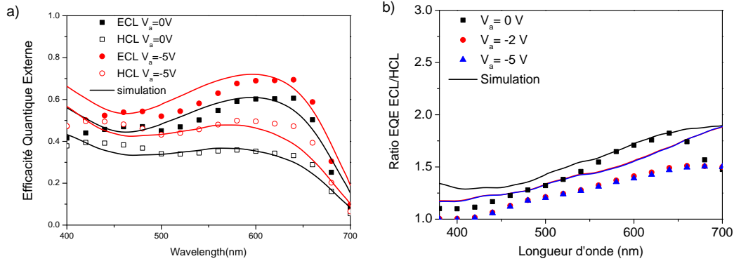
FIGURE 3.54 – Mesures d'efficacité quantique externe (0 V et -5 V) pour les deux côtés d'éclairément respectifs (ECL et HCL) a) et calcul du ratio d'efficacité entre l'éclairément côté cathode et l'éclairément côté anode b). Les courbes expérimentales sont modélisées en fixant un taux de pièges profonds de type accepteurs de 7 \times 10^{14} \text{cm}^{-3} .
