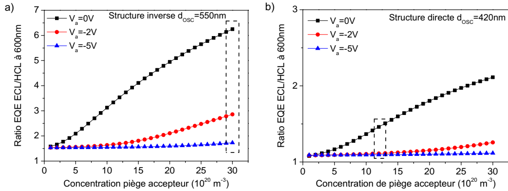
FIGURE 3.32 – Simulation numérique du ratio d'EQE entre ECL et HCL à 600 nm pour des polarisations externes de 0, -2 et -5 V en fonction de la concentration de pièges accepteurs pour la structure inverse a) et la structure directe b) de l'étude.
