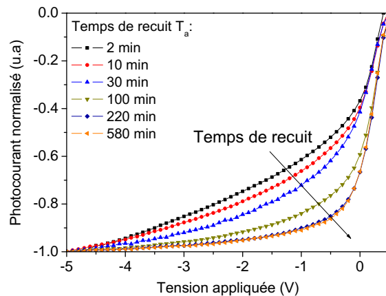
FIGURE 2.35 – Mesure du photocourant de la photodiode, normalisé par sa valeur à -5 V, en fonction de la tension de polarisation sous un éclairage en lumière blanche de 250 W/m 2 .
