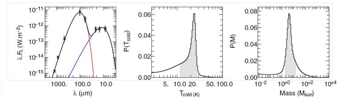
FIGURE 3.1: Exemple d'un fit de SED, extrait de Hill et al. (2009). Le fit en lui-même est représenté sur la figure de gauche (fit à deux composantes, dont la composante rouge contraint la masse du cœur dense), tandis que la figure centrale (resp. de droite) représente la dispersion de température (resp. de la masse) associée au fit de la composante froide.
