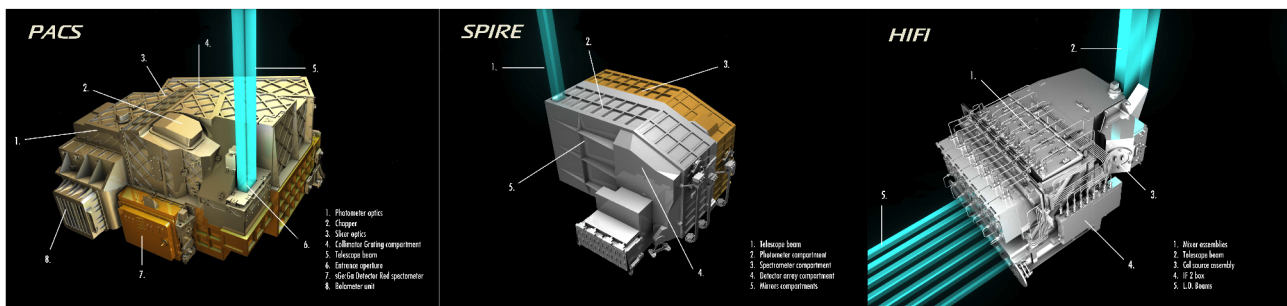
FIGURE 2.13: Vue des trois instruments embarqués sur Herschel . De gauche à droite : PACS, SPIRE et HIFI. Crédit : ESA.
