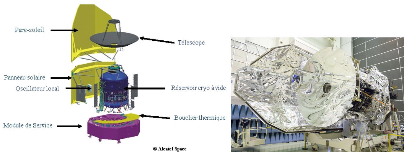
FIGURE 2.12: Gauche : Vue éclatée du satellite Herschel . Droite : Photo du satellite Herschel en salle blanche, avant le lancement. Crédit : ESA .
