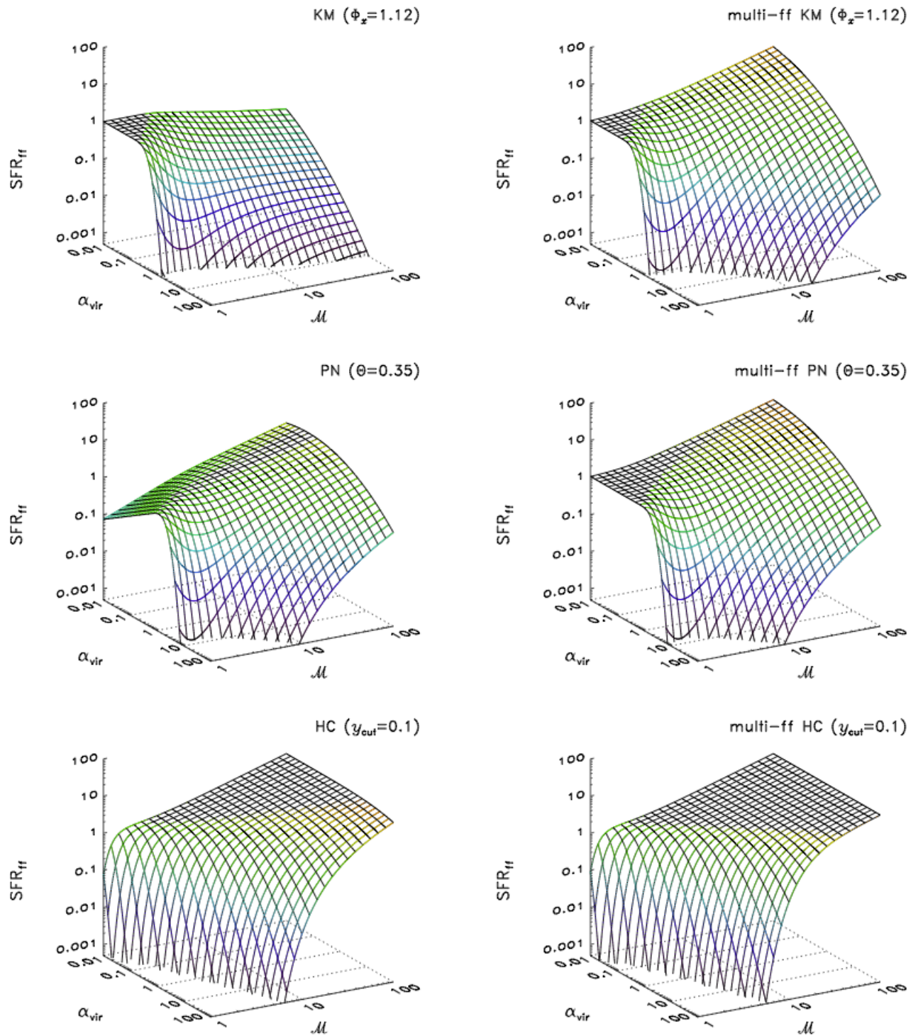
FIGURE 3.7: Comparaison des modèles analytiques de KM05, PN11 et HC11. Les trois figures de gauche montrent les modèles originaux des auteurs, les trois de droite montrent ces mêmes modèles dans leur version multi freefall. Extrait de Federrath & Klessen (2013).
