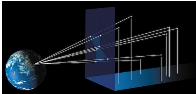
FIGURE 3.13: Exemple des effets de projection avec la constellation d'Orion, pour laquelle la distance précise des étoiles a pu être mesurée grâce à la méthode des parallaxes. Dans la 'réalité' de l'Univers à trois dimensions, les étoiles qui composent cette constellation ne sont pas du tout dans un même plan.
