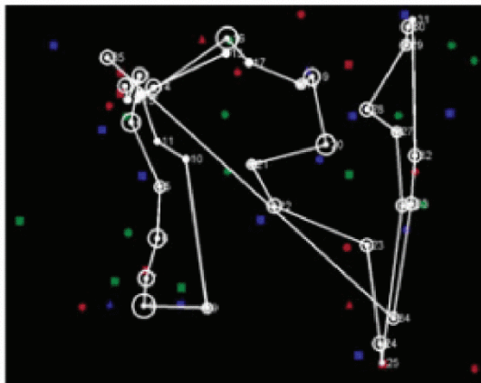
Figure 22 : Scanpaths pendant une tâche de recherche visuelle (visual search-task). Scanpath d'un patient de 72 ans avec HLH droite, à 8 jours de la lésion (phase aigue) (A). Scanpath du même patient à 18 mois de la lésion (phase chronique) (B). Le scanpath semble plus structuré en phase chronique qu'en phase aigue, avec une augmentation de la taille des saccades, une stratégie de recherche plus organisée en colonne, mais un même nombre de fixation. Scanpath d'un sujet contrôle de 65 ans (C). Figure tirée de Machner et al. (2009).
