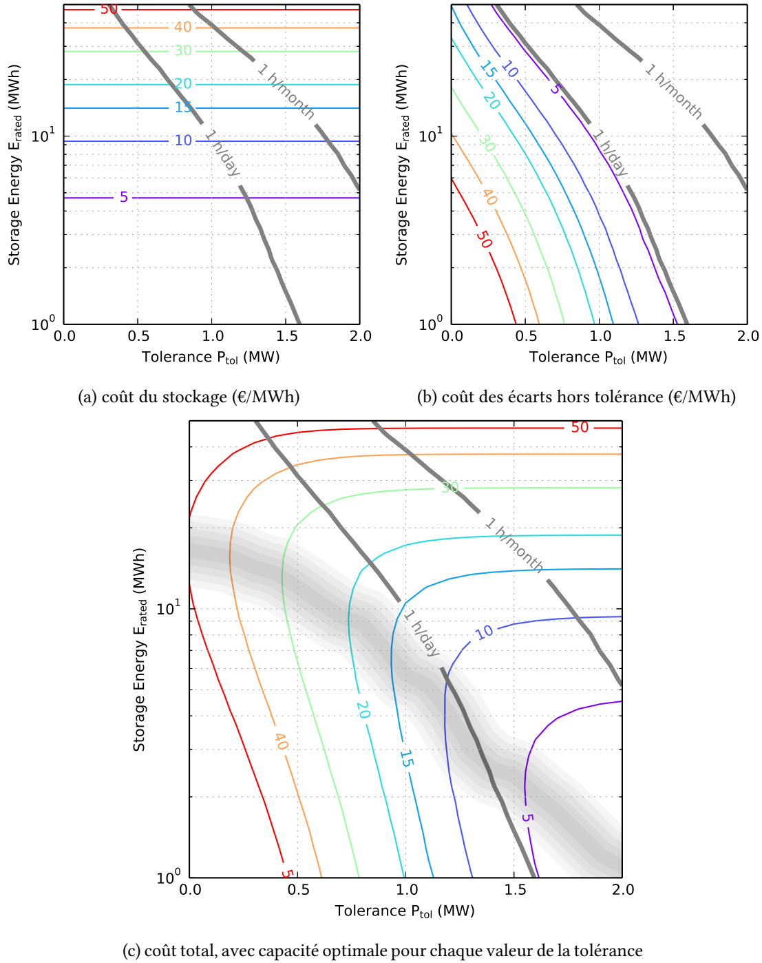
FIGURE 4.8 – Cartographie des coûts du système pour la garantie d'un engagement de production J+1 avec tolérance d'écart, fonction de la capacité de stockage et de la puissance d'écart toléré. Les coûts sont exprimés en "€/MWh d'énergie produite", d'après un calcul sur une durée t_{life} = 15 ans, avec hypothèse d'un facteur de charge de 20 % ( \bar{P}_{prod} = 2 MW). Coût du stockage c_{batt} = 280 k€/MWh et coût des écarts c_{dev} = 100 €/MWh.
