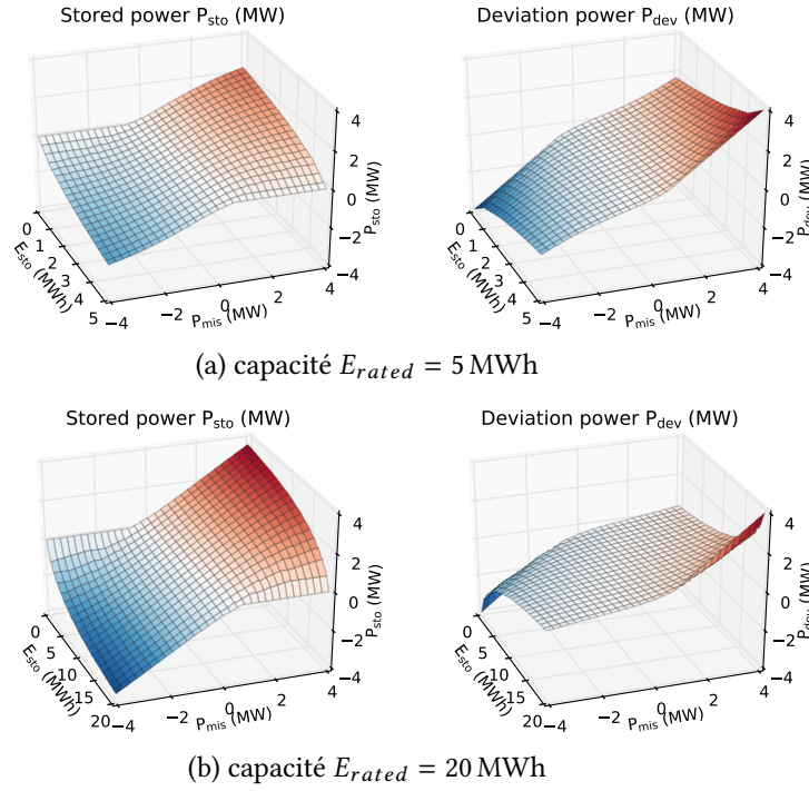
FIGURE 3.10 – Effet de la capacité sur la gestion optimale pour une pénalité quadratique (coefficient de corrélation \phi fixé à 0,8)
