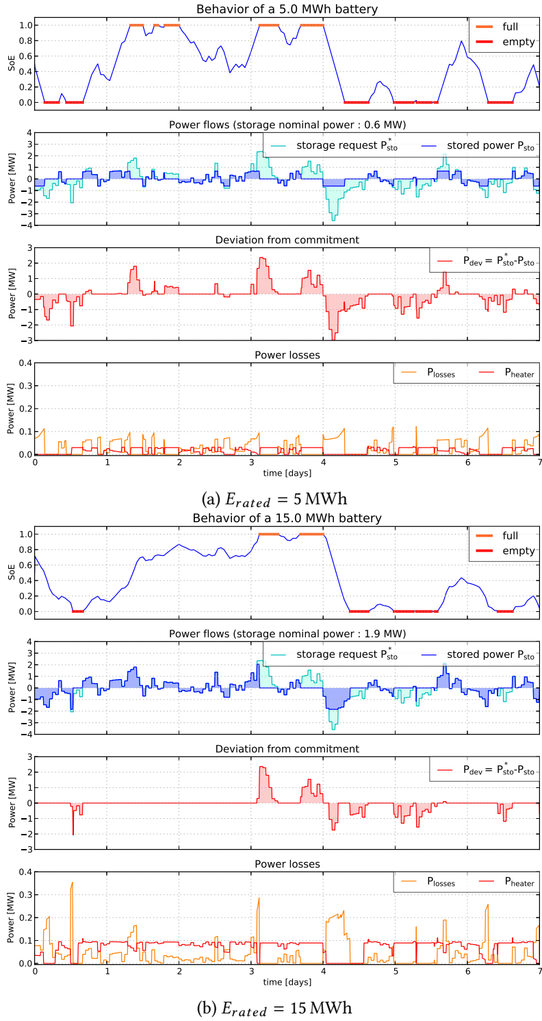
FIGURE 4.4 – Simulation stochastique avec le modèle de batterie NaS, la sollicitation d'entrée AR(1) d'écart-type \sigma_P = 1 \text{ MW} et \phi = 0,8 et loi de gestion empirique " P_{sto} = P_{mis} " [53].
