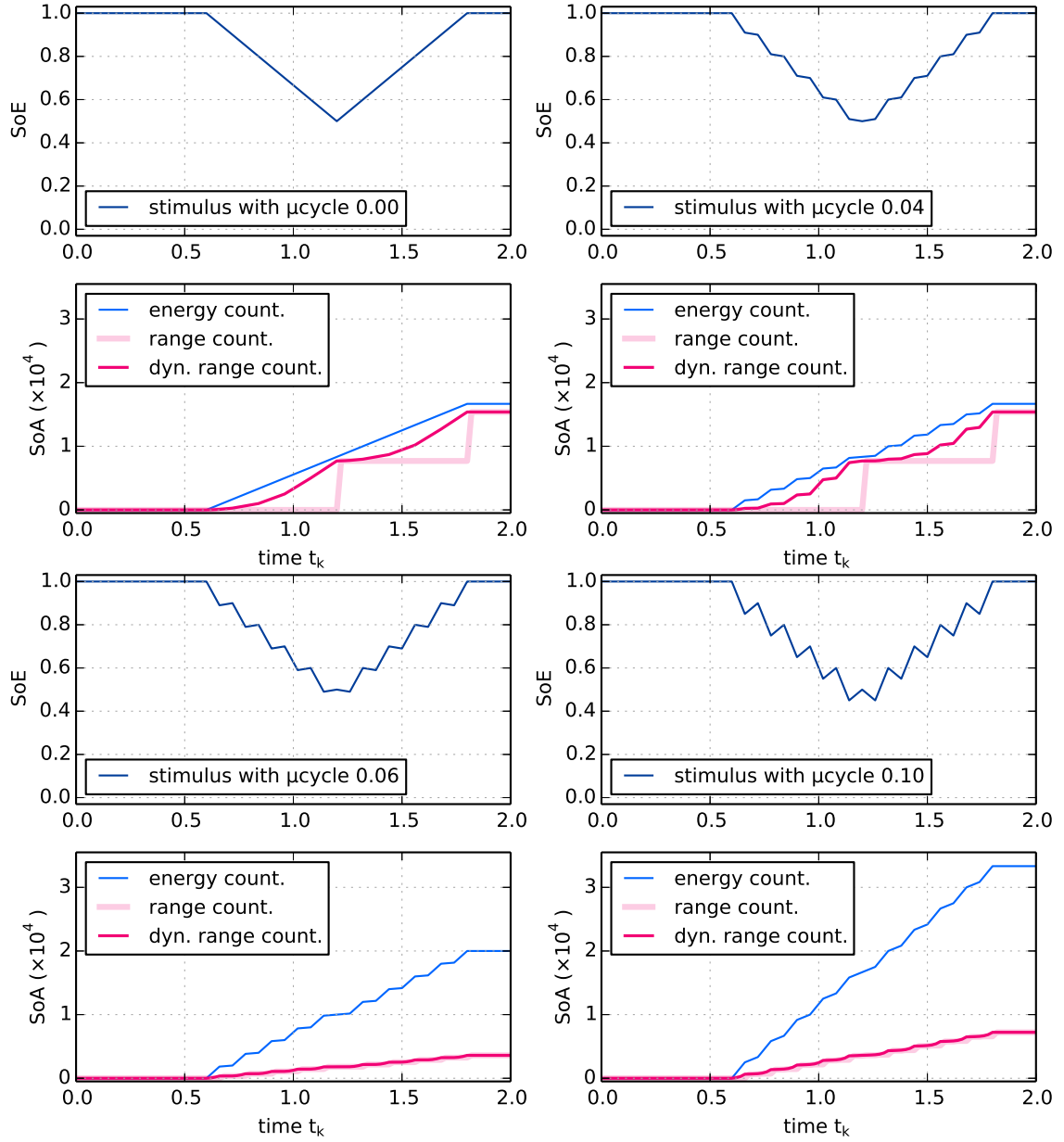
FIGURE 2.14 – Effets des micro-cycles sur le comptage : à un cycle de décharge de profondeur 0.50 sont superposés 10 micro-cycles de profondeur 0, 0.04, 0.06 et 0.10. EN HAUT : pour les profondeurs < 0.05 , le grand cycle n'est pas interrompu et donc la valeur finale du vieillissement est inchangée. EN BAS : pour les profondeurs > 0.05 , le grand cycle est interrompu, ce qui le masque aux yeux de l'algorithme Range Counting. Le vieillissement final est alors diminué ! À l'inverse, le comptage d'énergie est cohérent : les micro-cycles augmentent le vieillissement.
