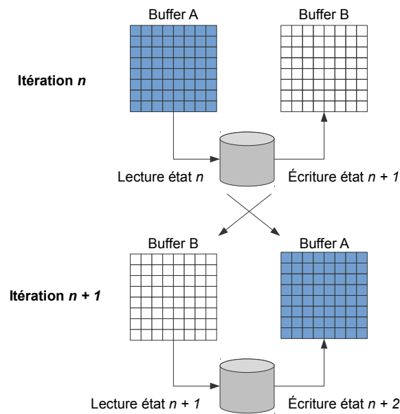
FIGURE 3.3 – Concepts de double buffering des données entre itérations
