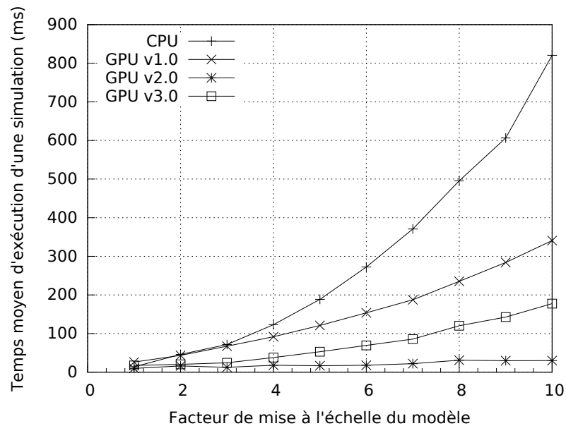
FIGURE 8.13 – Performances CPU et GPU MIOR sur carte Kepler K20m
