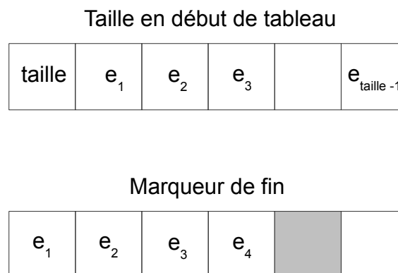
FIGURE 7.3 – Représentations de vecteurs proposées par MCMAS
