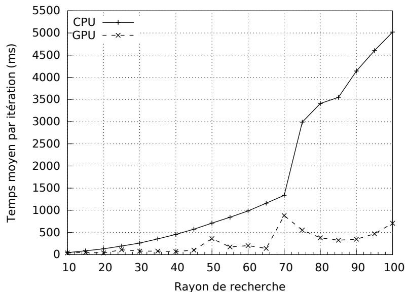
FIGURE 8.9 – Temps moyen d’exécution d’une itération du modèle proie-prédateur sur carte Radeon HD6870 et processeur AMD Phenom II X6 1090T
