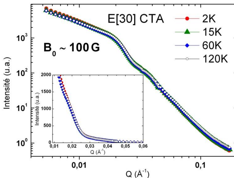
Figure 10-33 – Spectres de diffusion aux petits angles mesurés sous un champ magnétique proche de 100G et pour différentes températures dans la gamme [2K – 120K] pour E[30](b) CTA.
