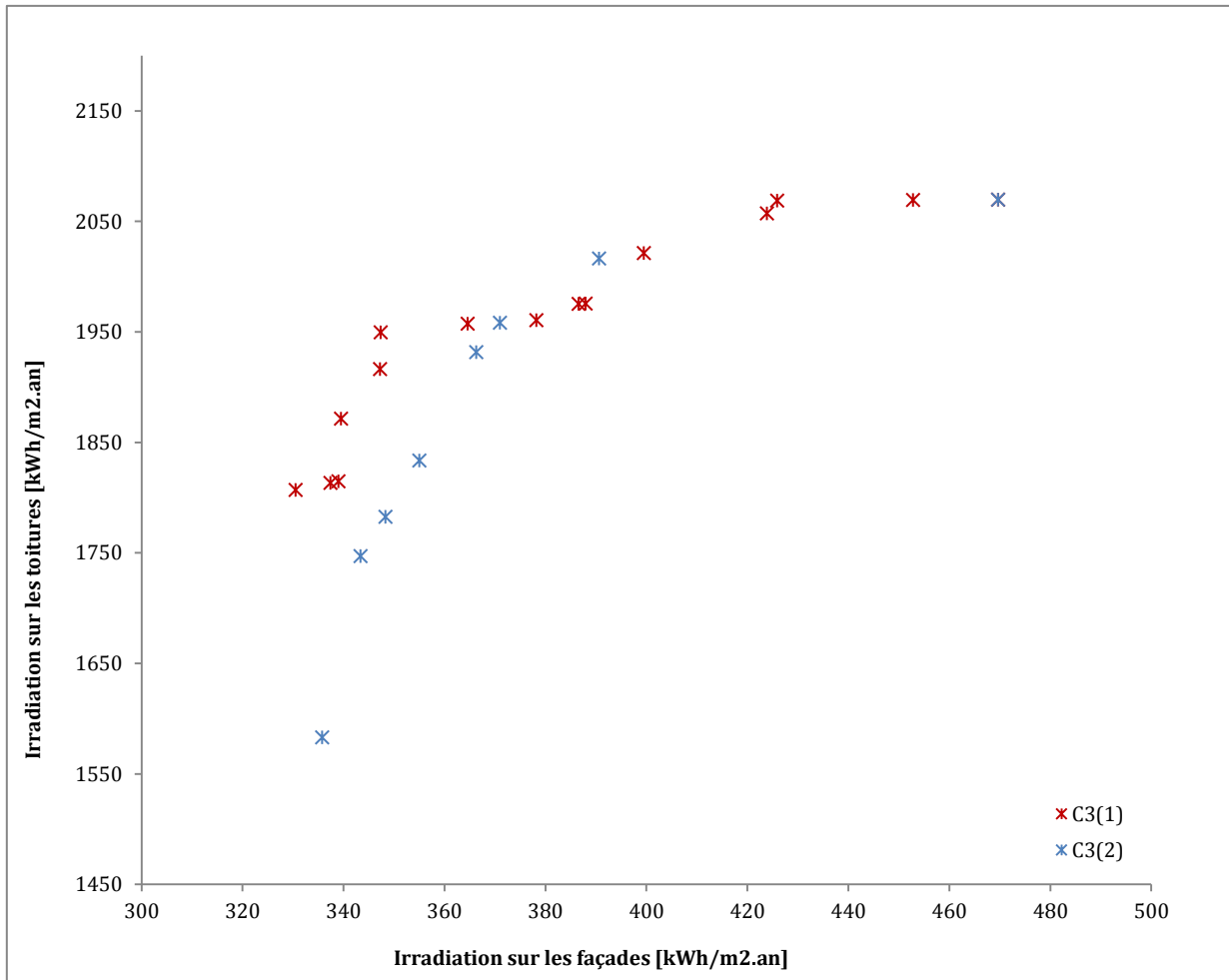
Figure 25: projets des fronts de Pareto pour les deux tours de simulations réalisés pour la classe 3.
