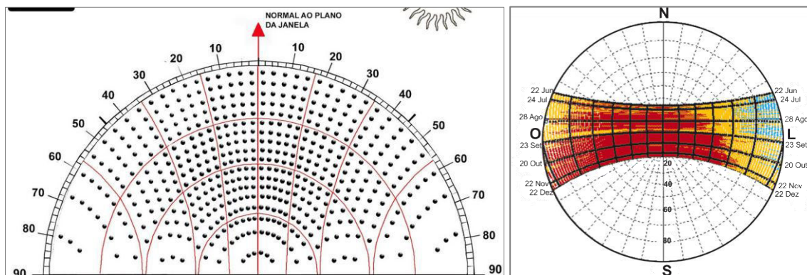
Figura 47: Diagrama de Pleyel com dados de iluminância externa e diagrama solar com sobreposição de dados de temperatura do ar externa para Maceió. Fonte: LABEEE, UFSC (2013).
