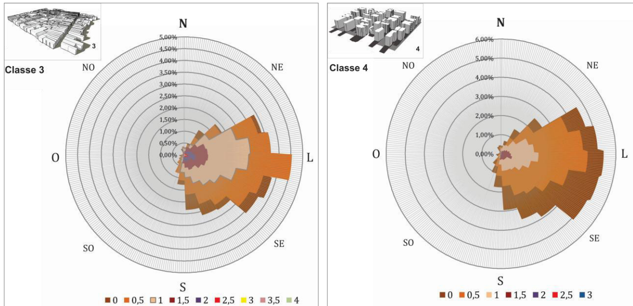
Figura 115: velocidade do vento corrigida para classe de rugosidade 3 e 4.
