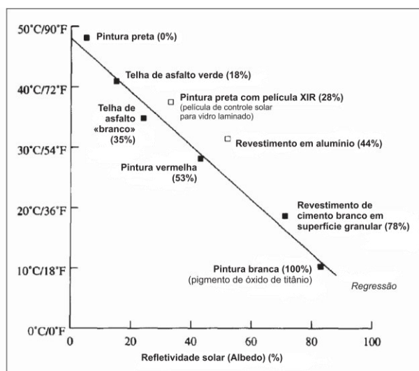
Figura 36: diferença entre a temperatura da superfície e do ar, em função do albedo de diferentes revestimentos. Fonte: adaptado de Rosenfeld et al. (1995).
