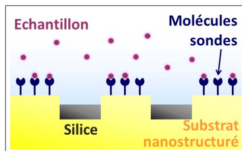
FIGURE 10.11 – Principe de la localisation des molécules sondes et cibles sur les nanocylindres. Un dépôt de silice permet de bloquer les parties d'or plat ne contribuant pas au signal SPR correspondant au mode localisé. L'utilisation d'une fonctionnalisation chimique orthogonale permet le greffage des molécules sondes sur les cylindres d'or disponibles.
