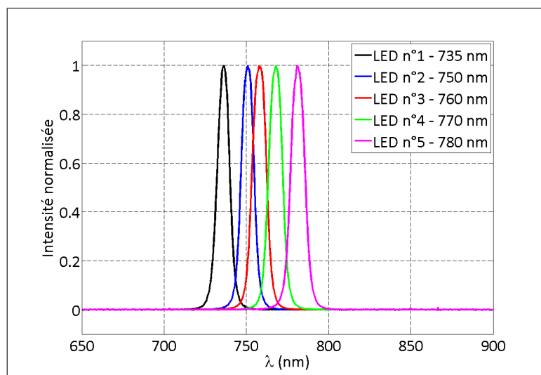
FIGURE 7.9 – Spectres d'émission des 5 LEDs en combinaison avec un filtre interférentiel. Les mesures présentées ont été effectuées à l'aide d'un spectromètre commercial (modèle USB2000+, Ocean Optics).
