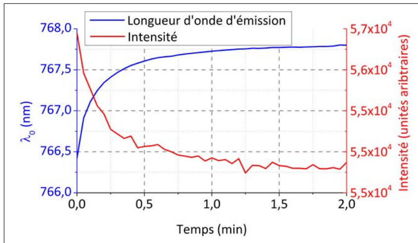
(b) Evolution des propriétés d'émission de la LED n°4 (770 nm) à long terme après commutation "on".
