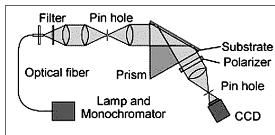
FIGURE 3.4 – Montage d'interrogation spectrale utilisant un monochromateur. Cette figure est tirée des résultats de Otsuki et Ishikawa [80].
