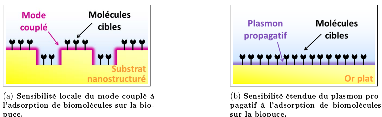
FIGURE 10.10 – Différence des surfaces sondées par le mode couplé, dans le cas d'une biopuce structurée, et du plasmon propagatif, dans le cas d'une biopuce conventionnelle.
