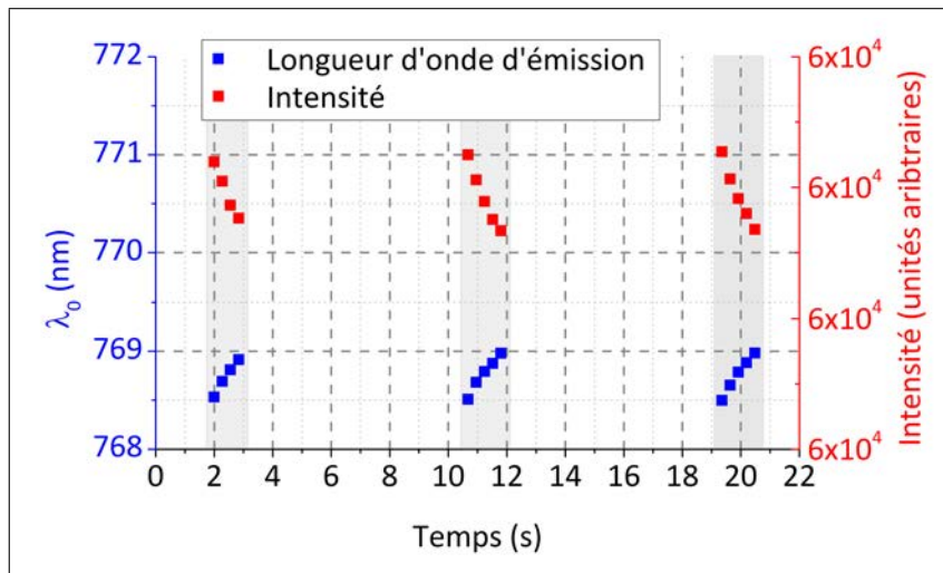
(a) Evolution des propriétés d'émission de la LED n°4 (770 nm) lors des sollicitations "on/off". Les mesures réalisées durant les commutations (représentées en zones grisées) mettent en évidence une augmentation de la longueur d'onde émise (en bleu), parallèlement à une diminution de l'intensité (en rouge).
