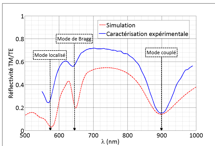
FIGURE 10.6 – Profil spectral de résonance pour un angle d'incidence de 71.1^\circ sur un prisme de verre BK7. Une épaisseur de 30 nm commune au film d'or et aux cylindres, un diamètre de 80 nm et une période de 200 nm ont été considérés lors des simulations et de la fabrication de la biopuce. Les résultats théoriques et expérimentaux ont été obtenus respectivement par Mitradeep Sarkar et Aurore Olivéro, doctorants au Laboratoire Charles Fabry.
