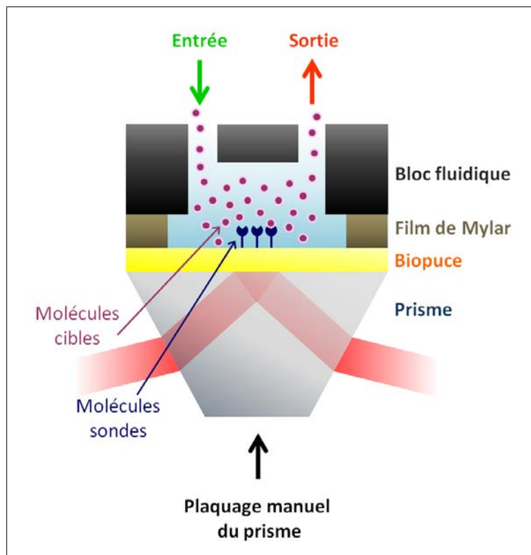
(c) Schéma du système de fluïdique utilisant un film de Mylar. Dans cette représentation de la cellule fluïdique vue en section, un bloc en titane, équipé de trous d'entrée et de sortie du flux, est recouvert par un film de Mylar présentant une découpe circulaire formant la cellule fluïdique.
