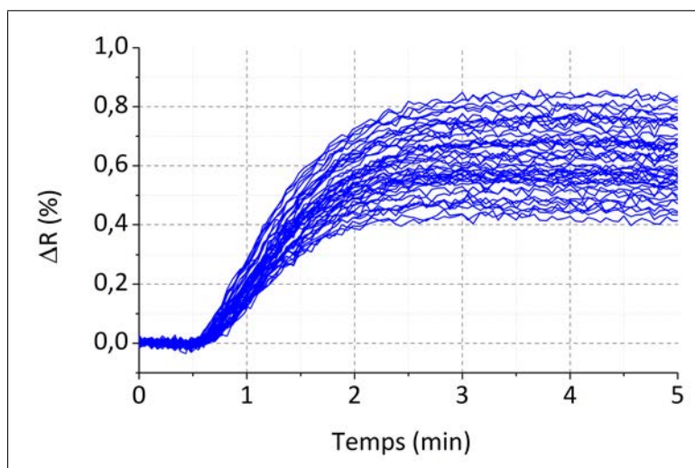
FIGURE 2.3 – Dispersion des données en interrogation en réflectivité. L'inhomogénéité de la surface analysée conduit naturellement à une dispersion des conditions de résonance plasmon. De ce fait, le choix d'un point de fonctionnement unique résulte en une dispersion des sensibilité aux différentes régions d'intérêt de la biopuce, et donc à une dispersion des données en termes de variation de réflectivité.
