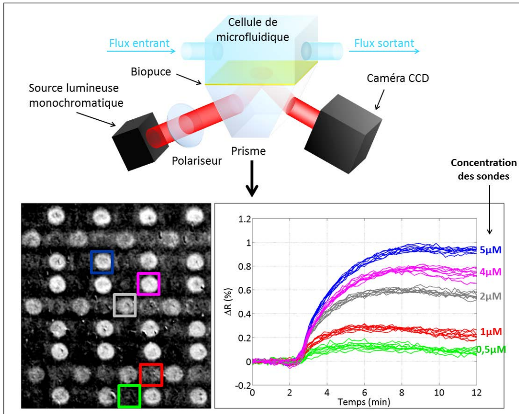
FIGURE 2.2 – Illustration des propriétés de mesure offertes par l'interrogation en réflectivité. Un montage classique de l'interrogation en réflectivité (présenté en haut de cette image) est basé sur une configuration de Kretschmann, avec une illumination monochromatique. L'angle d'incidence est fixé par la position angulaire de la pente maximale du profil de résonance plasmon. La mesure des variations de réflectivité est alors réalisée en polarisation TM, par un détecteur à deux dimensions en sortie du montage. Le suivi des interactions biomoléculaires peut ainsi être réalisé en temps réel (figure en bas à droite), et ce pour toute la surface de la biopuce imagée (représentée en bas à gauche).
