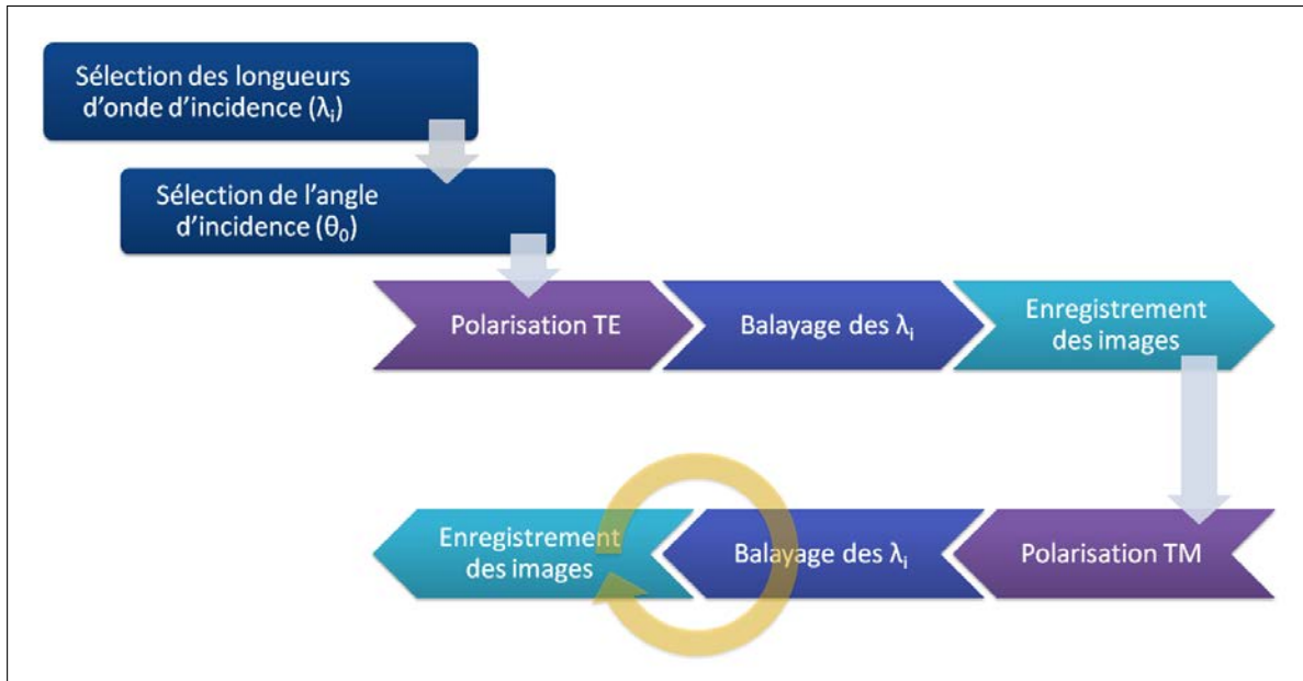
FIGURE 4.4 – Principe de fonctionnement de l'interrogation spectrale en mode cinétique. Après sélection des paramètres expérimentaux (angle et longueurs d'onde d'incidence), le système acquiert une première série d'images en polarisation TE. Le polariseur se place alors en polarisation TM et le monochromateur entame un balayage cyclique des longueurs d'onde d'excitation choisies. Pour chaque cycle de mesure et chaque longueur d'onde, l'image en réflexion de la biopuce est enregistrée par la caméra sur le disque dur.
