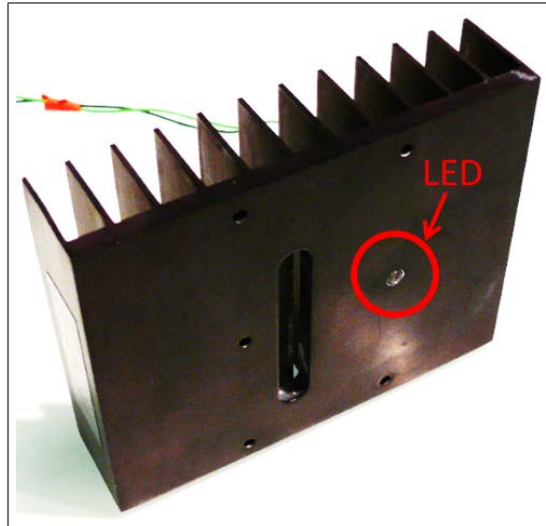
FIGURE 8.3 – Photographie du dispositif testé pour améliorer la stabilité thermique des LEDs à l'allumage. Un trou d'un diamètre de 5 mm a été percé dans un radiateur en aluminium, permettant d'insérer une LED enduite de pâte thermique pour favoriser la dissipation de la chaleur émise lors de l'allumage.
