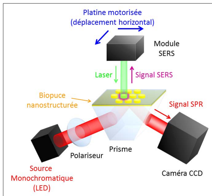
FIGURE 10.1 – Principe simplifié de l'instrument bimodal combinant une mesure SERS et SPR. Dans la configuration instrumentale envisagée, la partie inférieure du montage est consacrée à la mesure SPR. Dans la configuration de Kretschmann, une biopuce, placée sur un prisme, est illuminée par une source monochromatique (LED). Le signal est recueilli en temps réel et sur toute la surface analysée par une caméra CCD. La partie supérieure du prototype, constituée du module SERS, est exploitée après détection spécifique par SPR : le point de focalisation du laser excitateur est déplacé dans le plan de la biopuce jusqu'aux plots sondes d'intérêt. La mesure Raman permet alors l'identification précise des espèces cibles adsorbées.
