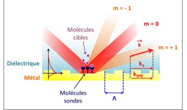
(b) Principe de l'excitation plasmonique basée sur l'utilisation d'un réseau. Dans cette configuration, la structuration de la biopuce en réseau de période \Lambda adaptée induit une diffraction du faisceau incident. De cette manière, l'indice effectif du premier ordre diffracté permet de satisfaire l'égalité avec le vecteur d'onde plasmon et atteindre la résonance.
