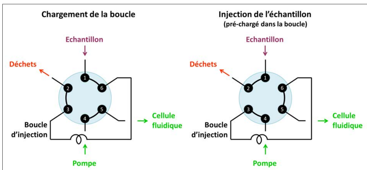
FIGURE 4.3 – Principe de fonctionnement de la vanne d'injection utilisée dans le montage expérimental. Un système de basculement entre les différentes entrées et sorties du flux permet l'injection des échantillons dans la cellule fluide. Dans une première position, dite de "chargement de la boucle", la solution à analyser est pré-chargée dans une boucle de 200 \mu\text{L} . Le surplus est automatiquement dirigé vers la sortie "déchets" : cette étape est décorrélée de la circulation du système fluide. Une seconde position "d'injection" est obtenue par basculement de la vanne : le milieu circulant dans le système, pompé par la pompe péristaltique, rentre alors dans la boucle et pousse l'échantillon pré-chargé vers la cellule fluide.
