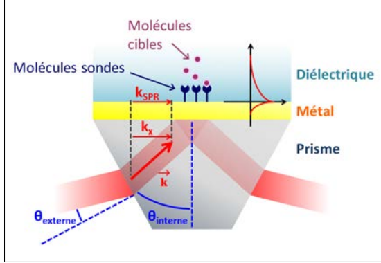
(a) Principe de l'excitation plasmonique basée sur l'utilisation d'un prisme. Dans cette configuration, la condition de résonance plasmon est satisfaite en augmentant l'indice du milieu incident par l'illumination de la biopuce à travers un prisme.
