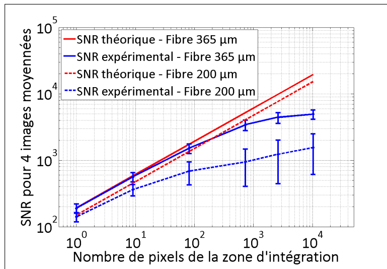
FIGURE 4.14 – Evolution du rapport signal à bruit en fonction de la moyennes spatiale pour deux fibres optiques de 365 \mu\text{m} et 200 \mu\text{m} de coeur. Ces données ont été obtenues pour une moyenne temporelle de 4 images.
