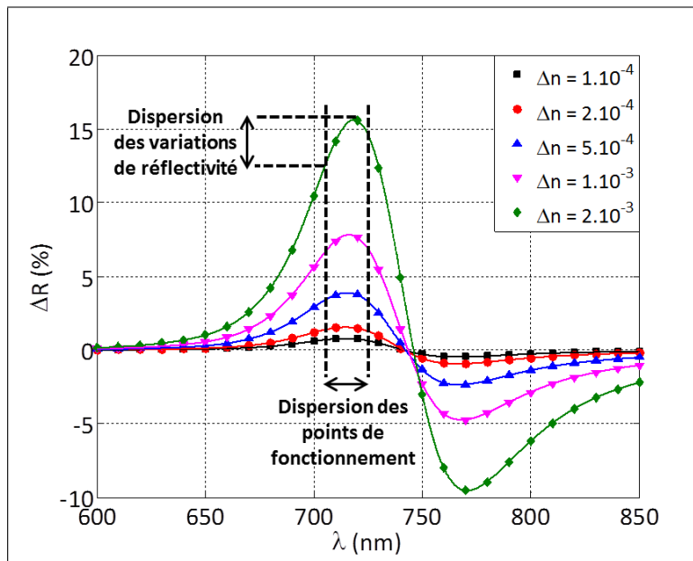
FIGURE 5.3 – Simulation des variations de réflectivité en réponses aux sauts d'indice réalisés expérimentalement.
