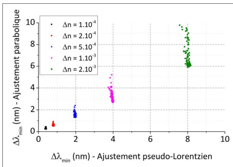
FIGURE 4.7 – Comparaison de la qualité de l’ajustement parabolique et pseudo-Lorentzien. Des données expérimentales correspondant à des injections de solutions d’indice croissant à la surface d’une lame d’or nu ont été traitées par les méthodes d’ajustement parabolique (présenté sur l’axe des ordonnées) et pseudo-Lorentzien (correspondant à l’axe des abscisses) pour déterminer le décalage spectral \Delta\lambda_{min} du minimum de réflectivité. Pour chaque saut d’indice étudié, le signal a été extrait sur 100 zones de 41 \times 41 pixels à la surface de la biopuce. La configuration d’interrogation spectrale adoptée est basée sur 5 longueurs d’onde espacées de 20 nm.
