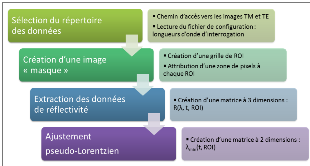
FIGURE A.1 – Principe du code d'extraction des données enregistrées en interrogation spectrale développé sous Matlab. Après lecture des paramètres d'acquisition dans le fichier de configuration, un masque est créé de manière à associer des zones de pixels (ROI) des images en réflectivité aux plots sondes. Une fois cette étape terminée, commence l'extraction des données, par la création d'une matrice à trois dimensions R(\lambda, t, ROI) contenant les valeurs de réflectivité TM/TE associées aux longueurs d'onde incidentes, aux plots sondes et aux temps de prise des images. Sur la base de ces résultats, un ajustement pseudo-Lorentzien est appliqué à chaque ensemble de valeurs de réflectivité discrètes correspondant à une ROI et un instant de mesure donnés. La matrice à deux dimensions ainsi créée, \lambda_{min}(t, ROI) , contient alors les valeurs des positions de la résonance plasmon, au cours du temps, pour chaque plot sonde de la biopuce.
