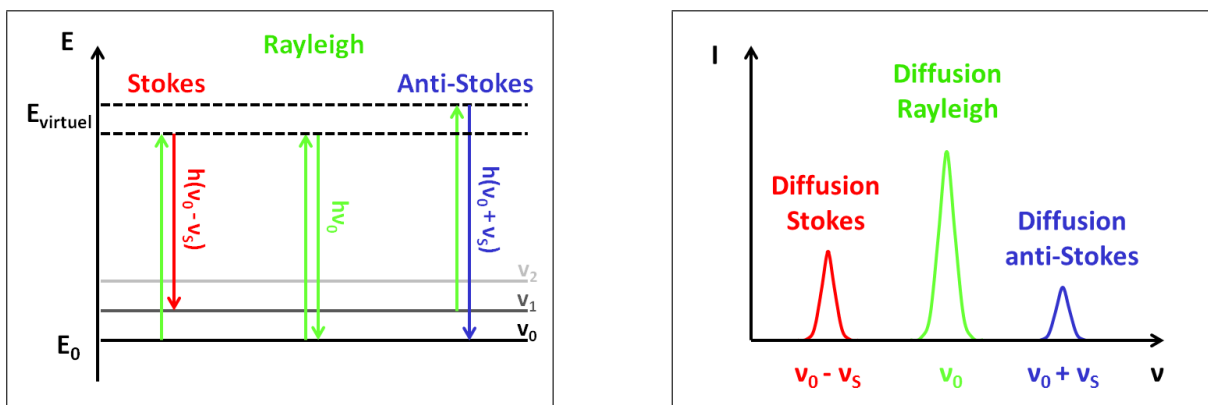
(a) Illustration de la diffusion Raman par un diagramme énergétique simplifié.
